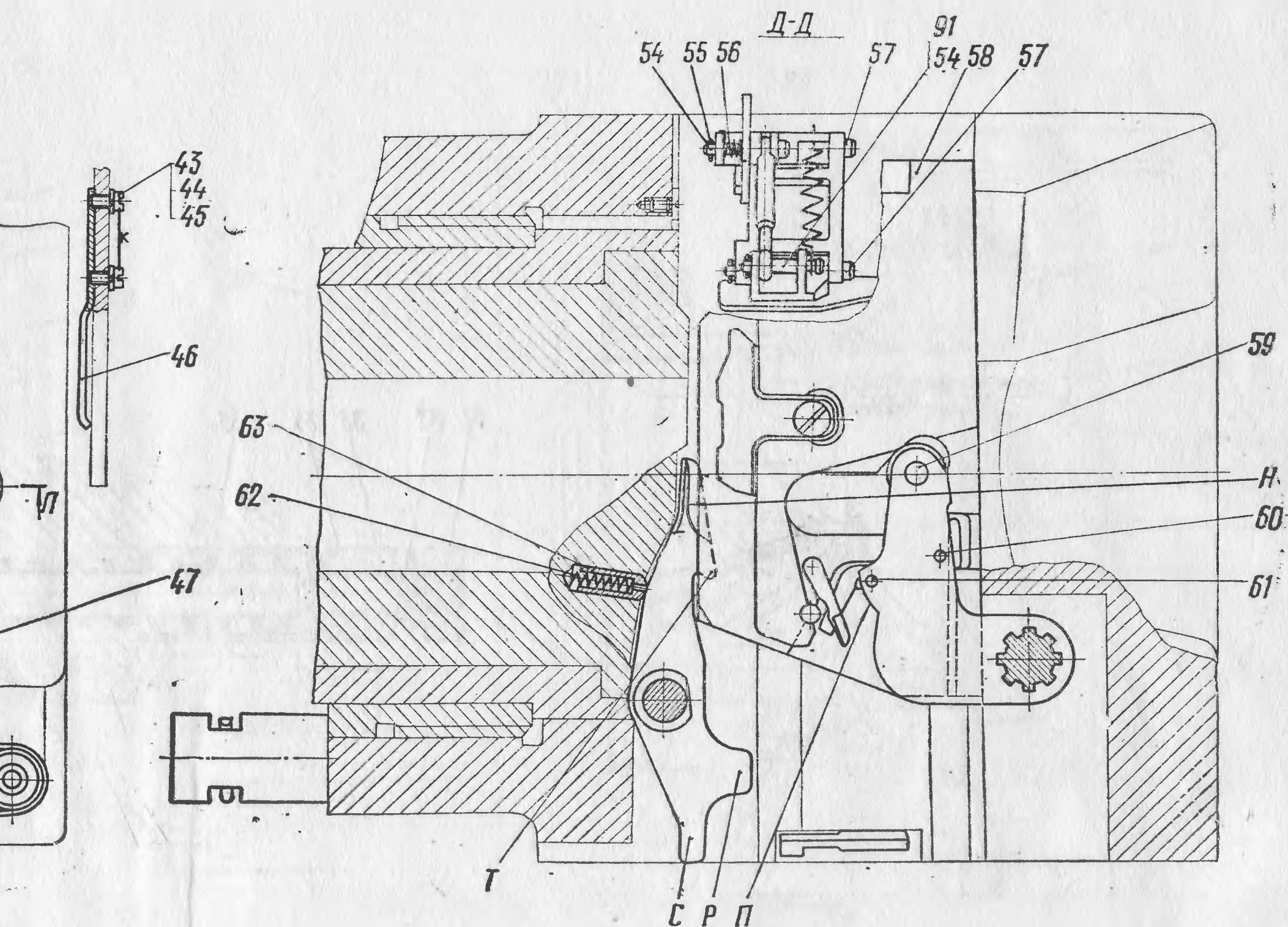
Рис. 8 (лист 2).
