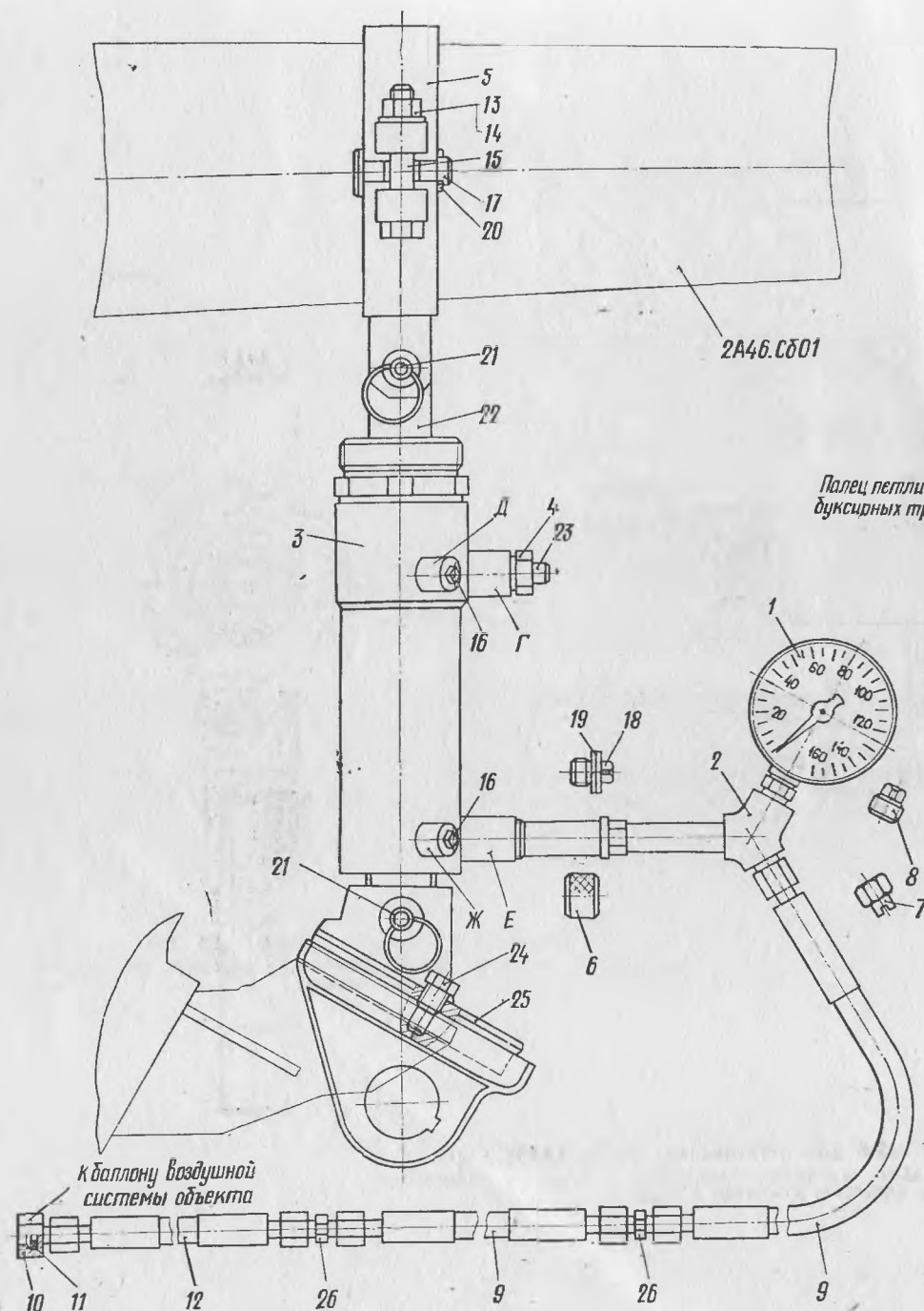
Крепление кронштейна на объекте сизделием 2А46-1
