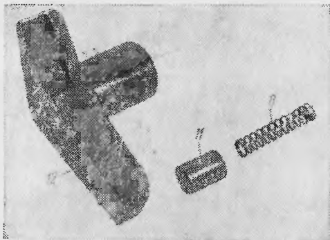
Рис. 13. Предохранительный механизм: 8 — пружина 2А20.02-35; 11 — колпачок 2А20.02-88; 12 — предохранитель спуска 2А20.02-4
