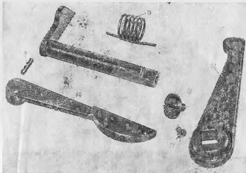
Рис. 14. Детали механизма повторного взведения: 3 — штифт 5u8x22; 4 — рычаг 2А26.10-122; 22 — ось повторного взвода 2А26.02-31; 23 — рычаг 2А26.02-116; 77 — винт В.М6-8g×10.6г.С 06 ГОСТ 17475-80; 78 — пружина повторного взвода 2А20.02-74; 79 — винт 52-ПТ-412С.02-103
