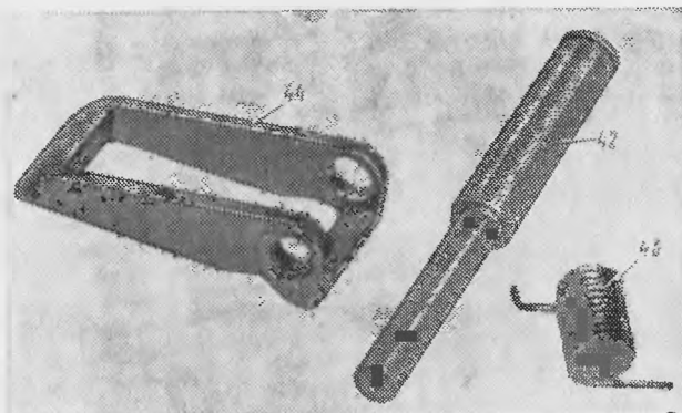
Рис. 17. Детали стопора лотка:
