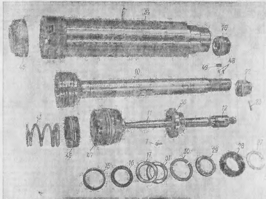
Рис. 26. Детали тормоза отката 2А46.С6 08:
