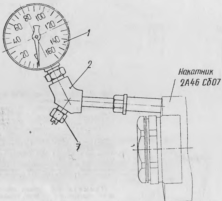
Рис. 50. Проверка давления в накатнике:
