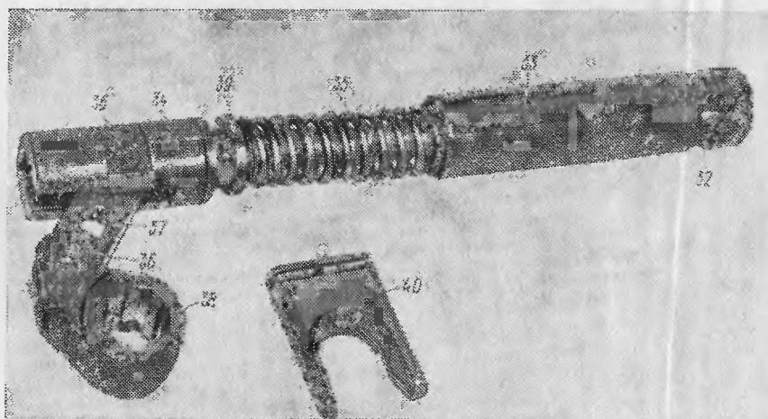
Рис. 15. Полуавтоматика: 32 — шплинт 4×45.06 ГОСТ 397-79; 33 — стакан 2А26. С6 02-19; 34 — шток полуавтоматики 2А26.02-12; 35 — пружина полуавтоматики 2А26.02-108; 36 — ось 2А26.02-106; 37 — серьга 2А26.02-110 или 2А26.02-110-1; 38 — кулачок полуавтоматики 2А26.02-109; 39 — втулка 2А26.02-107; 40 — скоба 2А26.02-114
