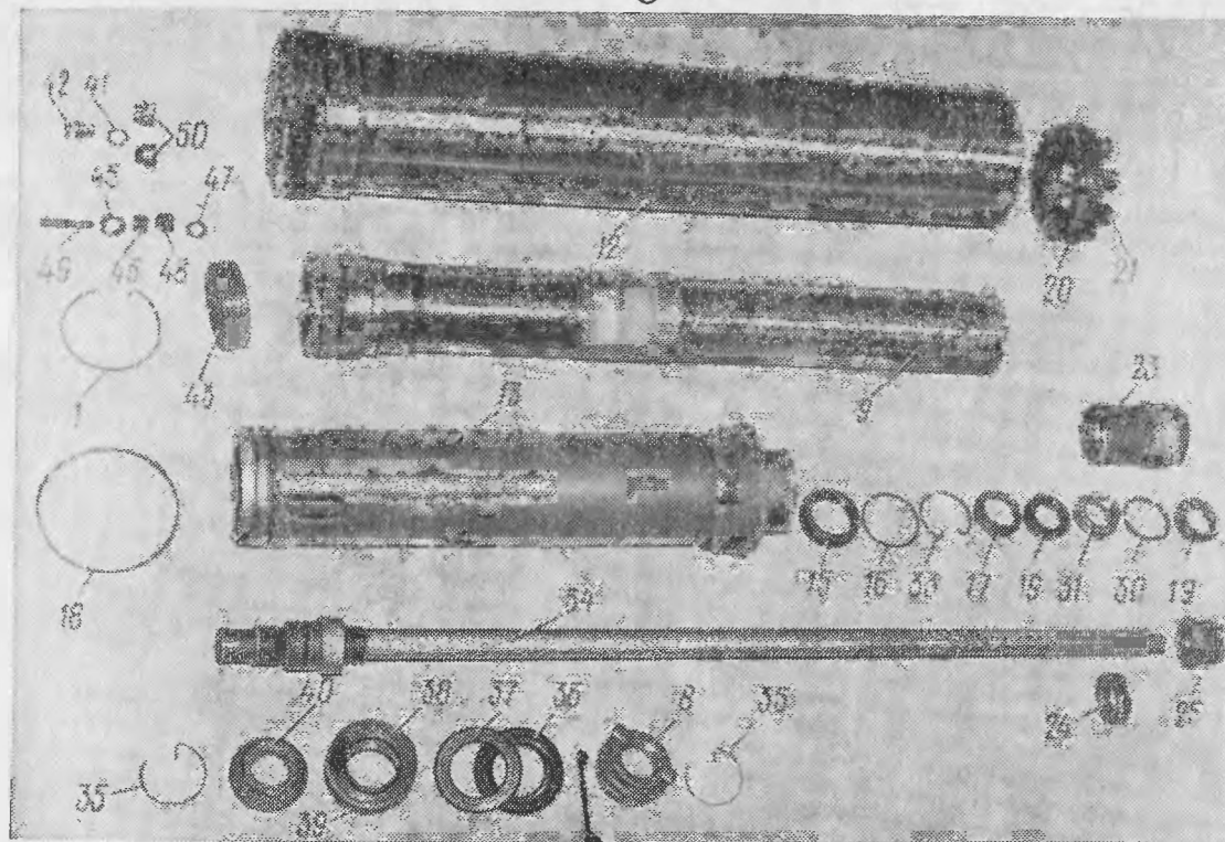
Рис. 29. Детали накатника:
