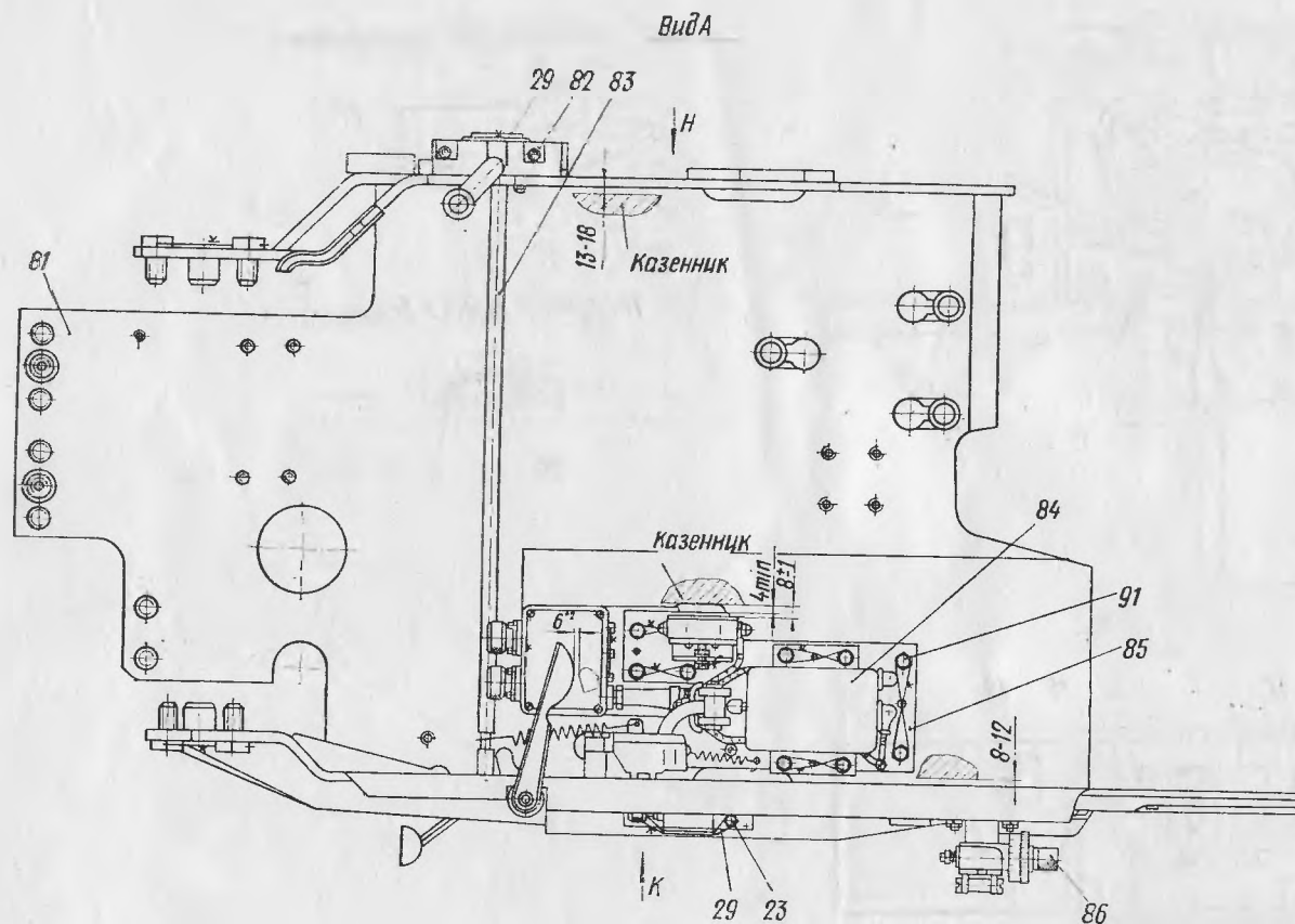
Рис. 35 (лист 3). Ограждение 2А46-1.С6 10:
