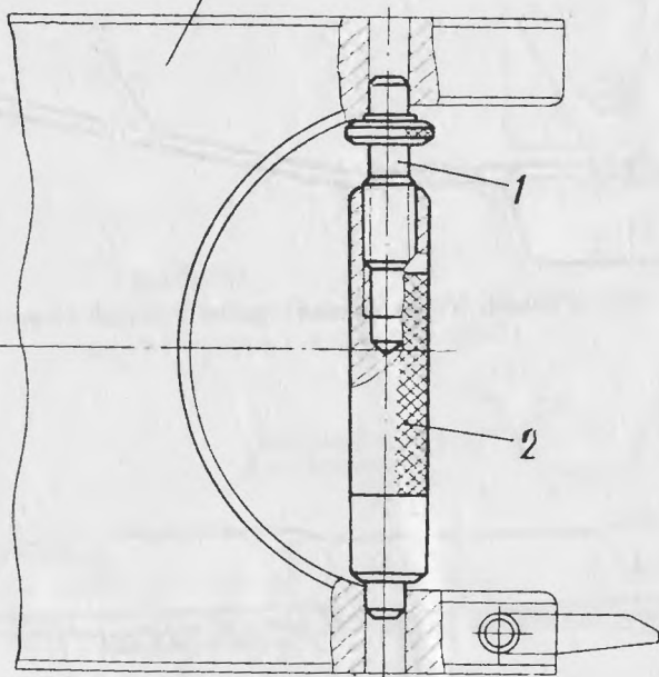
Рис. 57. Установка ручки 2А20.Сб 42-4 для вынимания клина:
