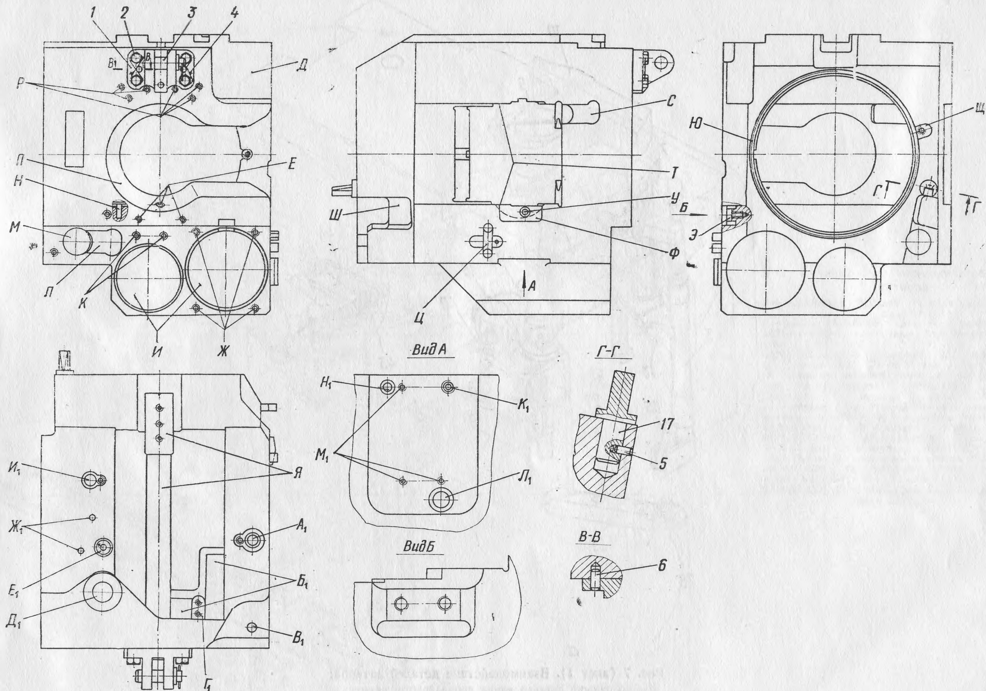
Рис. 6. Казенник:
