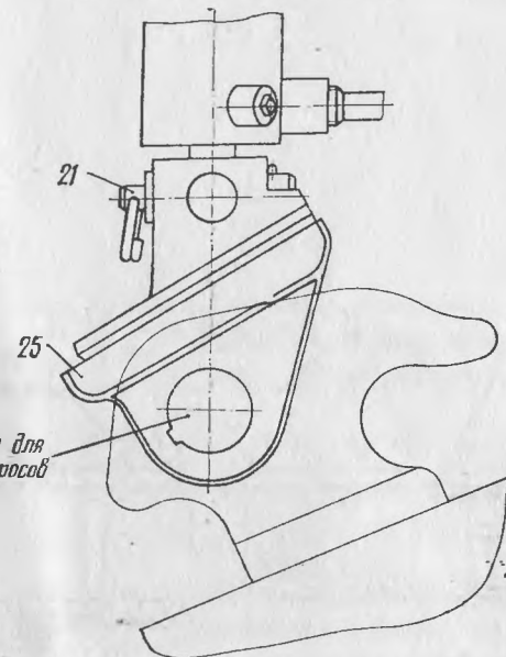
Крепление кронштейна на объекте сизделием 2А46-1
