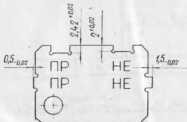
Рис. 58. Шаблон 2А26.42-21
