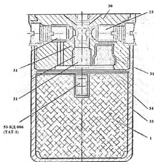
Рис. 14. Замедлительный и детонирующий узлы: 1- детонатор; 23- установочный винт; 31- пороховые цилиндрики; 33- стакан детонатора; 34- прокладка
