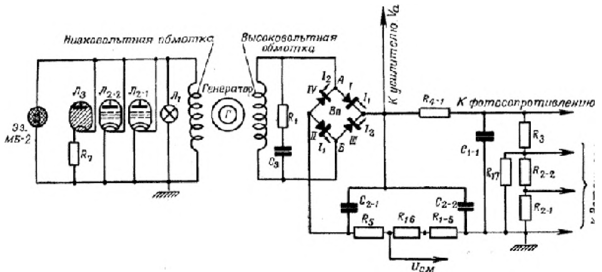
Рис.30 Схема питания взрывателя
