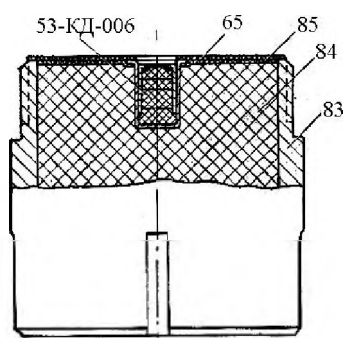
Рис.19. Детонирующее устройство: 65- прокладка; 83- стакан; 84- шашка; 85- кружок; 53- КД- 006- капсуль-детонатор ТАТ-1
