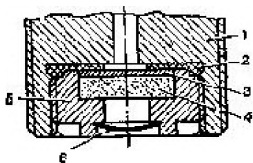
Рис. 22. Воспламенительное устройство взрывателя АТ-ЭБ: 1- хвостовик корпуса; 2- герметизирующее кольцо; 3- шелковая сетка; 4- воспламени тельная петарда; 5- донная втулка; 6- доньевая заделка
