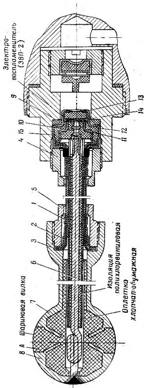
Рис.16 Электропиротехническое устройство:
