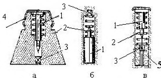
Рис. 3 Реакционные ударные механизмы
