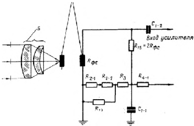
Рис.28. Приемник взрывателя (схема)
