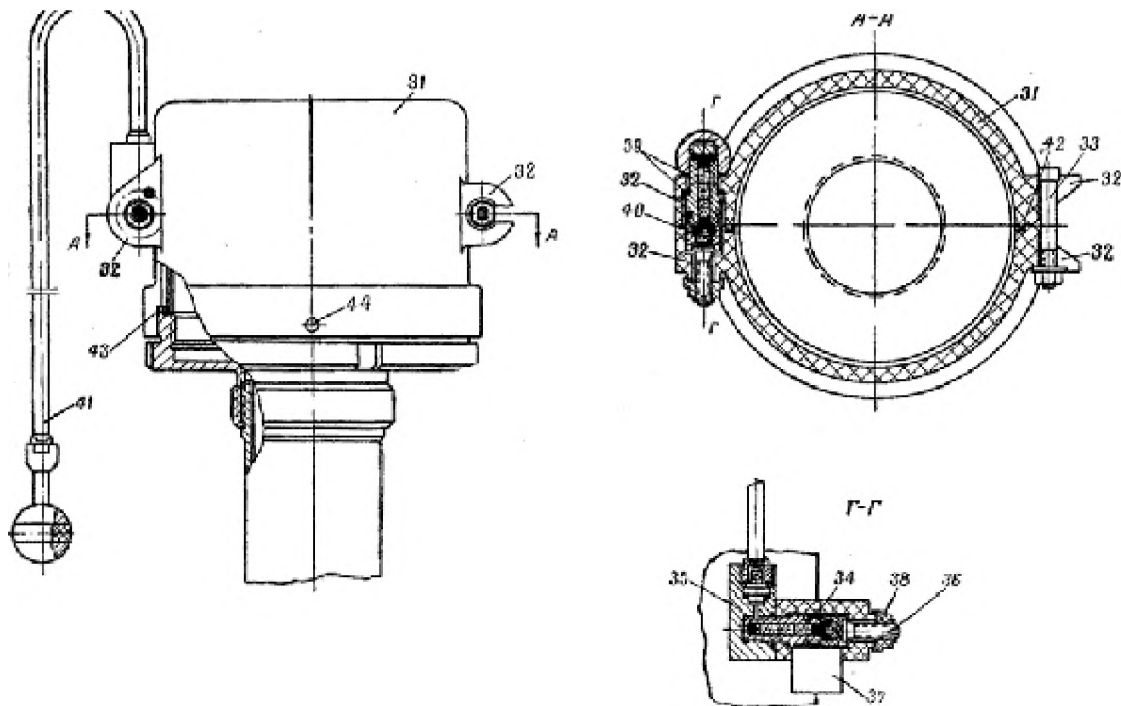
Рис.32 Защитное устройство взрывателя:
