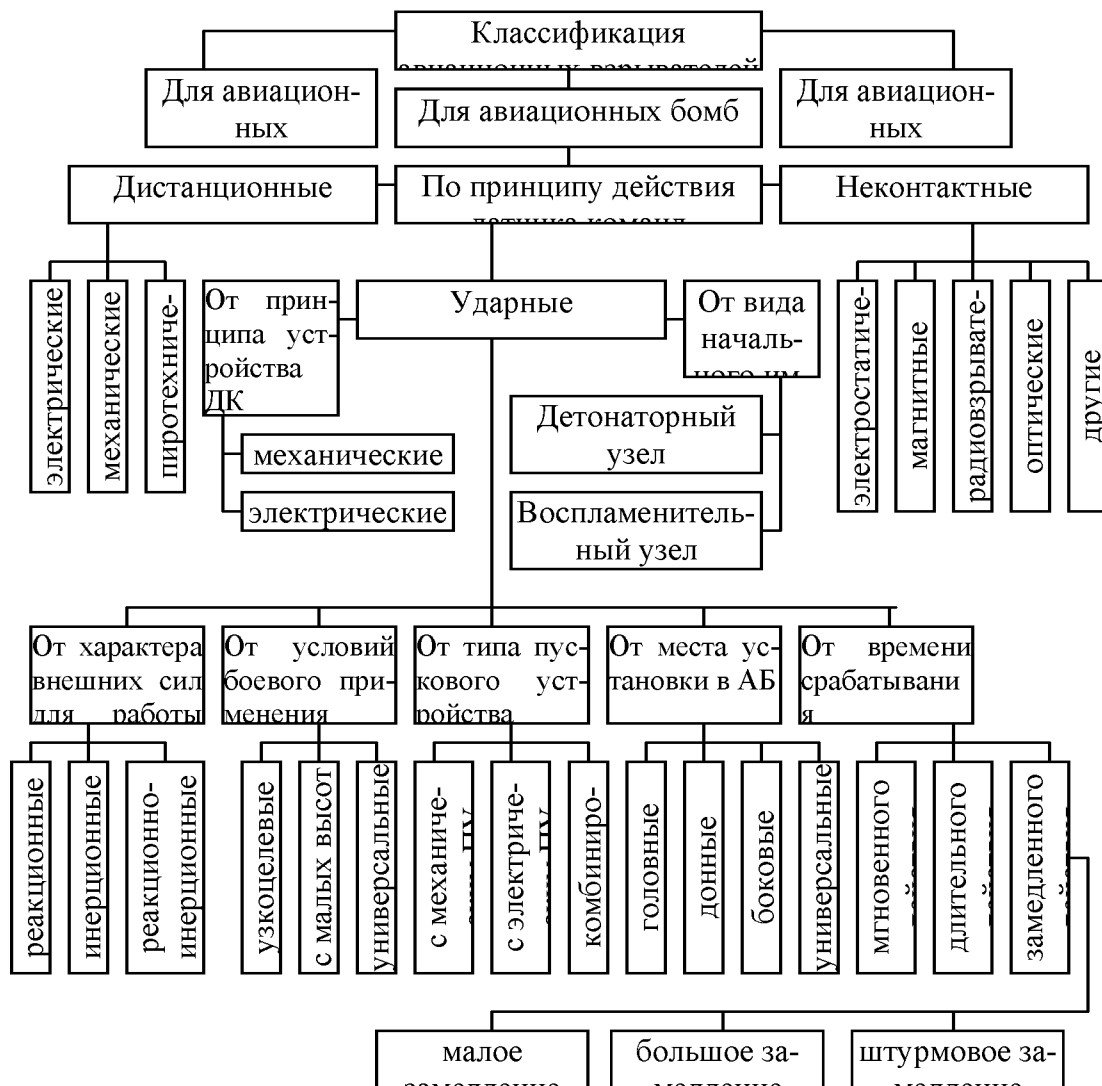
Рис.2. Классификация взрывателей
