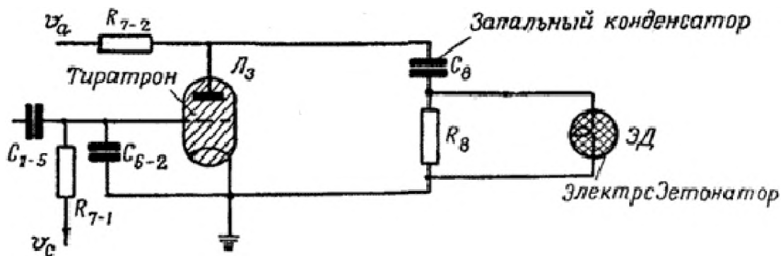
Рис.31 Исполнительный каскад взрывателя
