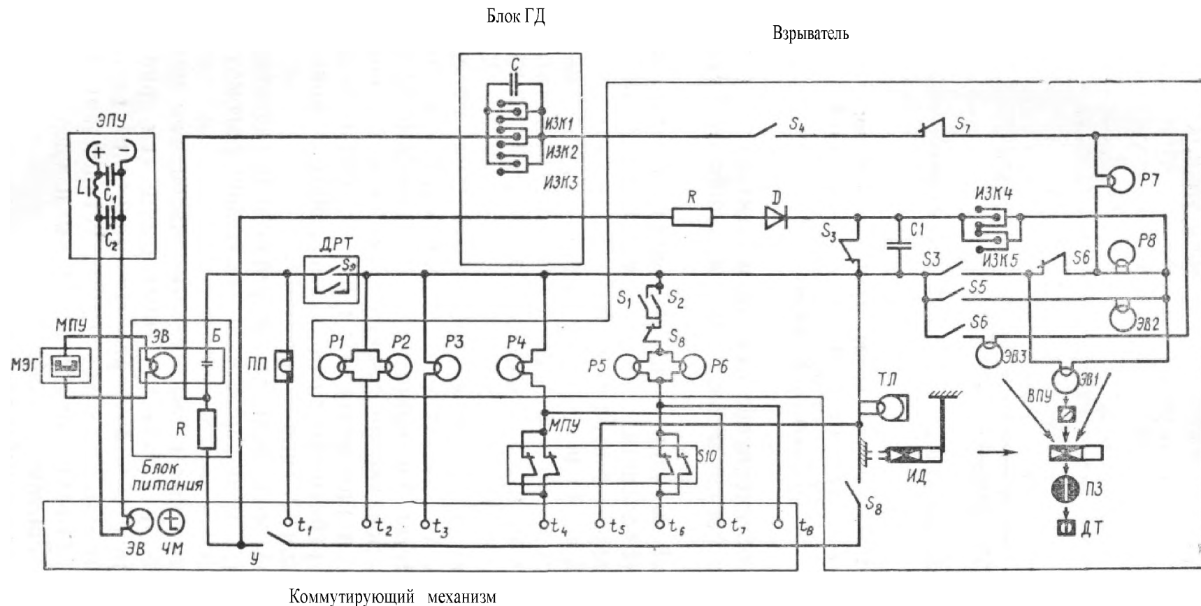
Рис. 35. Функциональная электрическая схема АВУ:
