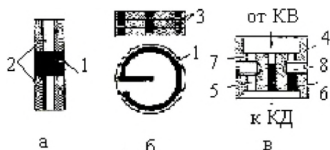
Рис.5 Замедлительное устройство:
