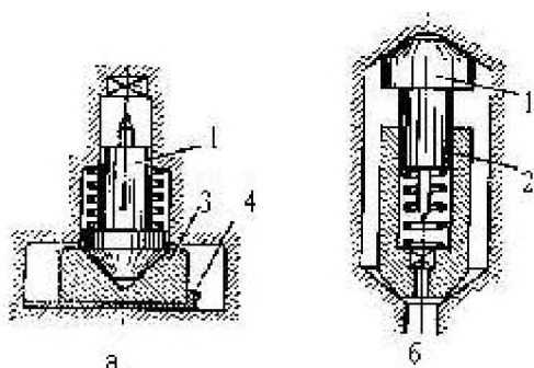
Рис.4 Бокобойные и всюдубойные ударные механизмы: а-бокобойный; б- всюдубойный; 1,2- инерционные ударники; 3- инерционная шайба; 4- жесткий предохранитель
