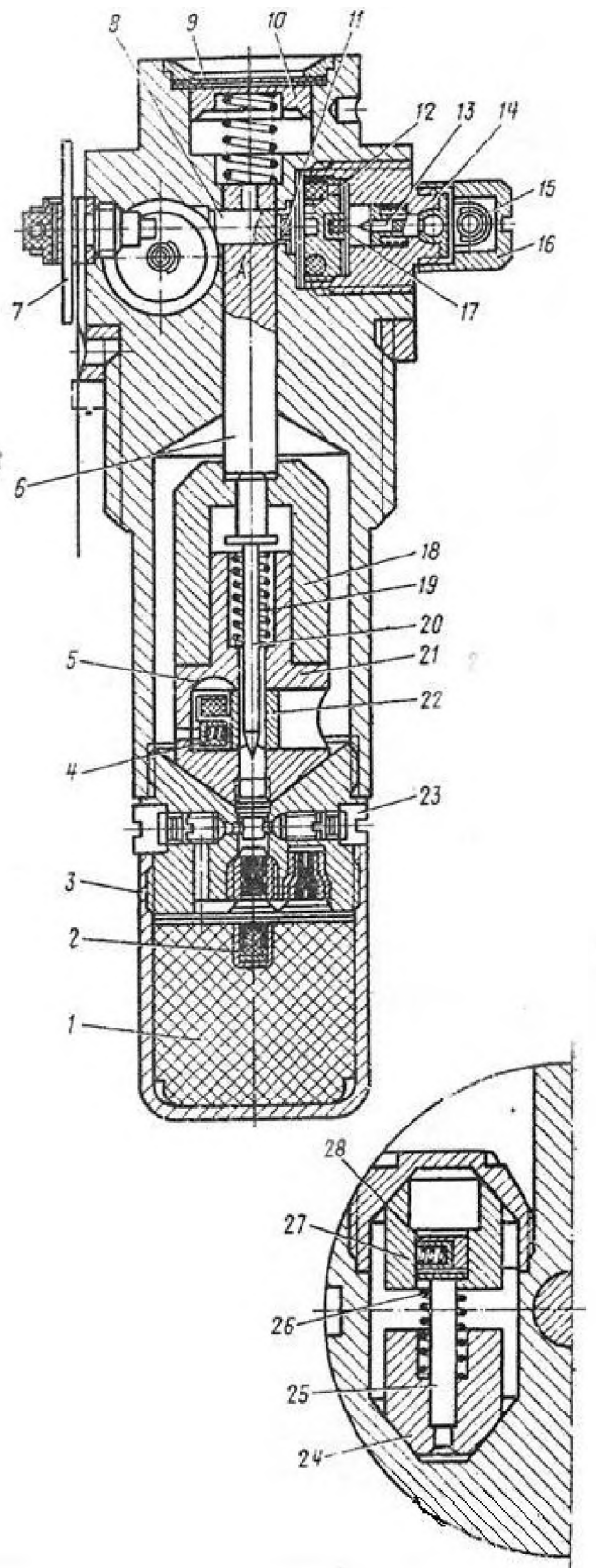
Рис. 10. Устройство взрывателя:
