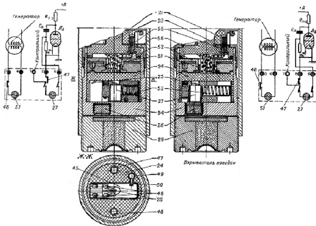
Рис.33 Запально- предохранительный механизм и элементы огневой цепочки. 21- колодка с контактами; 23- крышка; 24- колодка; 25- контактные пластины; 26- передаточный заряд; 27- электродетонатор; 29- стакан с детонатором из флегматизирующего ТЭНа; 45- движок; 46- контакты движка; 47- переключатель; 48- размыкатель; 49- стопор; 50- штифт; 51- кольцо; 52- грибок; 53- пружина; 54- корпус; 55- штепсели; 56- гайка; 57- электро-запал МБ-2Н.
