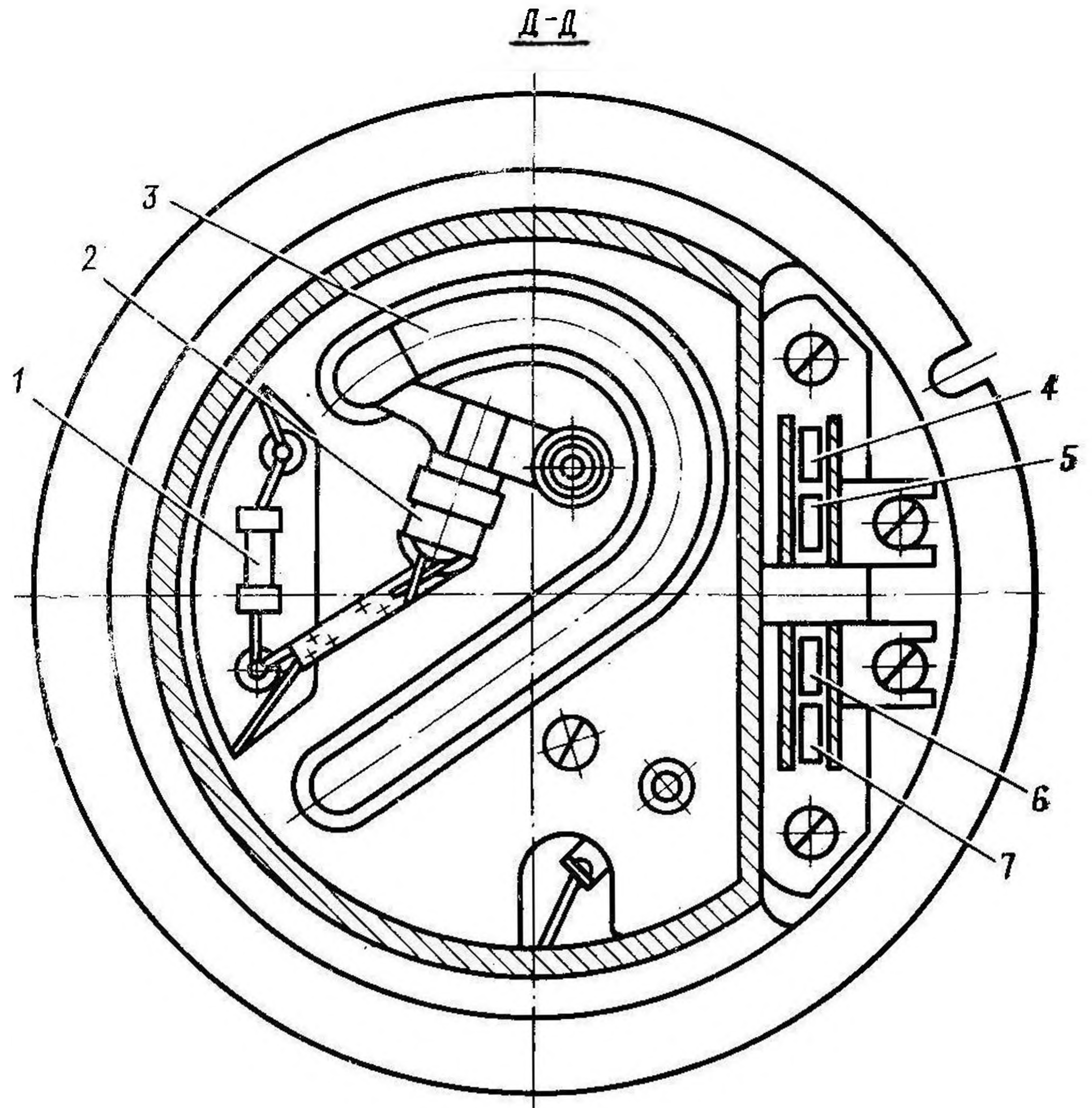
Рис. 18. Предохранительно-исполнительный механизм 9Э256:
