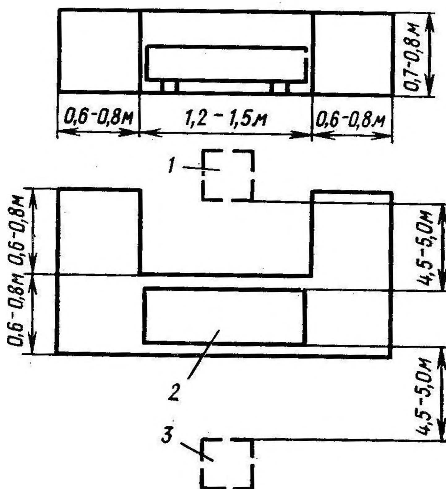
Рис. 39. Траншея для проверки выстрелов ЗУБК10 на функционирование:
