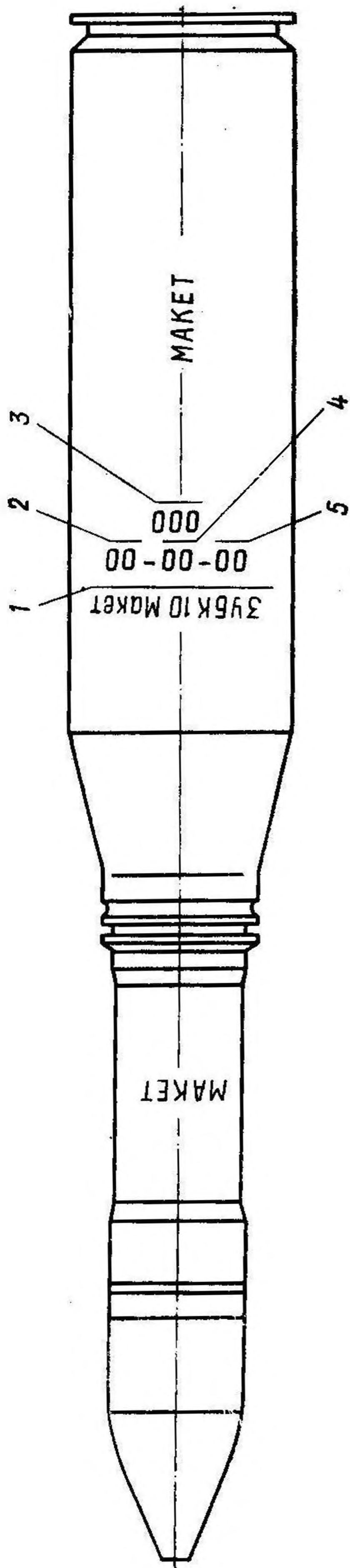
Рис. 35. Маркировка габаритно-весового макета:
