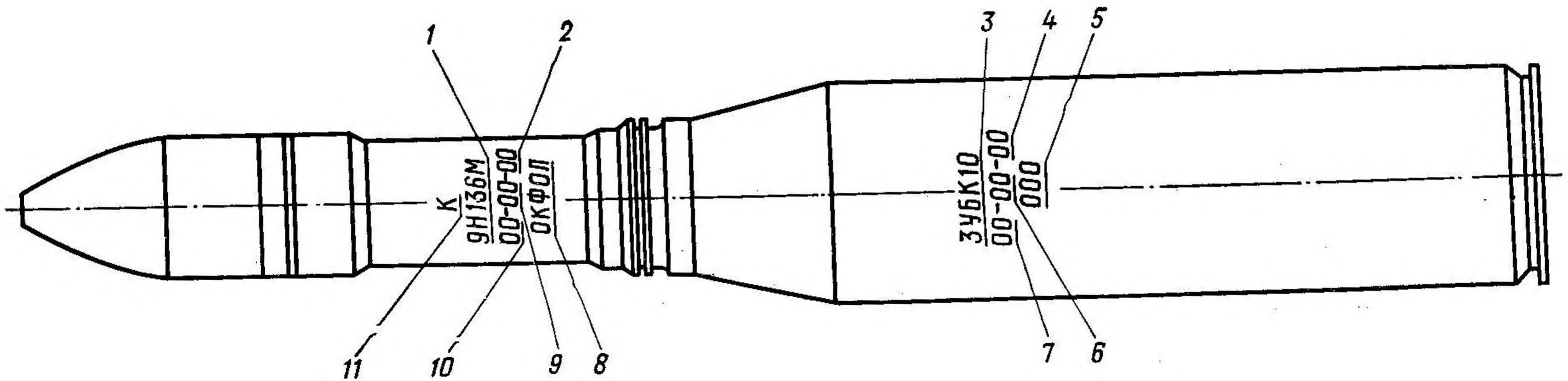
Рис. 32. Маркировка выстрела 3УБК10:
