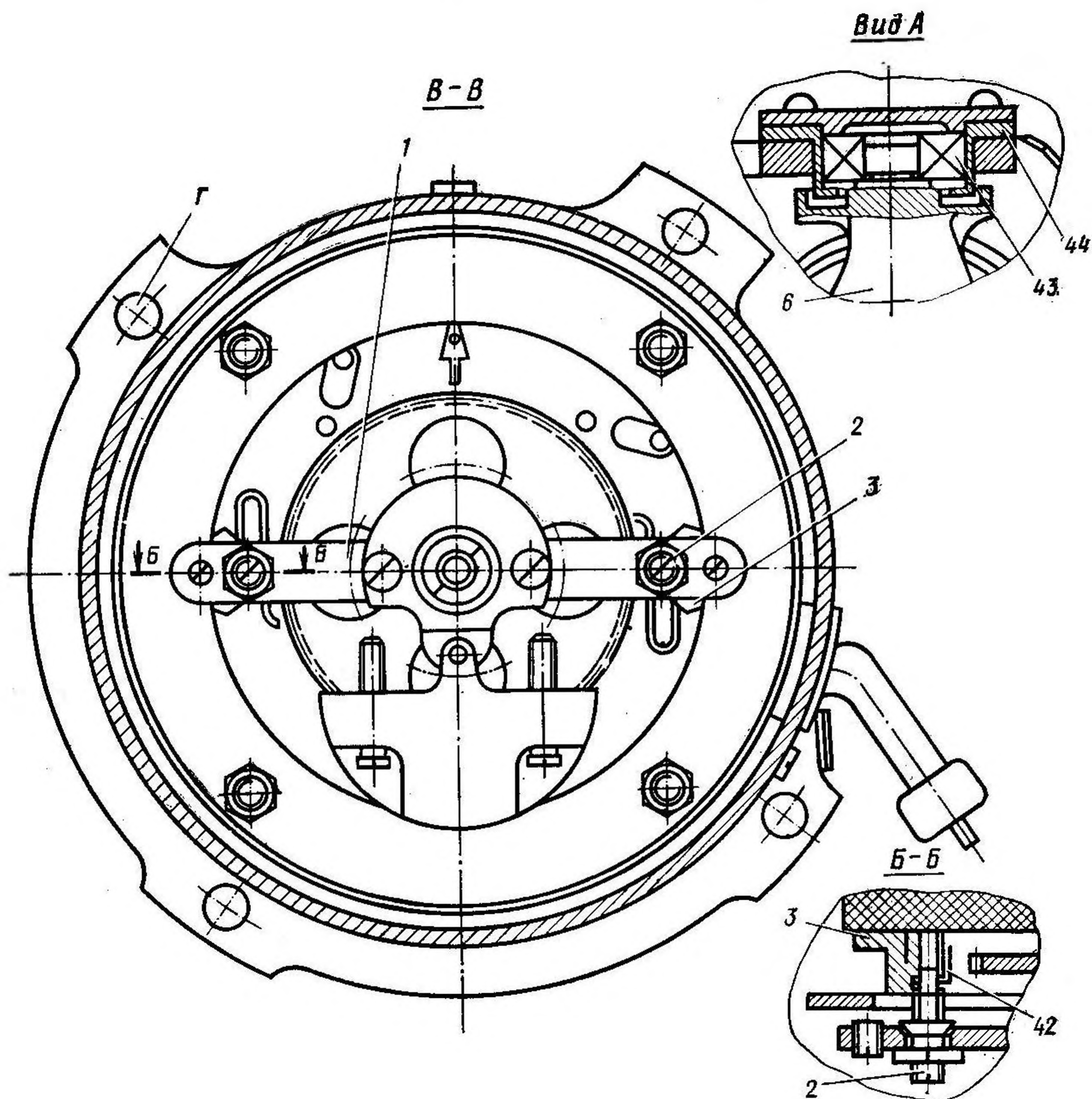
Рис. 27. Гироко
