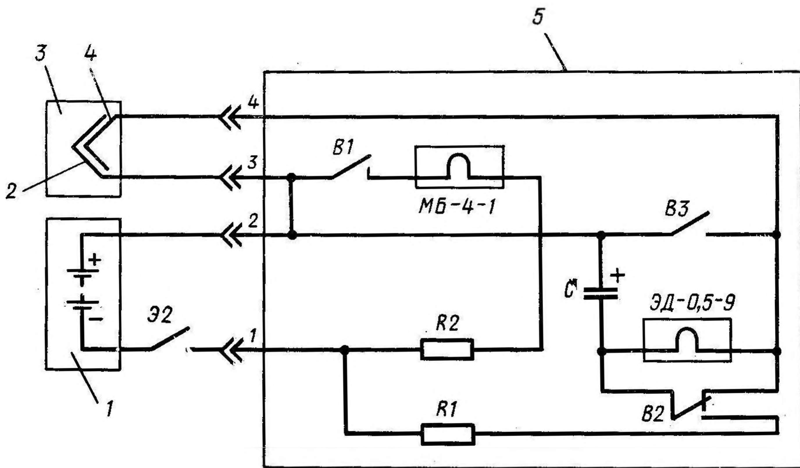
Рис. 19. Электрическая схема предохранительно-исполнительного механизма 9Э295:
