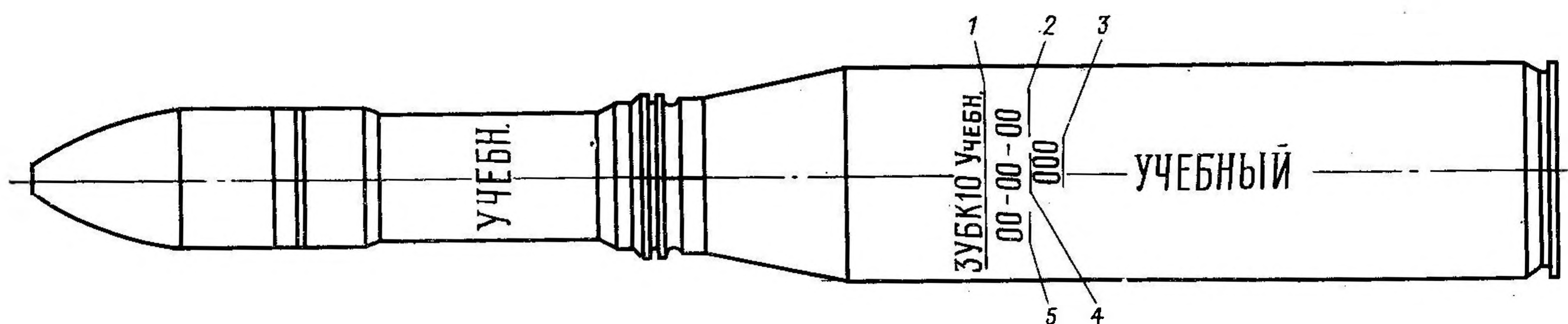
Рис. 34. Маркировка учебного выстрела с действующей аппаратурой:
