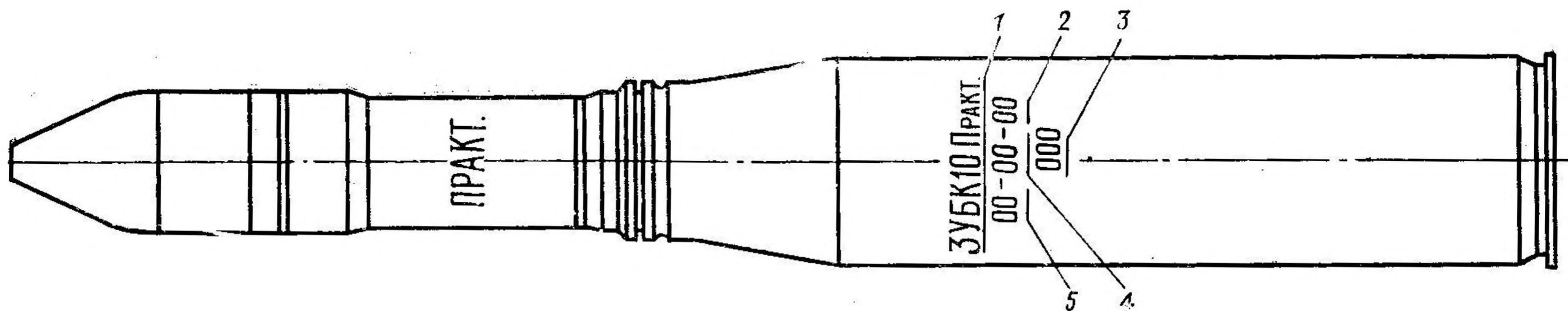
Рис. 33. Маркировка практического выстрела:
