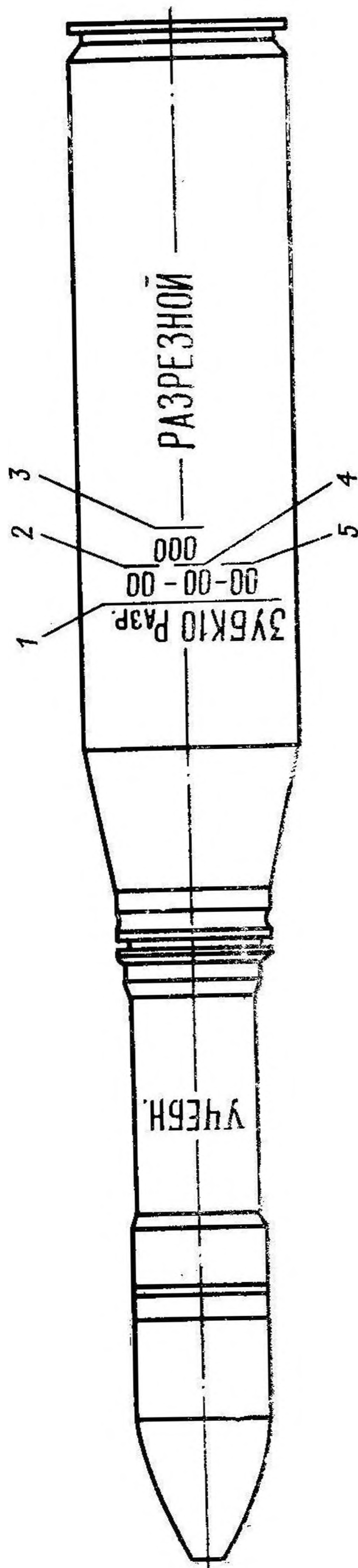
Рис. 36. Маркировка учебного разрезного выстрела:
