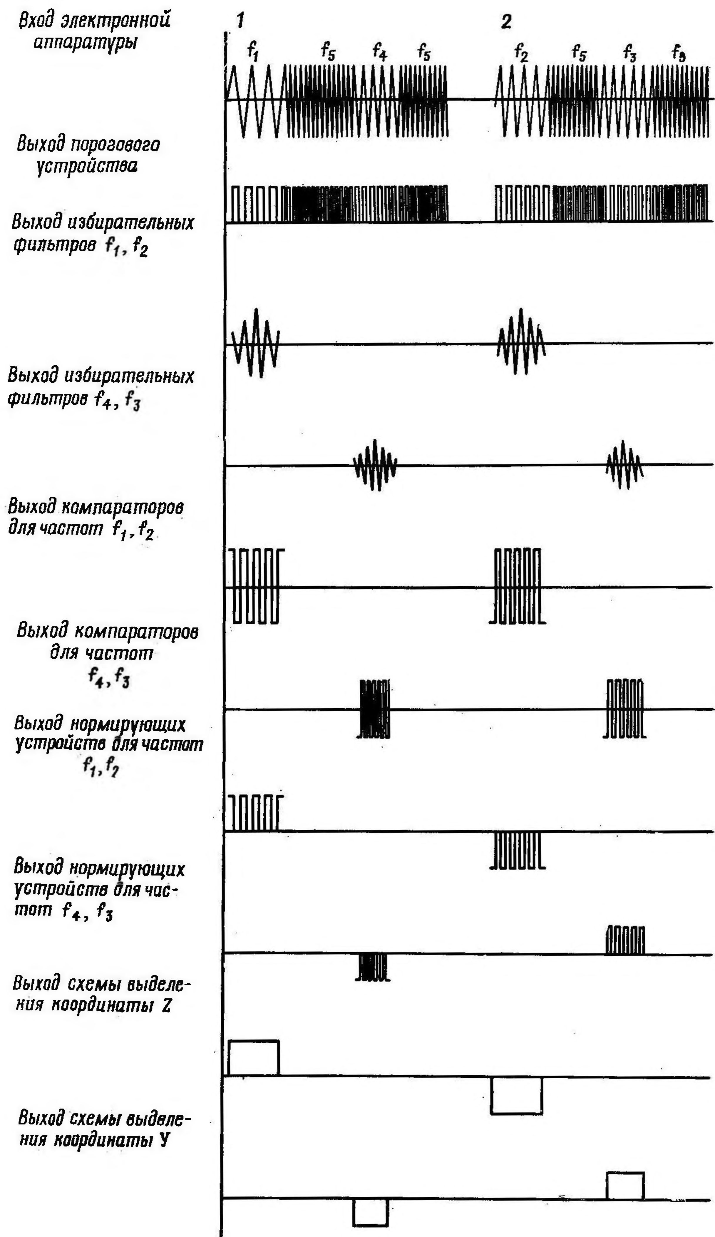
Рис. 9. Форма сигнала для характерных точек электронной аппаратуры
