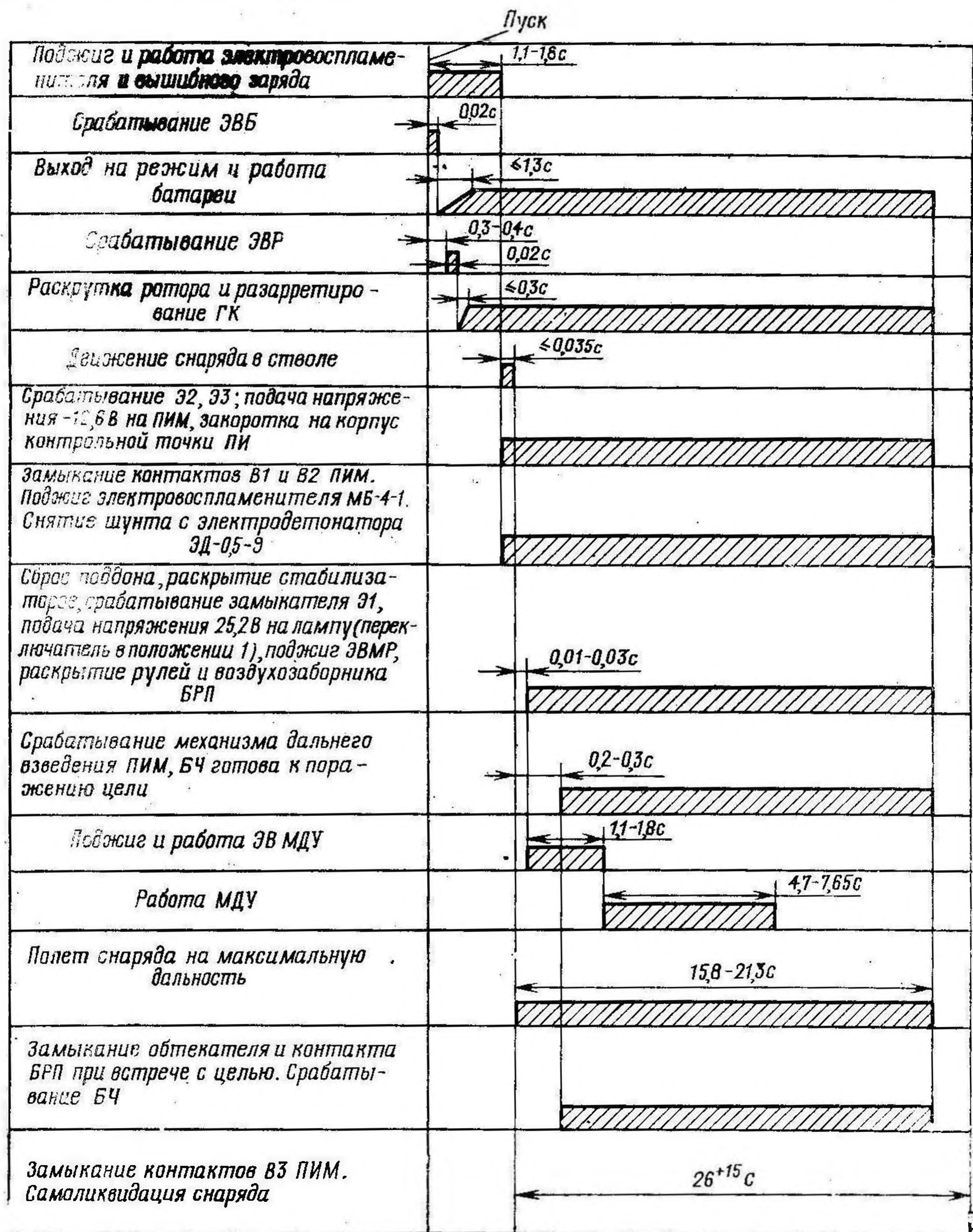
Рис. 29. Временная циклограмма работы выстрела ЗУБК10
