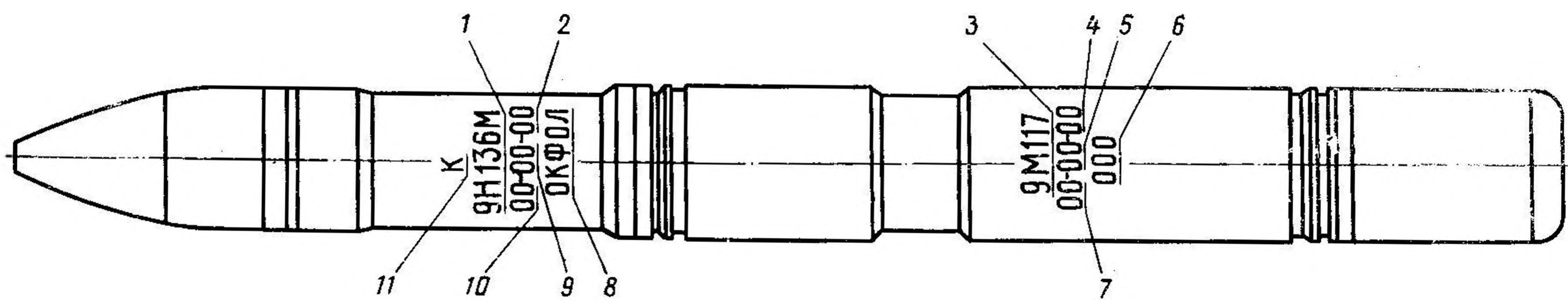
Рис. 31. Маркировка управляемого снаряда 9М117:
