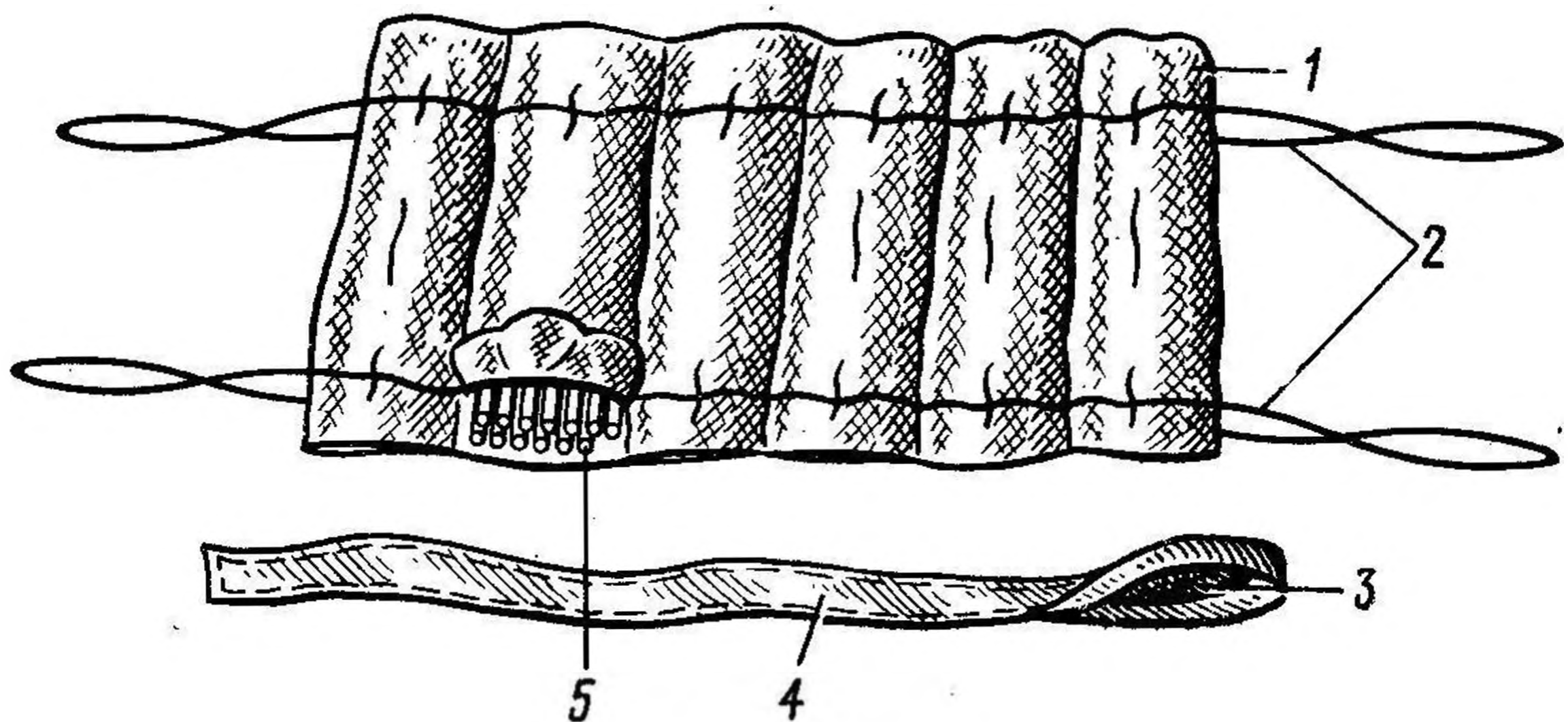
Рис. 5. Вышибной заряд 9Х918:
