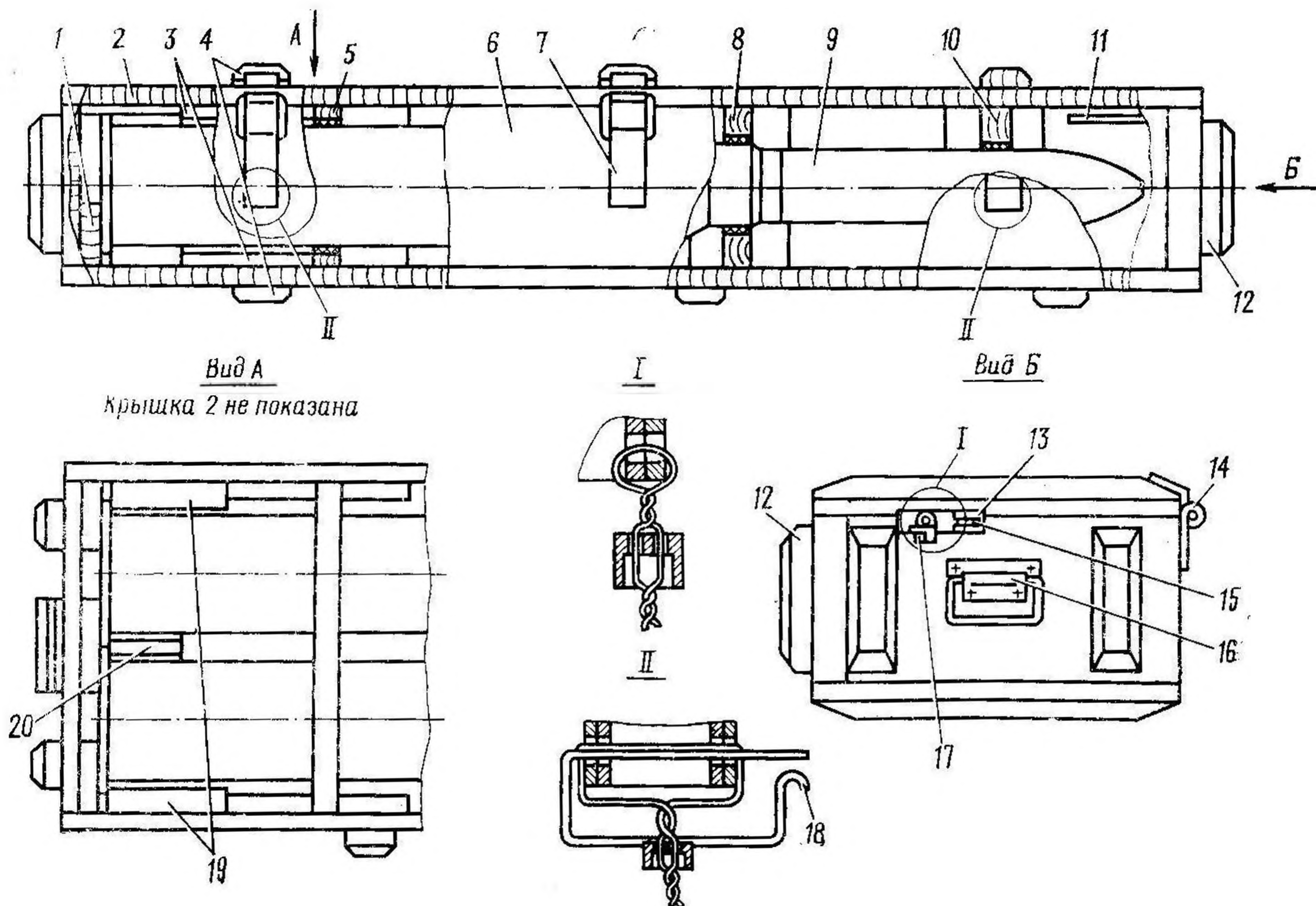
Рис. 37. Упаковка 9Я58 с выстрелами ЗУБК10:
