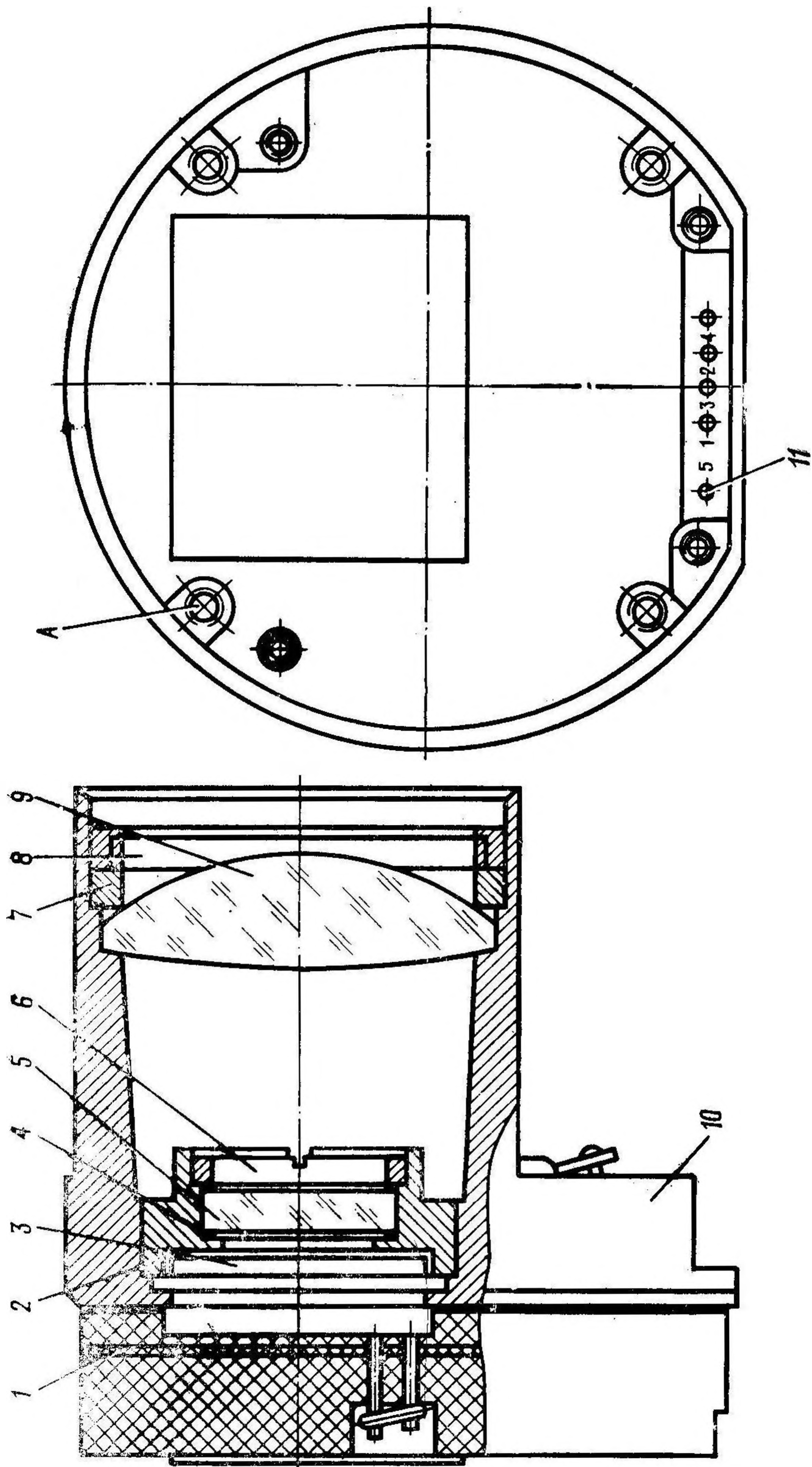
Рис. 25. Приемник излучения:
