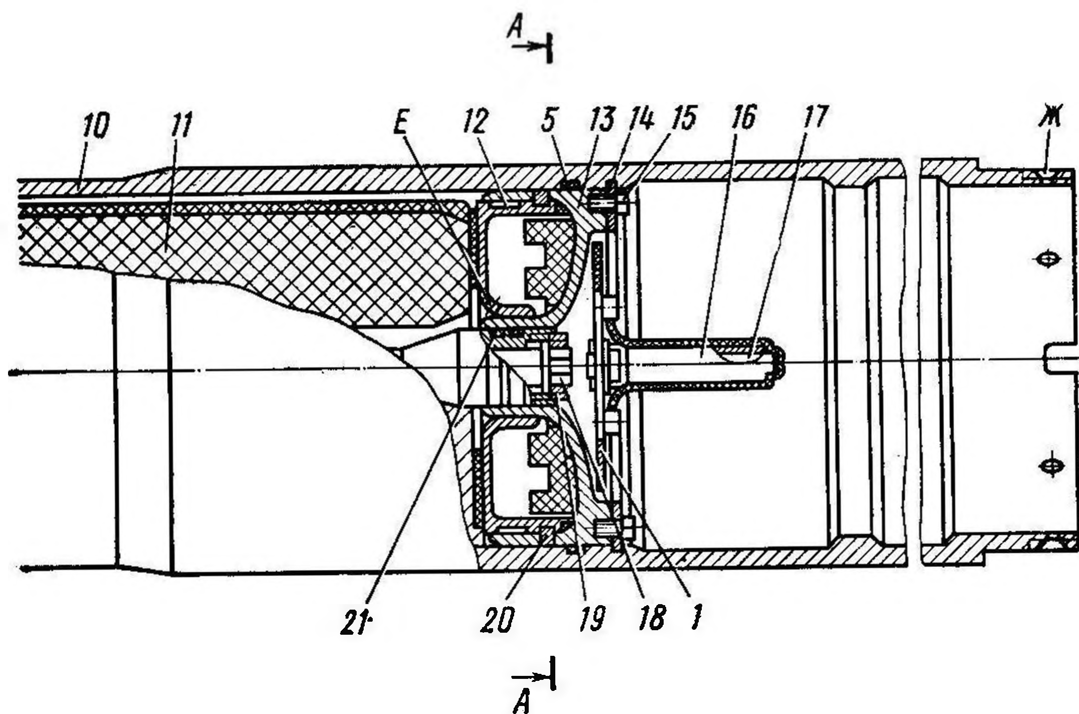
Рис. 20. Маршевая двигательная установка:
