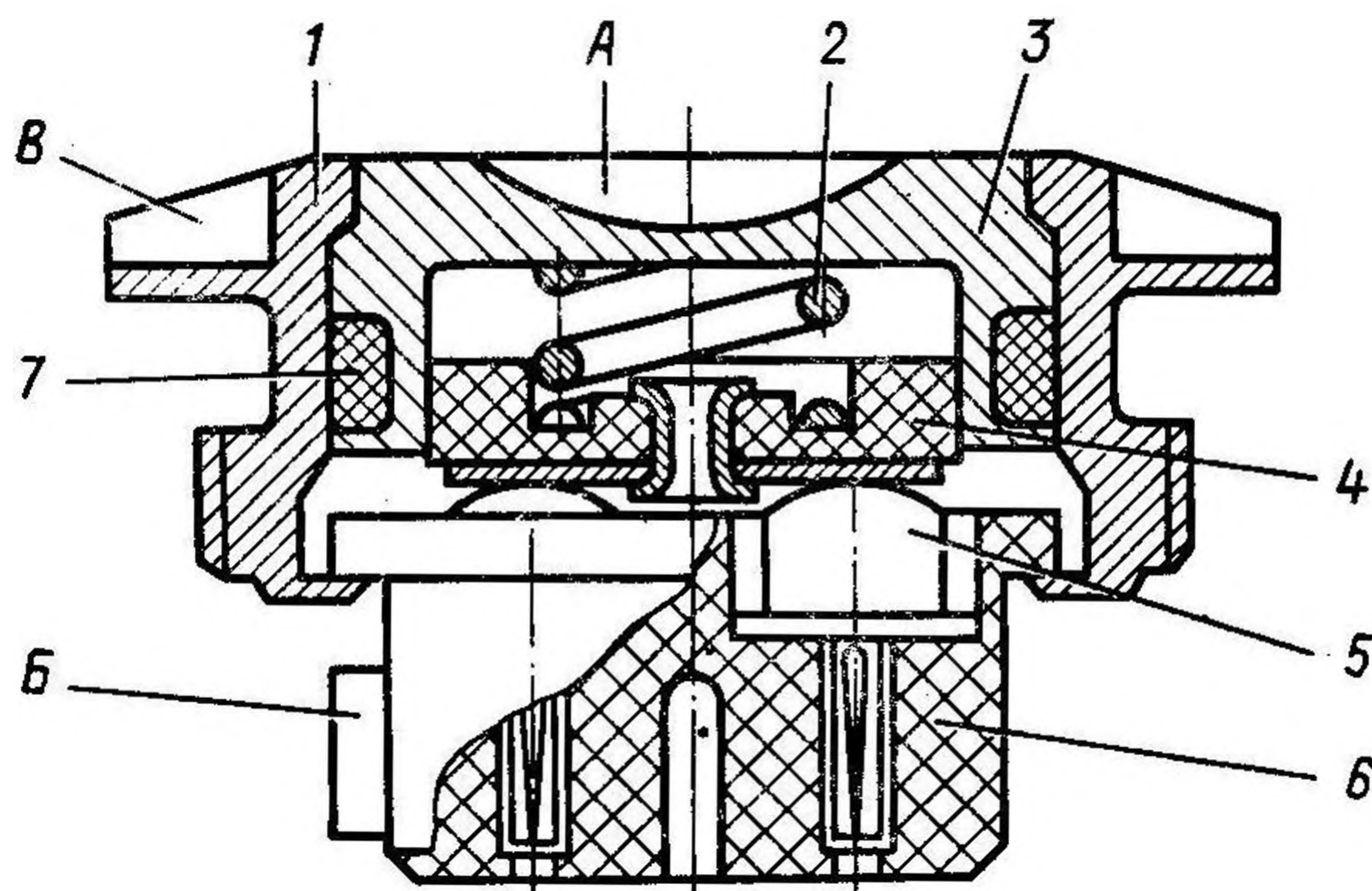
Рис. 14. Переключатель:
