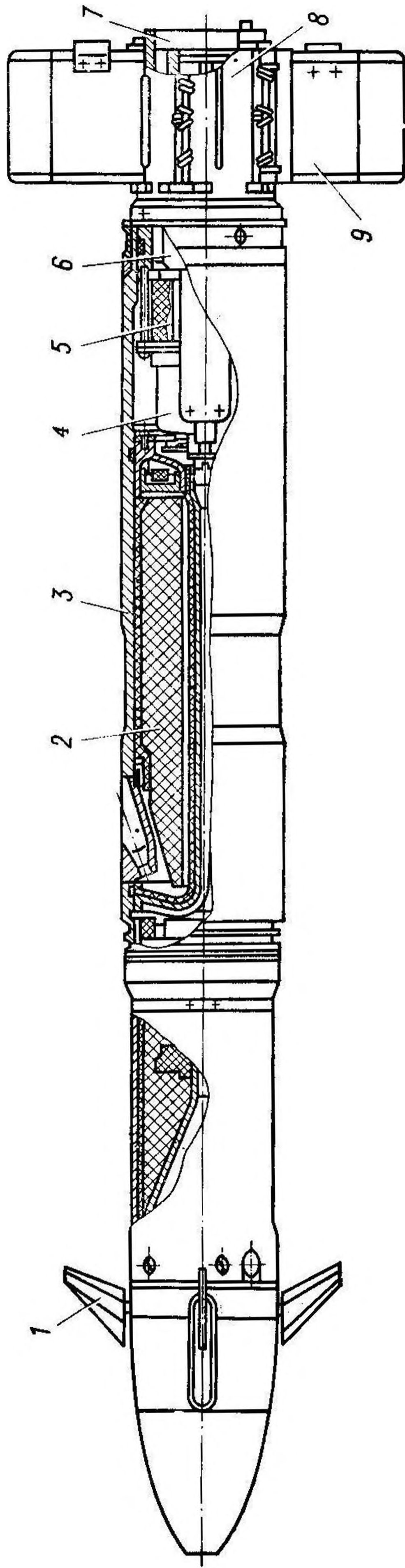
Рис. 7. Снаряд 9М117 в полете (вид в разрезе):
