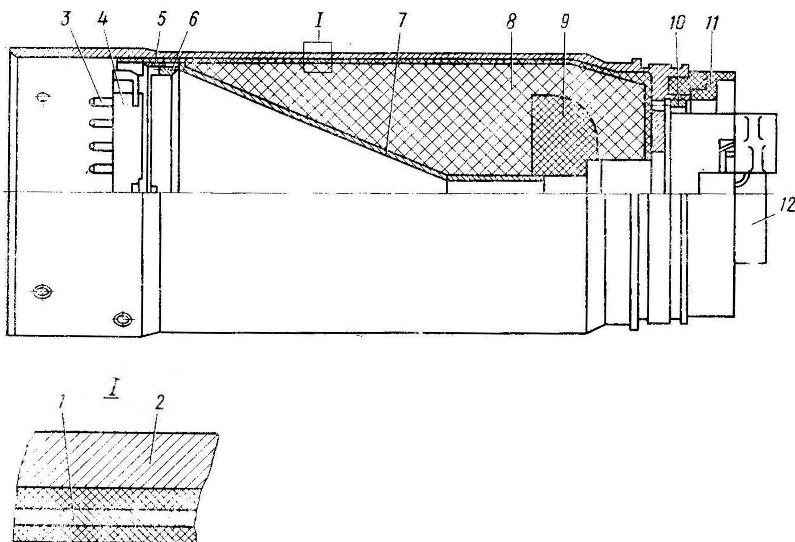
Рис. 17. Боевая часть 9Н136М:
