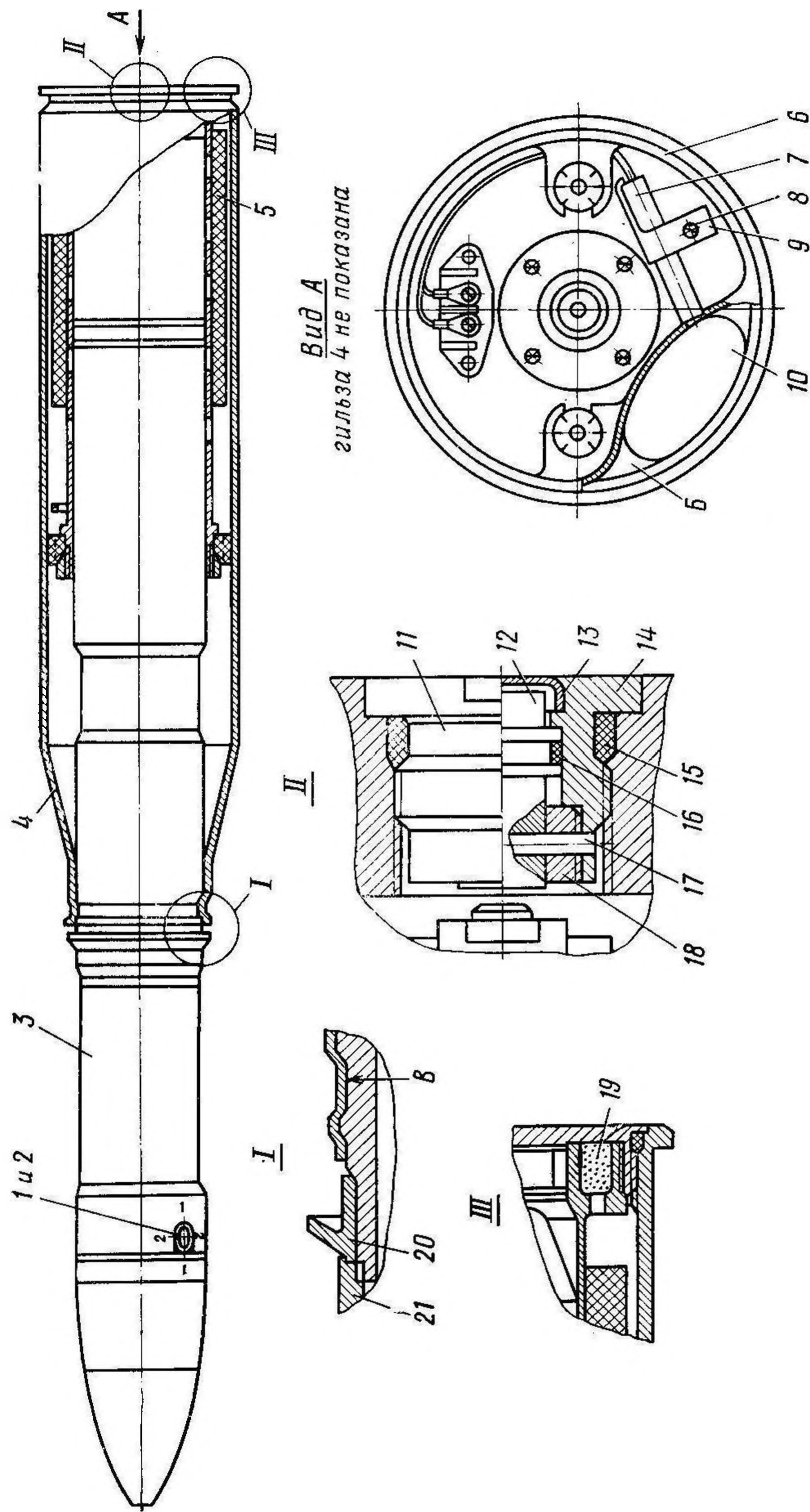
Рис. 2. Выстрел ЗУБК10 (вид в разрезе):
