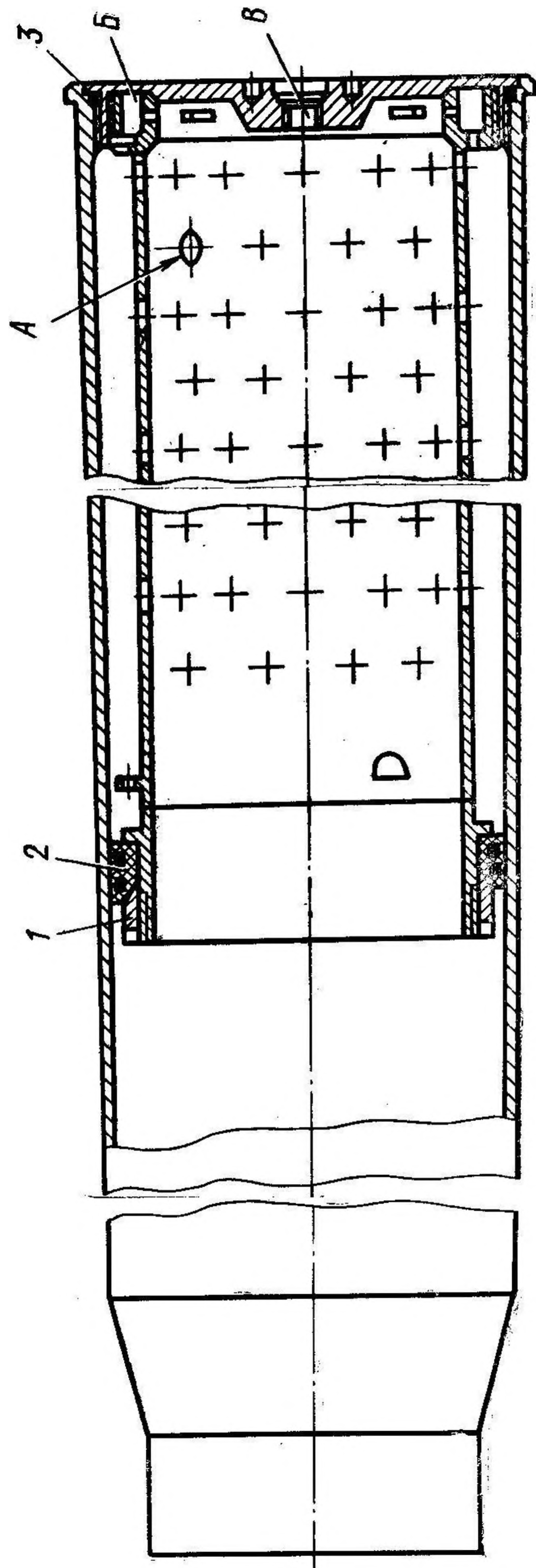
Рис. 4. Гильза (вид в разрезе):
