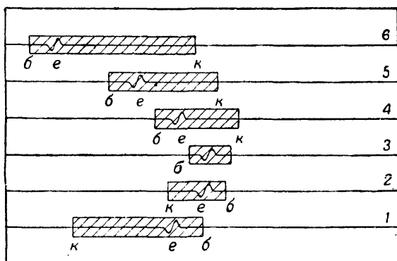
Рис. 113. Лента с вырезанными окнами. За начальный звукоприемник взят третий
