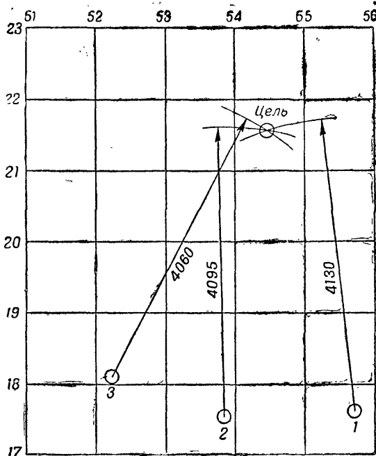
Рис. 97. Схема определения координат целей с помощью секундомера по рассчитанным дальностям
