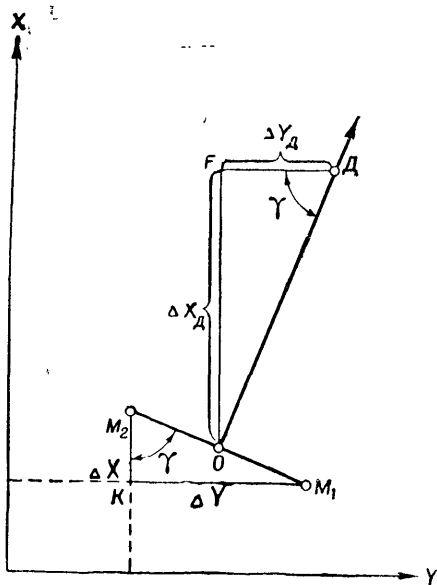
Рис. 94. Схема определения координат точек на директрисе O и D
