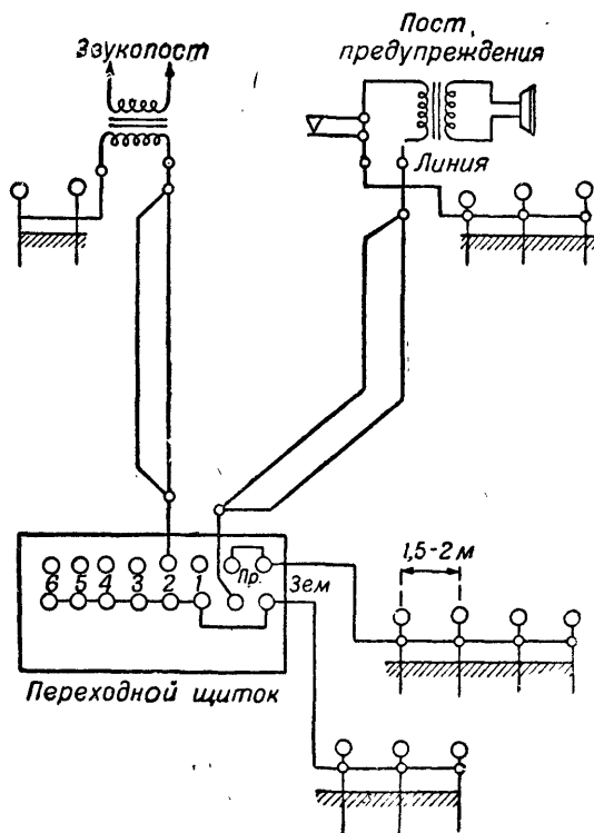
Рис. 152. Работа на однопроводной линии второго звукового поста и поста предупреждения
