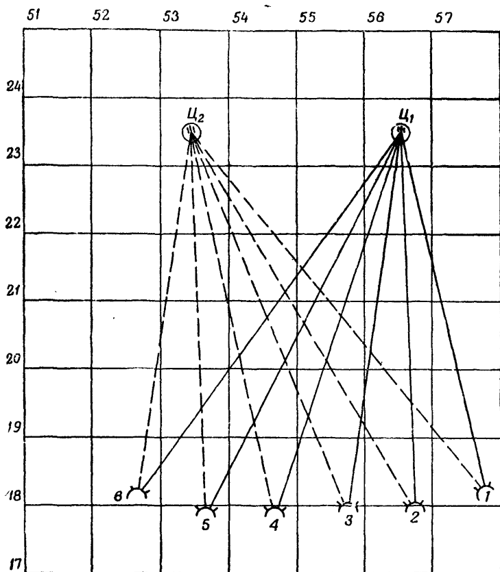
Рис. 100. Схема относительного расположения двух целей и шести звукоприемников
