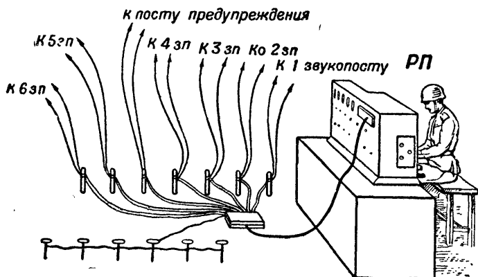
Рис. 148. Направление линий связи на посты от центральной станции
