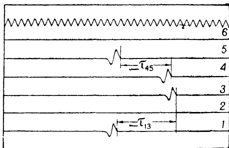
Рис. 69. Отсчеты между первым — третьим и четвертым — пятым звукоприемниками
