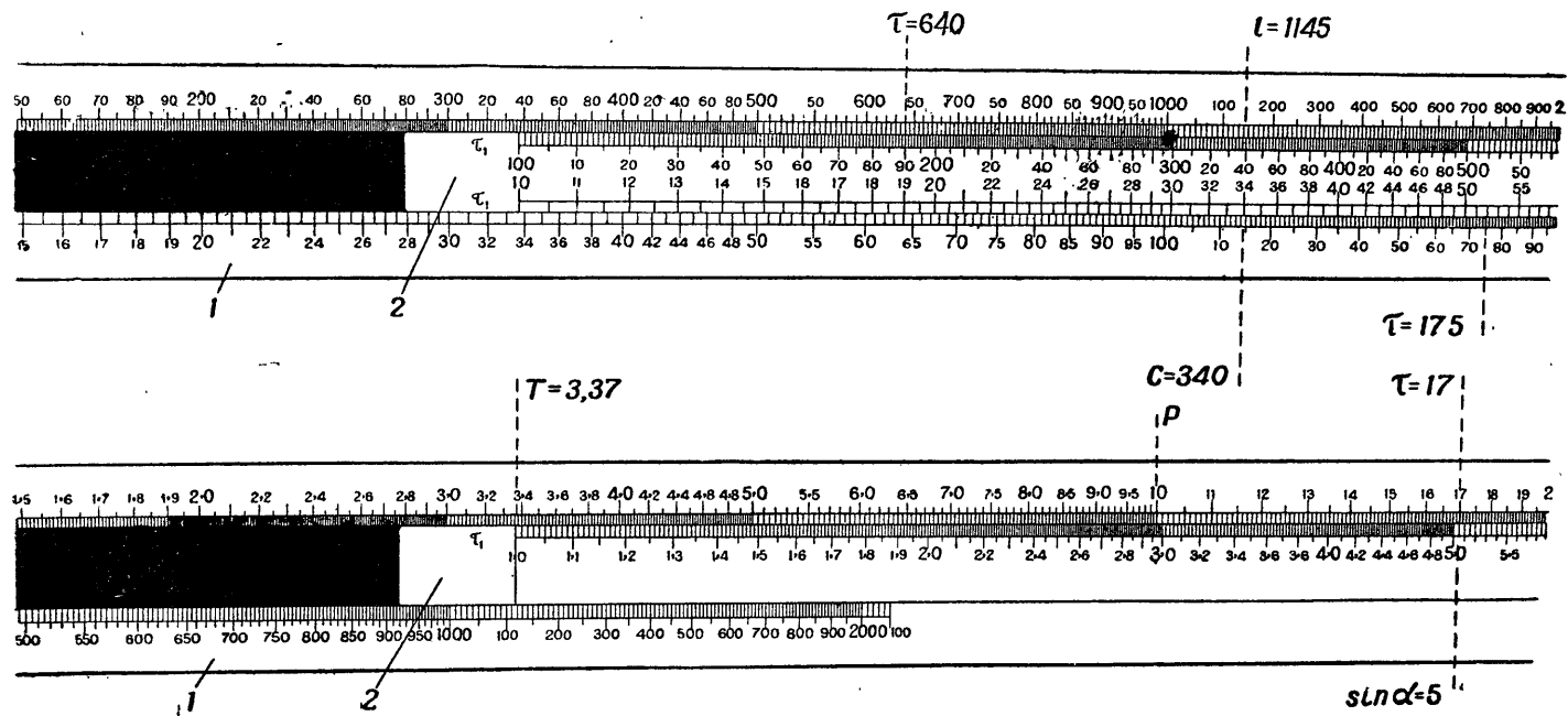
Рис. 86. Счетная звукометрическая линейка
