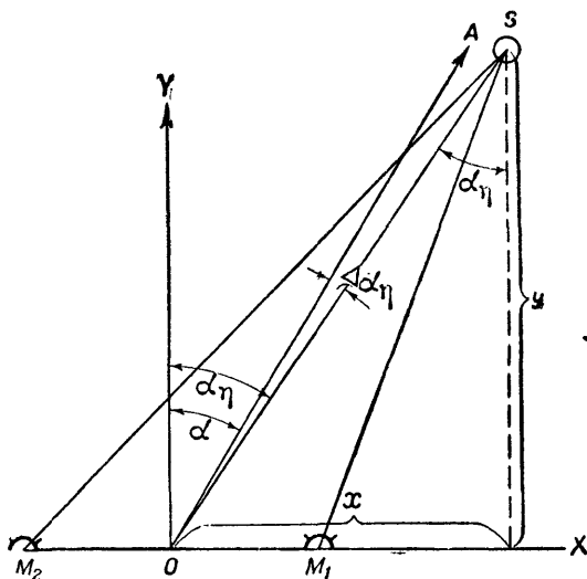
Рис. 46. Схема для вывода поправки на удаление
