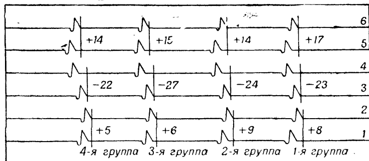
Рис. 83. Четыре группы записей, полученные для определения параллакса перьев
