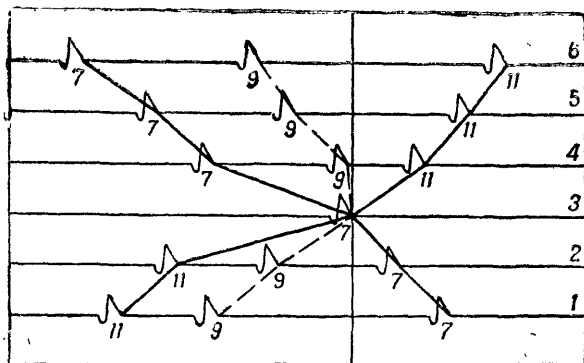
Рис. 125. Графики систем по правым точкам разведучастков 7, 9 и 11 рис. 124
