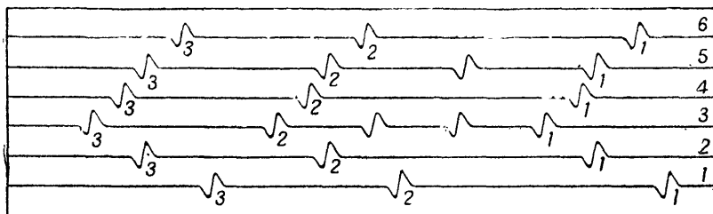
Рис. 123. Лента с записями, полученная при стрельбе трехорудийной батареей
