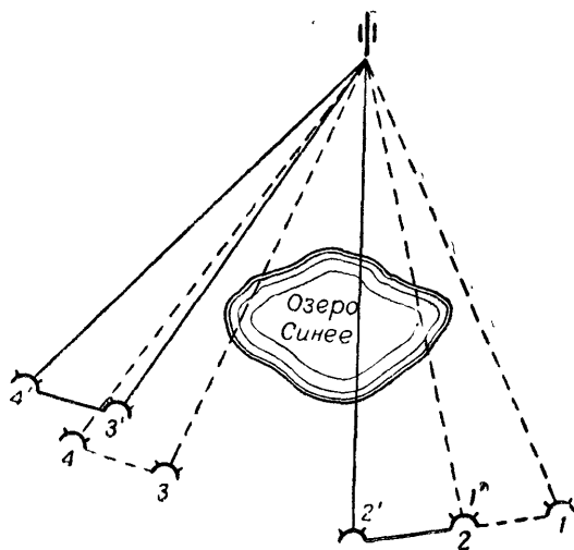
Рис. 143. Правильное (1'—2' и 3'—4') и неправильное (1—2 и 3—4) расположение звукоприемников за озером
