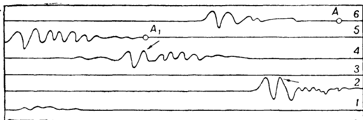
Рис. 76. Определение соответственных точек для снятия отсчетов при плохих началах записей
