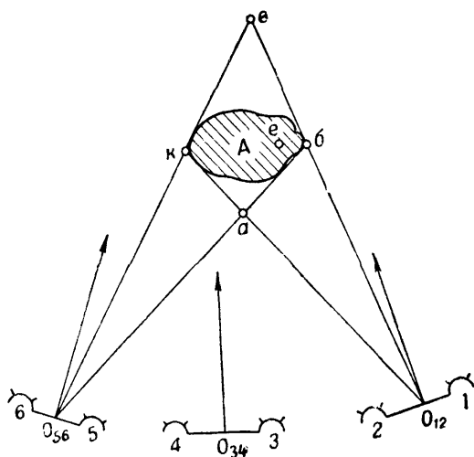
Рис. 108. Разведывательный участок, образованный касательными, проведенными из центров крайних акустических баз
