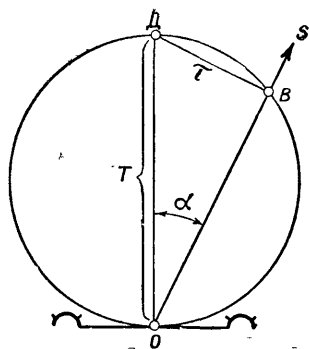
Рис. 88. Определение направления по \tau
