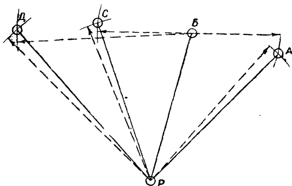
Рис. 171. Схема топографической привязки по звуку
