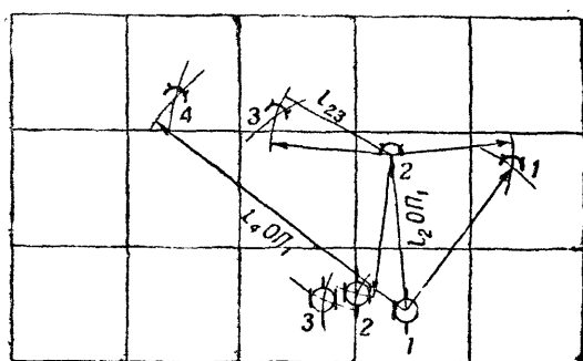
Рис. 172. Схема топографической привязки звуковых постов и огневых позиций по звуку
