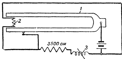
Рис. 64. Схема работы камертонного механизма
