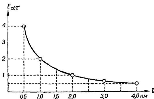
Рис. 130. Зависимость ошибки разброса E_{\alpha\tau} от длины базы l
