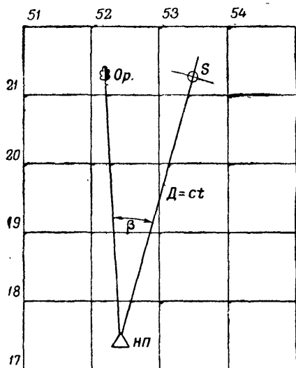
Рис. 98. Определение положения цели с одного пункта по углу и дальности
