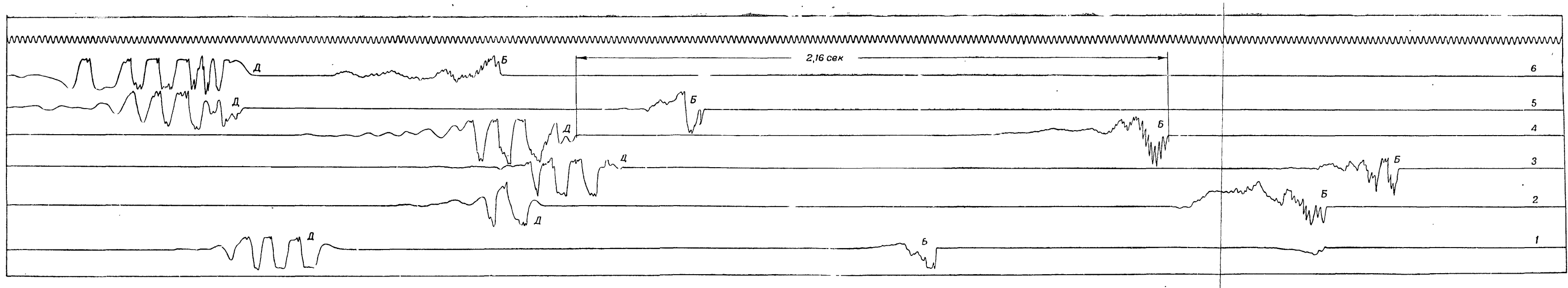
Рис. 20. Записи дульной и баллистической волн 122 мм пушки
