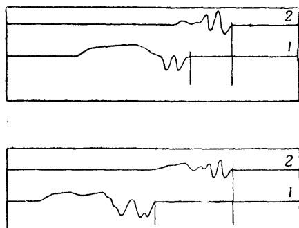
Рис. 78. Вверху записи с истинными началами, внизу запись первого пера дана с опозданием на один период
