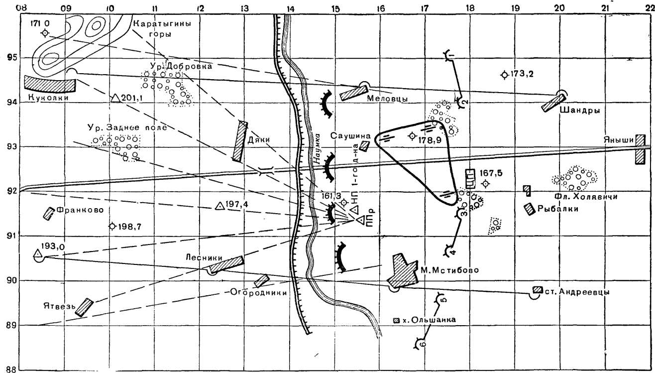
Рис. 159. Схема развертывания батареи звуковой разведки в период подготовки артиллерийского наступления
