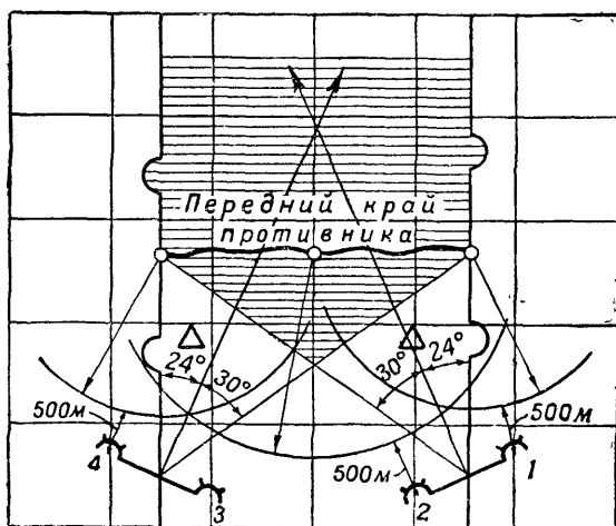
Рис. 163. Район надежной работы при засечке 81-мм минометов при средних условиях слышимости
