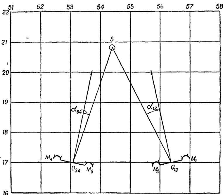
Рис. 41. Определение местоположения цели при наличии двух баз
