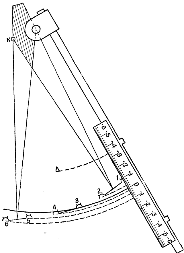
Рис. 115. Схема работы с помощью планшетной линейки
