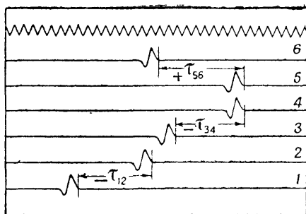
Рис. 68. Отсчеты трех акустических баз, отмеченные соответствующими индексами
