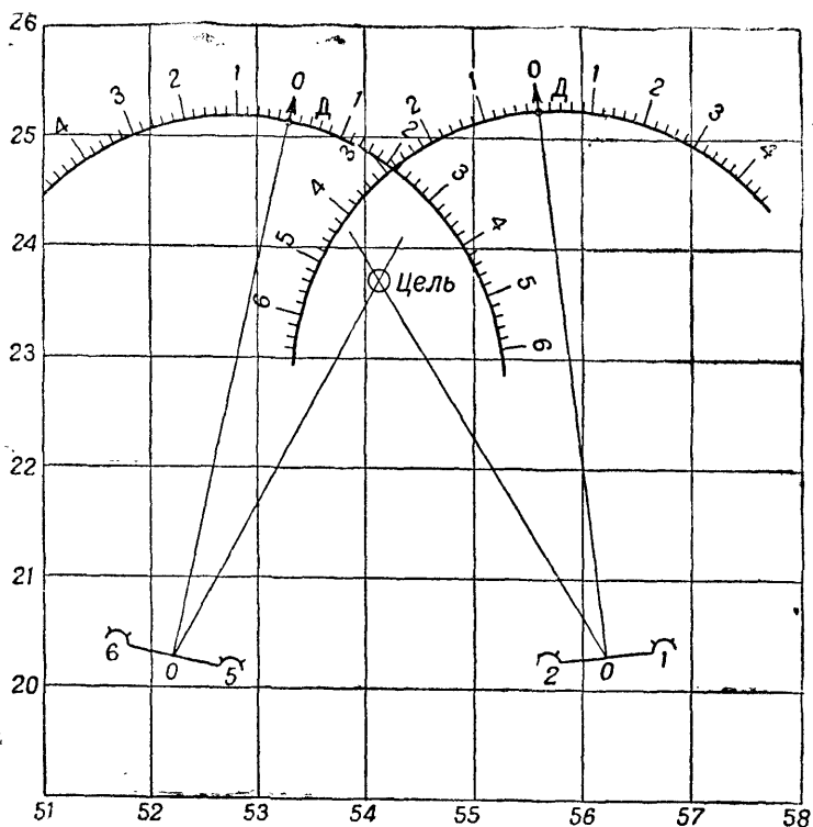
Рис. 92. Построительные дуги с нанесенными делениями
