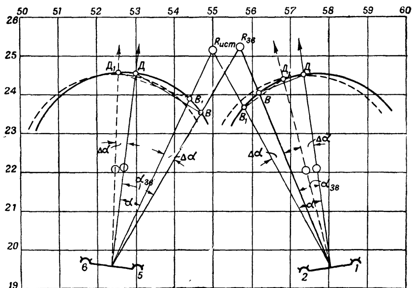
Рис. 137. Исключение систематической ошибки поворотом директрис
