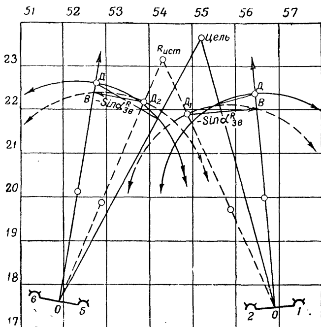
Рис. 138. Построение истинной директрисы по звуковому реперу
