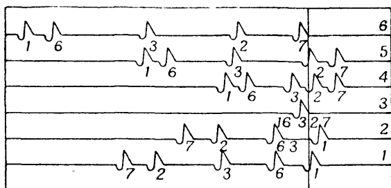
Рис. 107. Записи звуковых волн от целей, указанных на рис. 105, при совмещении начал их на линии третьего пера
