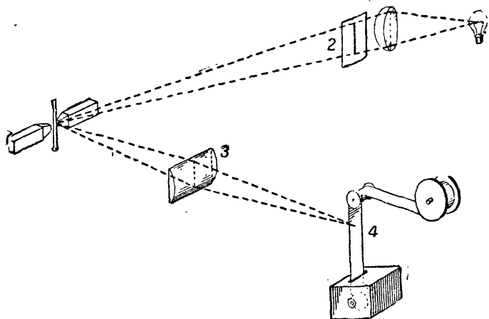
Рис. 66. Схема пишущего механизма с фотооптической записью звукометрической станции бывшей германской армии
