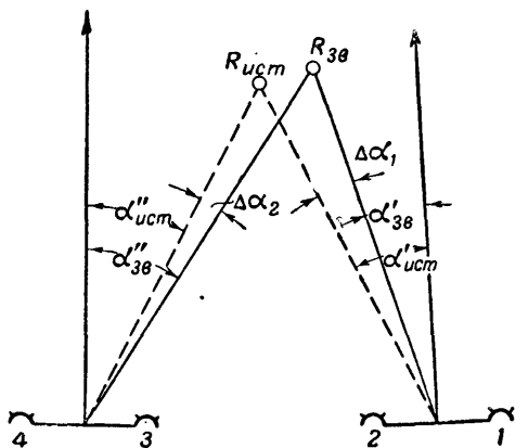
Рис. 136. Определение систематической ошибки при нанесении на планшет истинного положения репера R_{ист} и положения, определенного звуковой разведкой R_{зв} .
