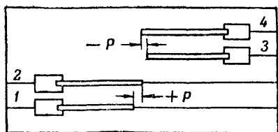
Рис. 82. Определение знака поправки на параллакс перьев
