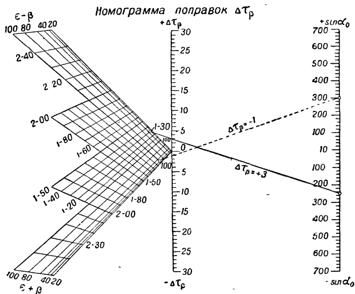
Рис. 60. Номограмма поправок на наклон баз и угол места цели
