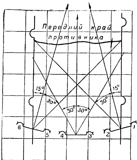
Рис. 147. Район надежной работы при большом удалении звуковых постов от переднего края противника
