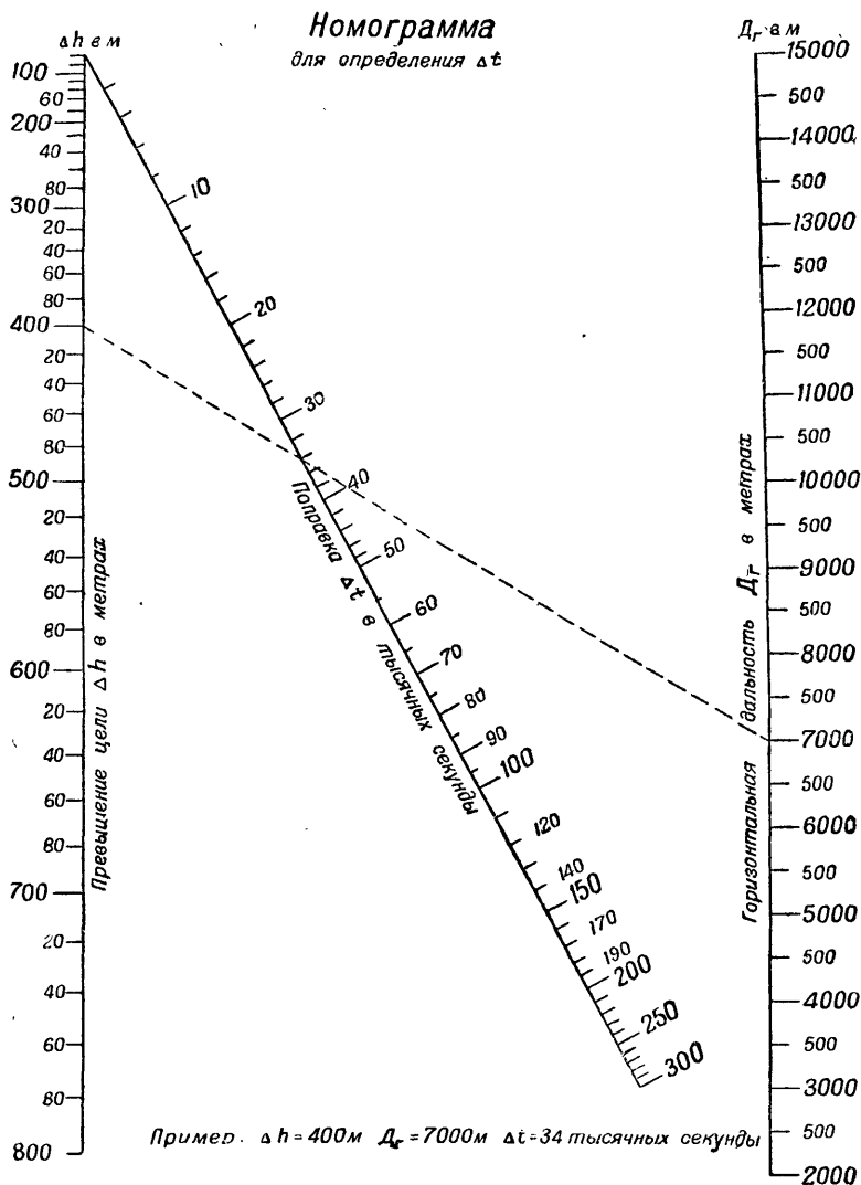
Рис. 58. Номограмма для определения \Delta t
