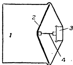
Рис. 61. Схема звукоприемника с угольным микрофоном
