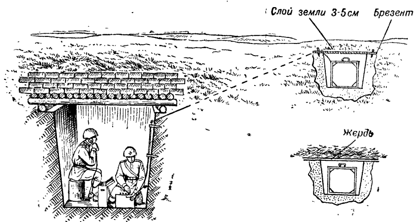
Рис. 149. Блиндаж и окоп звукоприемника на посту звуковой разведки
