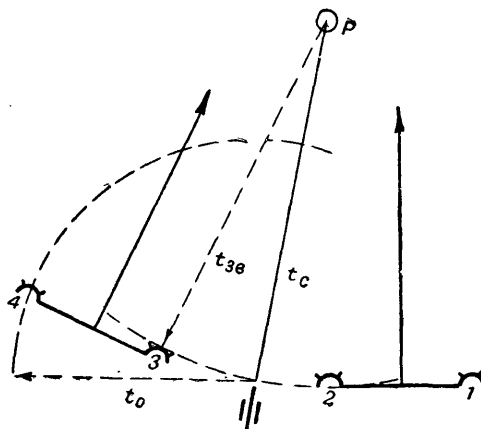
Рис. 166. Схема расчета темпа огня
