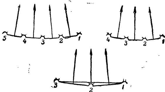
Рис. 95. Схема образования трех акустических баз при различном числе звукоприемников
