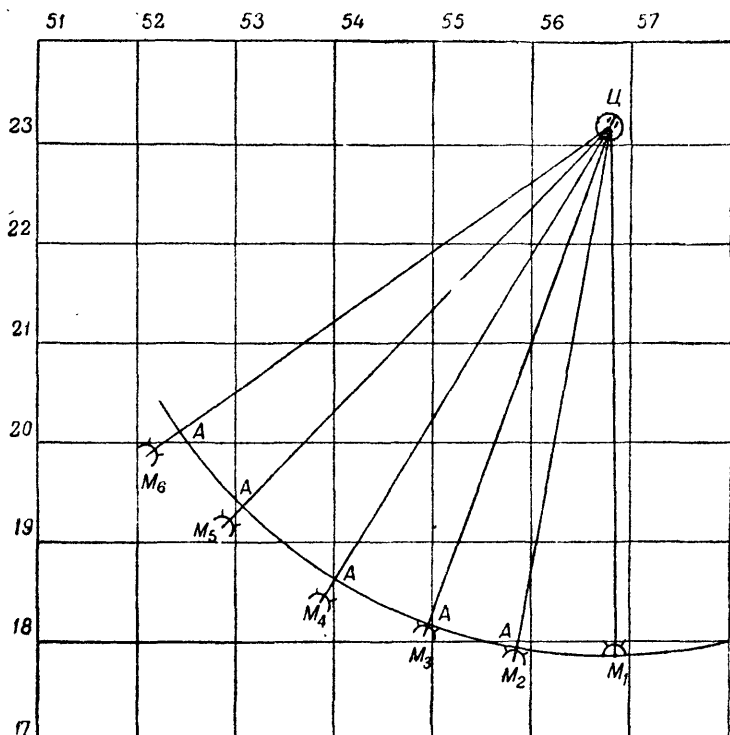
Рис. 103. Схема относительного расположения одной цели и шести звукоприемников
