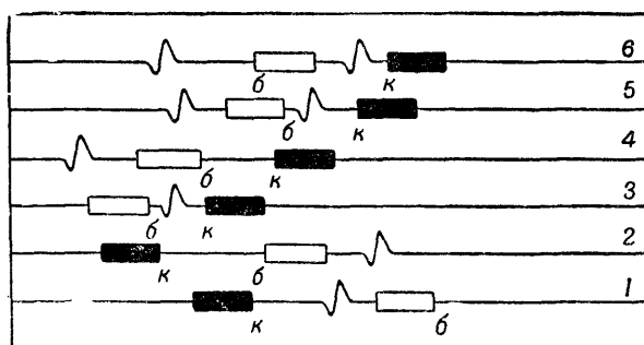
Рис. 117. Во все окна дешифратора попало по одной записи
