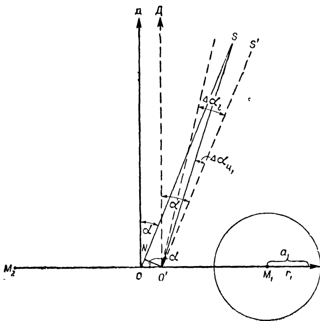
Рис. 131. Влияние ошибки в привязке правого звукового поста относительно левого на определение угла \alpha (ошибка направлена вдоль базы)
