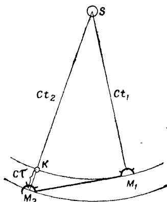
Рис. 37. Источник звука расположен на разном удалении от звукоприемников
