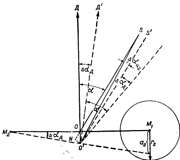
Рис. 132. Влияние ошибки в привязке правого звукового поста относительно левого на определение угла \alpha (ошибка направлена перпендикулярно базе)
