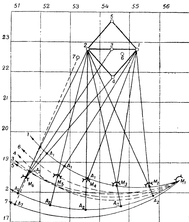
Рис. 105. Схема относительного расположения целей, находящихся в четырехугольнике и в вершинах его, относительно звукоприемников
