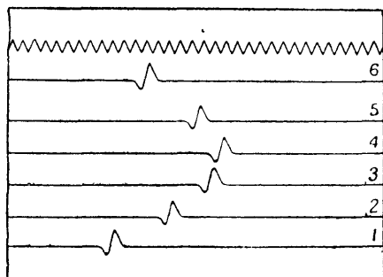
Рис. 67. Записи на ленте при работе шести звукоприемников
