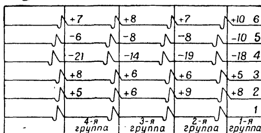
Рис. 84. Определение параллакса перьев по отношению к записи пера первого звукприемника
