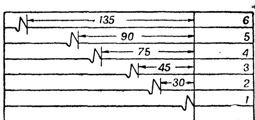
Рис. 104. Записи звуковых волн от цели, указанной на рис. 103
