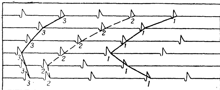
Рис. 102. Расшифрованная лента с записями трех целей
