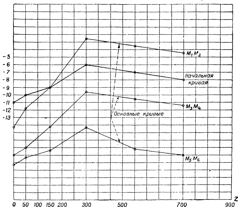
Рис. 55. Планшетка с нанесенными на ней начальной и основными кривыми для трех баз
