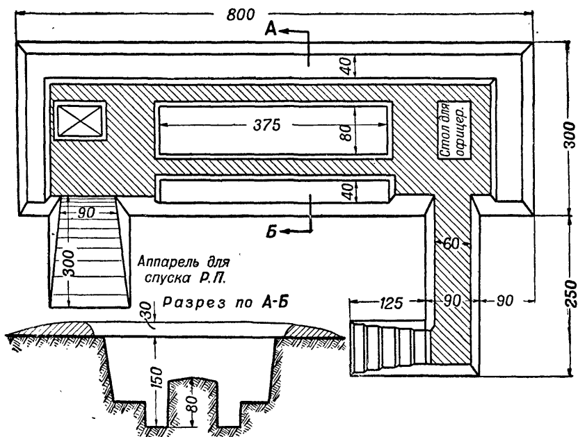
Рис. 154. План окопа центрального пункта
