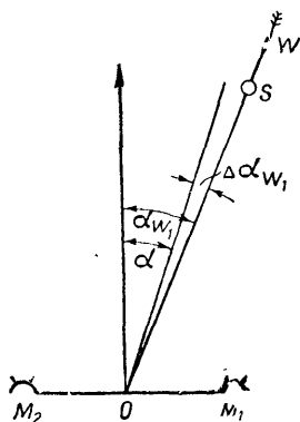
Рис. 47. Ошибка в определении угла \alpha , получаемая вследствие изменения скорости звука под влиянием ветра
