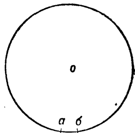
Рис. 7. Небольшой участок сферической волны а б принимается за волну плоскую
