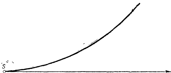
Рис. 26. Искривление звукового луча при уменьшении скорости звука с высотой
