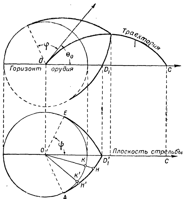
Рис. 19. Вид баллистической волны в плоскости стрельбы и в плоскости горизонта орудия
