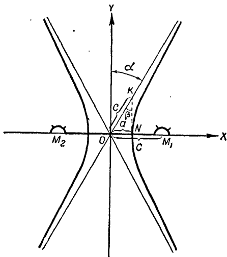
Рис. 45. Гипербола и ее асимптоты
