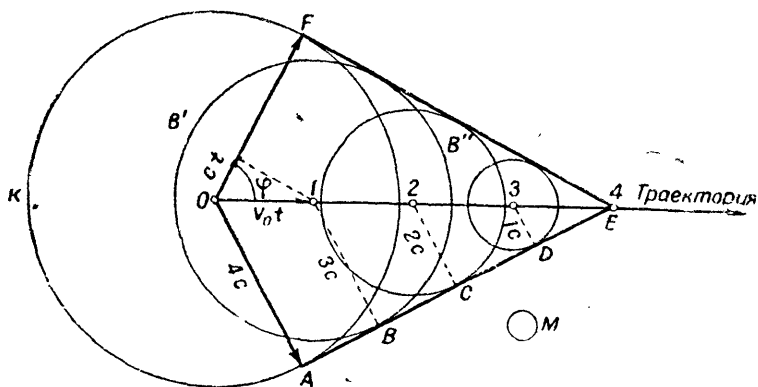
Рис. 18. Схема образования баллистической волны
