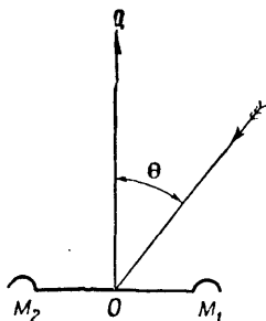
Рис. 50. Схема определения угла \theta
