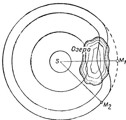
Рис. 22. Деформирование звуковой волны при ее прохождении в летнее жаркое время над озером
