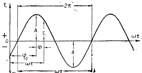
Рис. 4. Графическое изображение колебательного процесса
