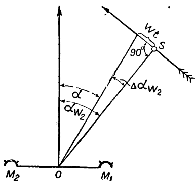
Рис. 48. Ошибка в определении угла \alpha вследствие смещения центра звуковой волны под влиянием ветра
