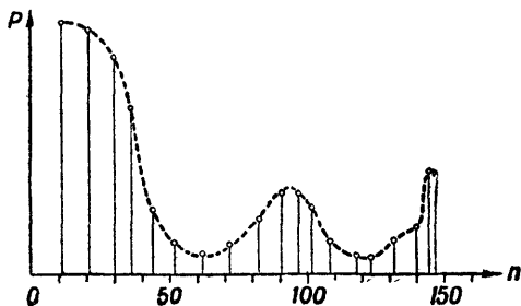
Рис. 5. Акустический спектр дудной волны
