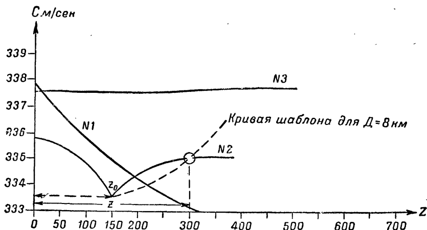
Рис. 52. Графики изменения скорости звука с высотой
