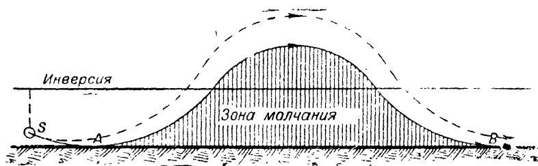
Рис. 30. Преломление акустического луча вначале при понижении, а затем при повышении температуры с высотой
