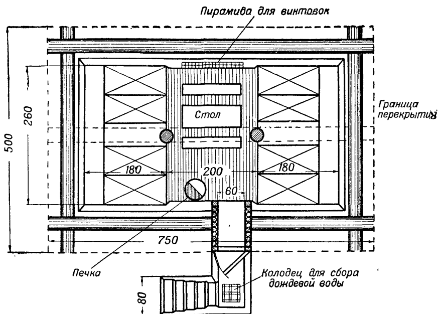
Рис. 156. План землянки для отдыхающей команды центрального пункта
