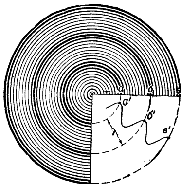
Рис. 6. Схема распространения сферических продольных волн
