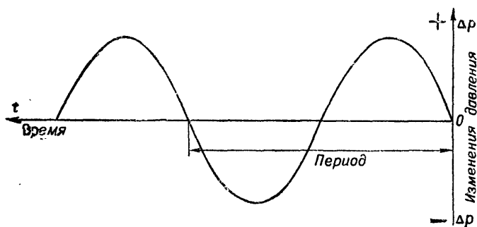
Рис. 9. График изменения давления при прохождении плоской волны
