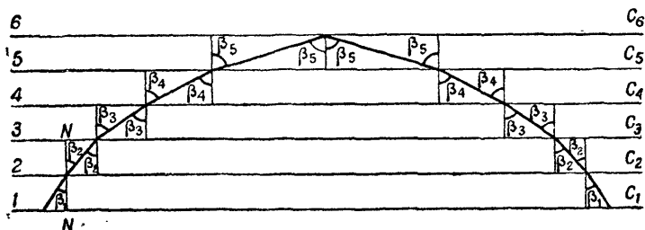
Рис. 24. При переходе из одной среды в другую звуковые лучи претерпевают преломление
