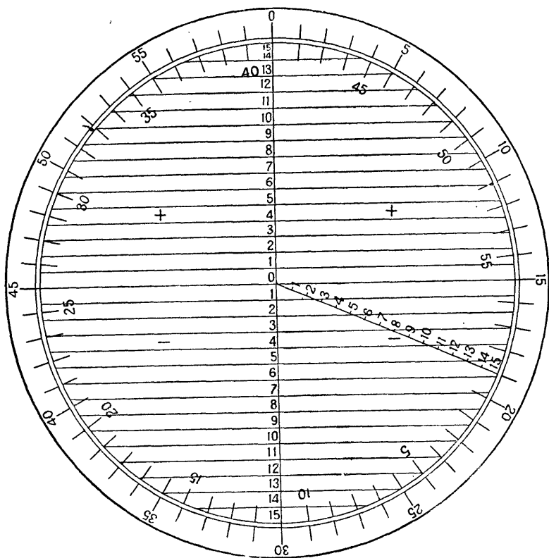
Рис. 56. Круг ветров для определения продольной слагающей ветра
