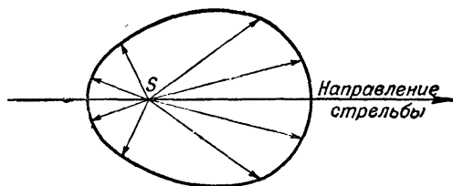
Рис. 15. Распределение давления в дульной волне
