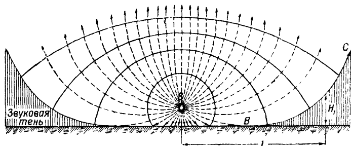
Рис. 27. Искривление звуковых лучей при понижении температуры с высотой
