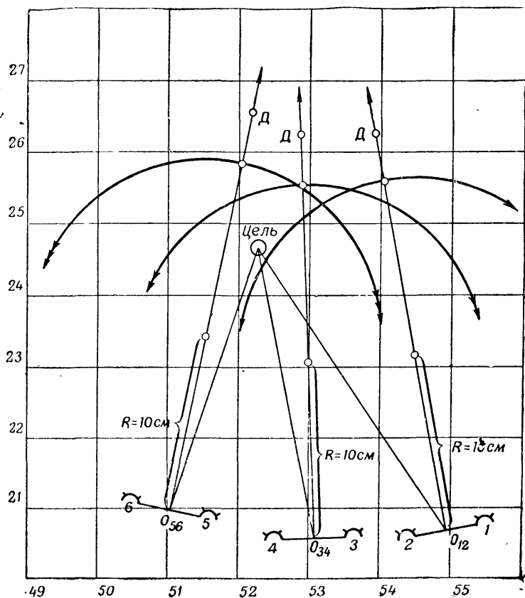
Рис. 93. Определение координат цели при смешанном способе работы
