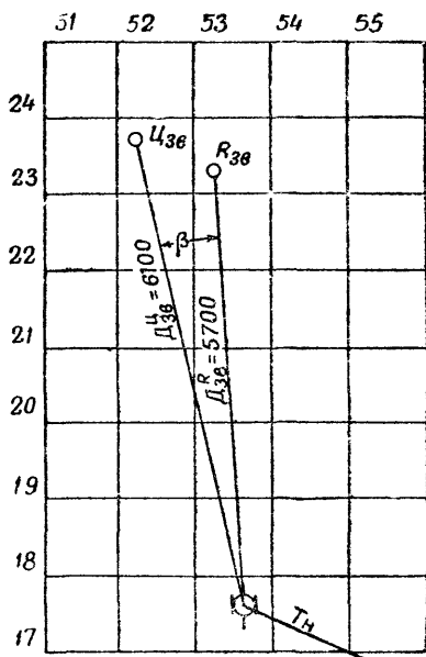
Рис. 169. Измерение отклонения разрывов от звукового репера по огневому планшету
