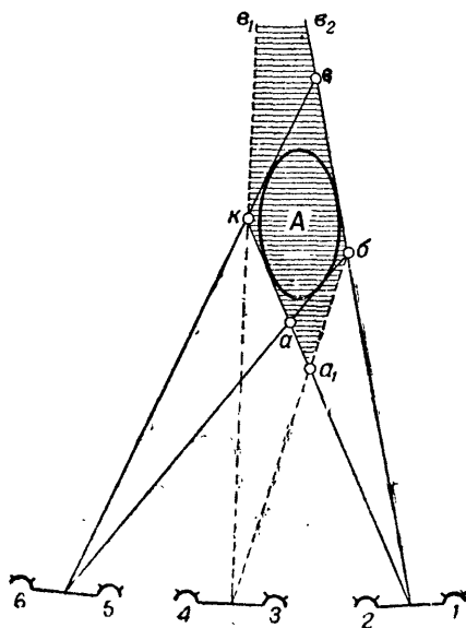
Рис. 111. Разведучасток, образованный касательными, проведенными из центров крайних и средней базы, больше разведучастка, образованного касательными из центров крайних баз
