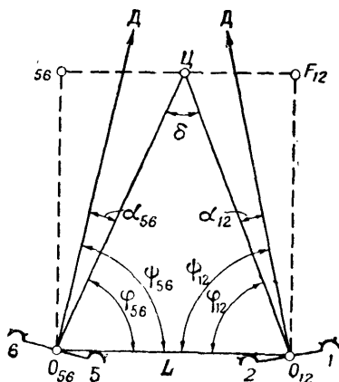
Рис. 96. Схема определения координат цели вычислительным способом
