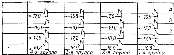
Рис. 85. Группы записей и вертикальные линии к ним для определения параллакса перьев с помощью циркуля и масштабной линейки
