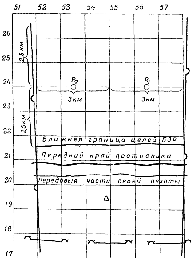
Рис. 135. Расположение реперов в полосе разведки батареи
