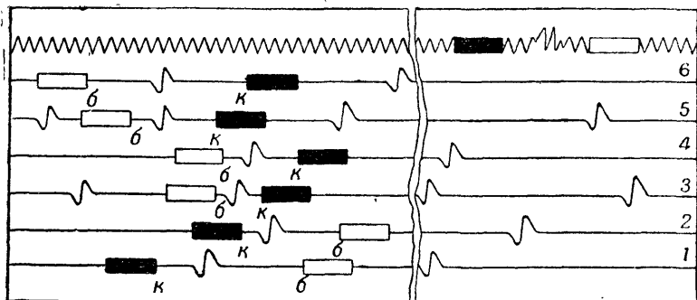
Рис. 118. Записи цели и отметка предупредителя встали в окна дешифратора
