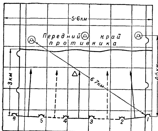
Рис. 164. При нормальном развертывании батареи засечка минометов производится с помощью трех-четырех постов, ближайших к данной цели
