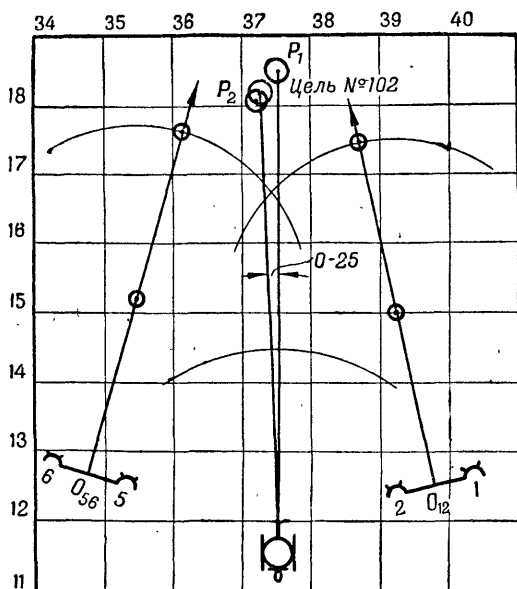
Рис. 168. Измерение отклонений по планшету батареи звуковой разведки
