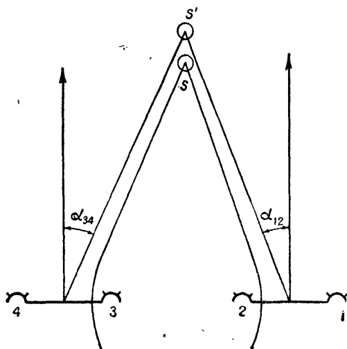
Рис. 44. Определение положения цели с помощью гипербол и асимптот
