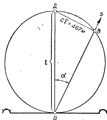
Рис. 87. Определение направления по C\tau
