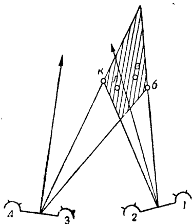
Рис. 110. Разведывательный участок лежит по обе стороны директрисы правой базы
