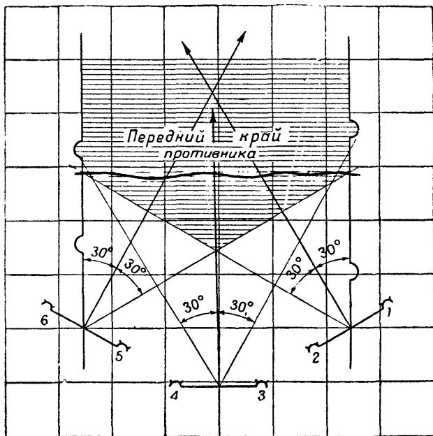
Рис. 146. Район надежной работы
