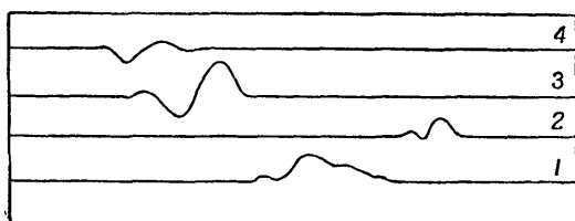
Рис. 74. Записи первого и второго перьев получены при установке звукоприемников в разных условиях слышимости. Записи третьего и четвертого перьев получены при условии, что четвертый звукоприемник был менее чувствителен, чем третий
