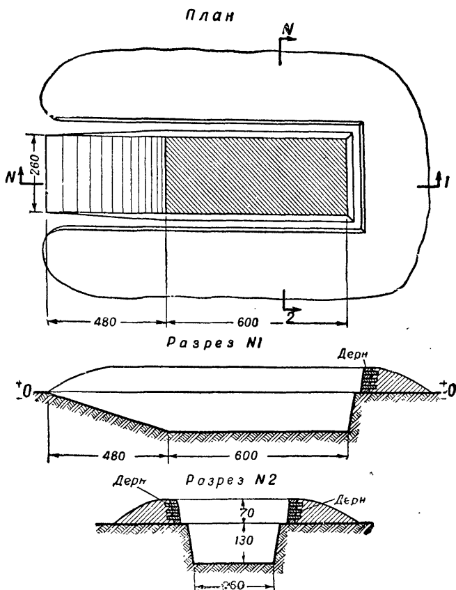
Рис. 158. Котлован для укрытия автотранспорта
