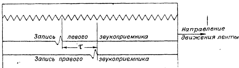
Рис. 40. Записи на ленте при приеме звука двумя звукоприемниками одной базы
