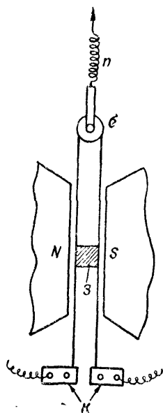
Рис. 65. Схема шлейфа
