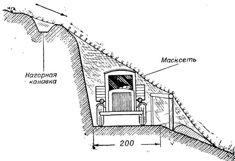
Рис. 157. Заслон для укрытия автотранспорта
