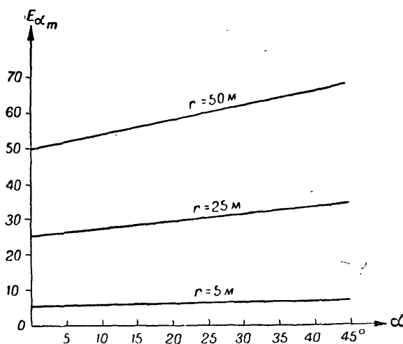
Рис. 133. График ошибок E_{\alpha m} в зависимости от величин угла \alpha при r = 5 \text{ м} , r = 25 \text{ м} и r = 50 \text{ м}
