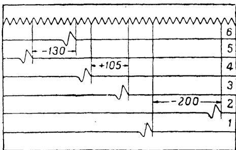
Рис. 72. Снятие отсчетов по зубцам записи камертона
