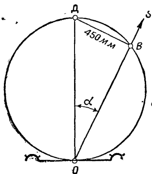
Рис. 89. Определение направления по \sin \alpha
