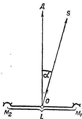
Рис. 38. Элементы акустической базы
