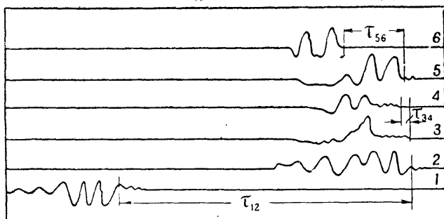
Рис. 79. У кривых первого, второго, третьего, четвертого и пятого перьев впереди выступают записи отраженных волн в виде мелких зубчиков
