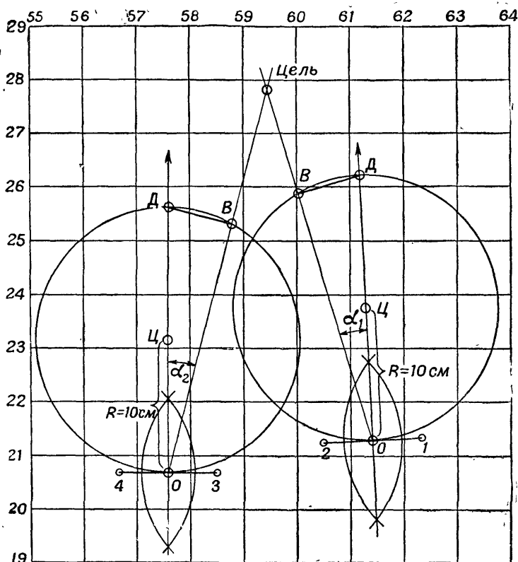
Рис. 91. Определение координат цели графическим способом
