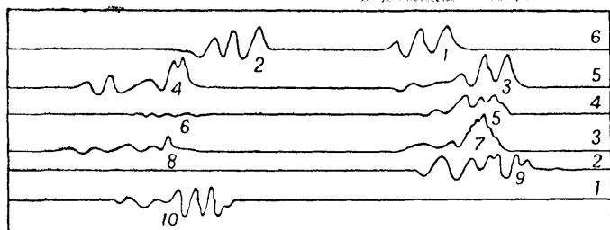
Рис. 80. На линиях второго, пятого и шестого перьев записи балистических волн, отмеченные цифрами 9, 1 и 3, легко можно принять за дульные
