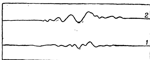
Рис. 34. Записи, полученные при отражении волн от местных предметов
