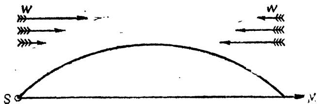
Рис. 31. Искривление звукового луча при попутном ветре, усиливающемся с высотой, и при встречном ветре, уменьшающемся с высотой
