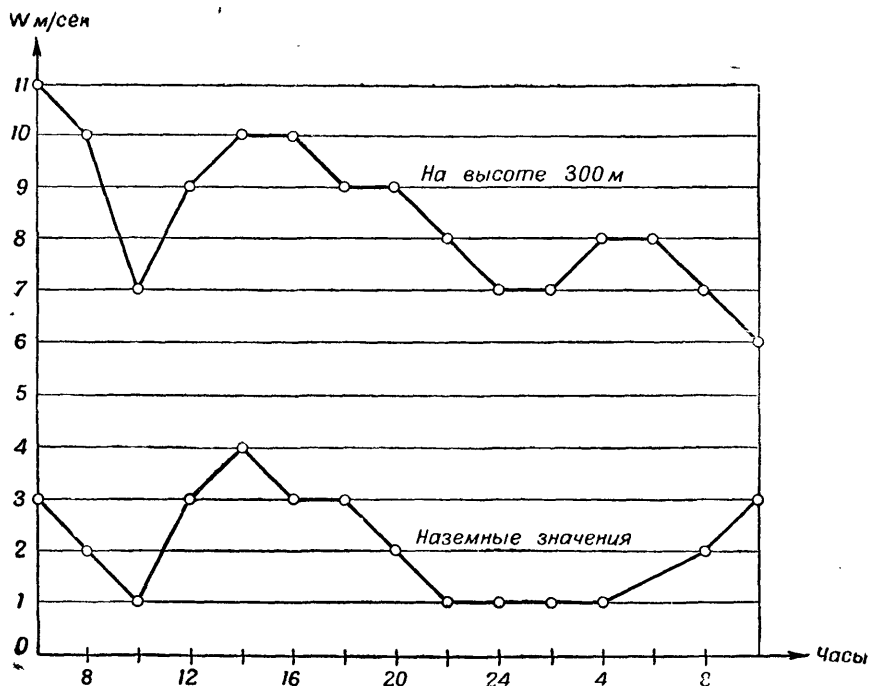
Рис. 129. Медленные изменения скорости наземного ветра и на высоте 300 м
