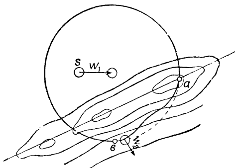
Рис. 23. Изменение фронта звуковой волны в связи с изменением скорости и направления ветра
