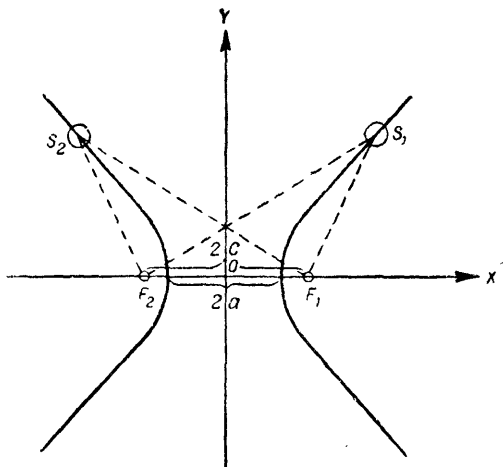
Рис. 43. Гипербола
