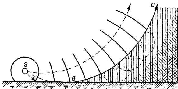
Рис. 28. Дифракция звука в области звуковой тени
