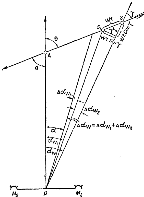
Рис. 49. Схема для вывода общей формулы поправки на ветер
