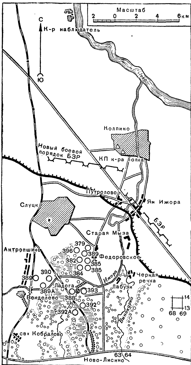
Рис. 144. Для засечки важных целей (392 и 392А) с целью уменьшения продольной слагающей встречного ветра боевой порядок БЗР переместили на север
