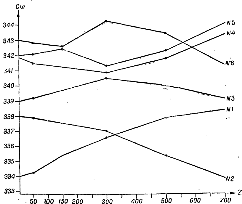
Рис. 33. Графики изменения скорости звука с высотой для определения благоприятных и неблагоприятных условий работы
