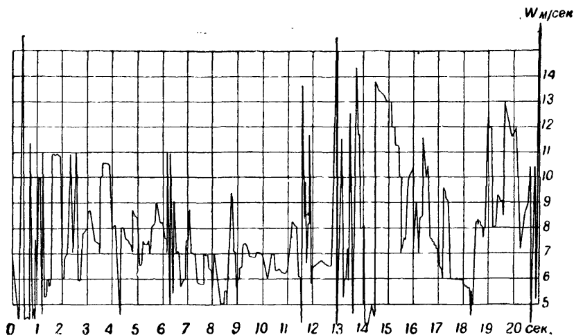
Рис. 128. Быстрые изменения скорости ветра
