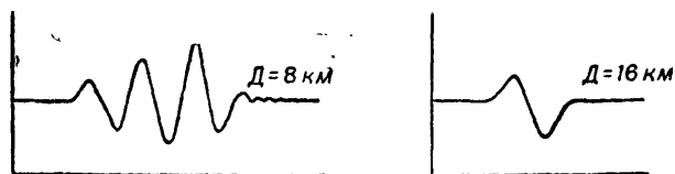
Рис. 36. Изменение характера записи дульной волны с увеличением расстояния от орудия
