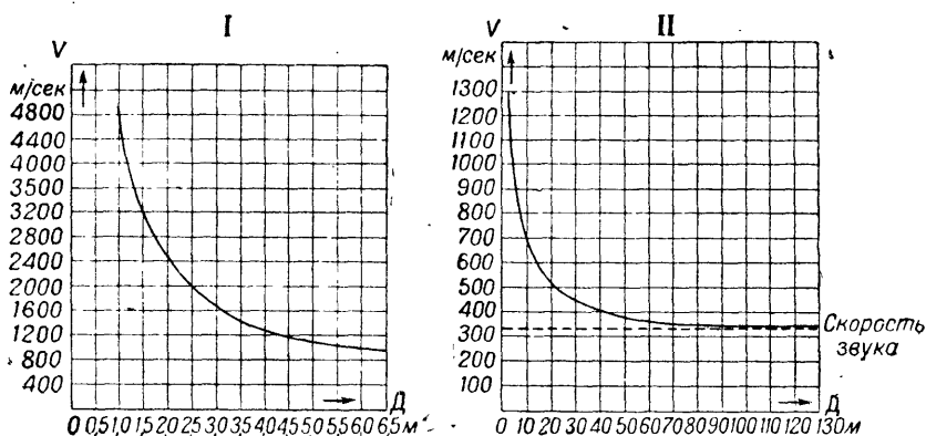
Рис. 12. Изменение скорости ударной волны в зависимости от расстояния
