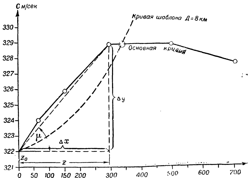
Рис. 51. График изменения скорости звука с высотой
