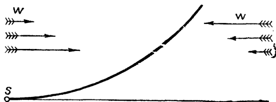
Рис. 32. Искривление звукового луча при попутном ветре, уменьшающемся с высотой, и при встречном ветре, усиливающемся с высотой
