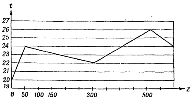
Рис. 127. Основная кривая скорости звука имеет два максимума
