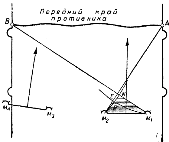
Рис. 145. Участок местности, на котором изменения метеорологических факторов сильно искажают отсчеты
