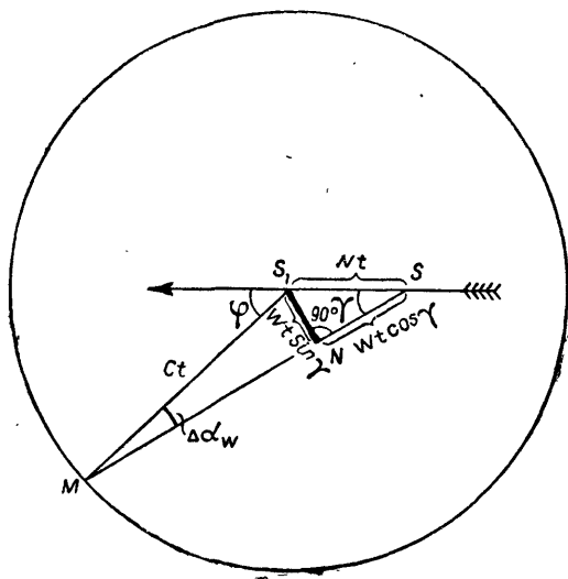
Рис. 10. Смещение центра акустической волны по направлению ветра
