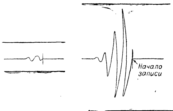
Рис. 1. Записи, полученные при стрельбе из одного орудия при разных метеорологических условиях
