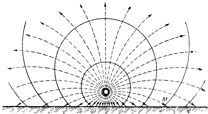
Рис. 29. Искривление звуковых лучей при повышении температуры с высотой
