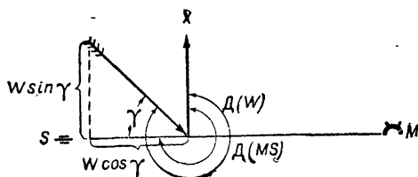
Рис. 11. Схема определения угла \gamma , продольная и боковая слагающие ветра
