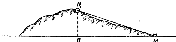
Рис. 57. Цель (точка C ) находится выше звукоприемника (точка M )
