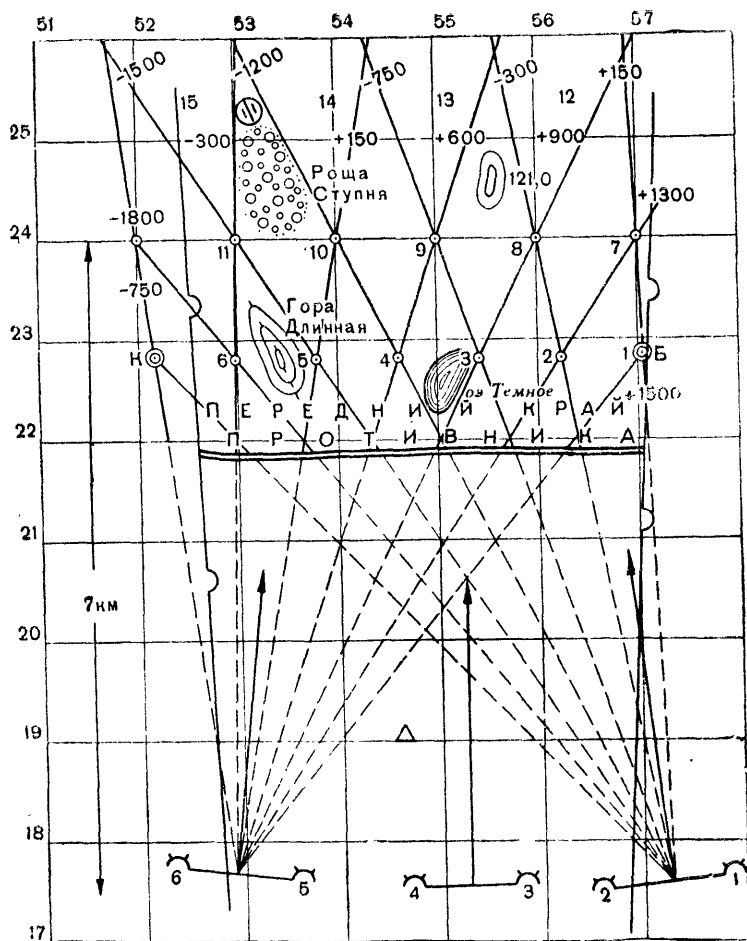
Рис. 124. Схема разведывательных участков с указанными величинами отсчетов с крайних баз
