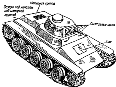
Рис. 10. Уязвимые места танка для поражения зажигательными бутылками.
