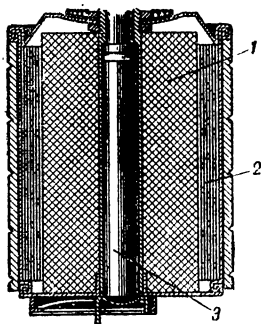
Рис. 4. Разрывной заряд
