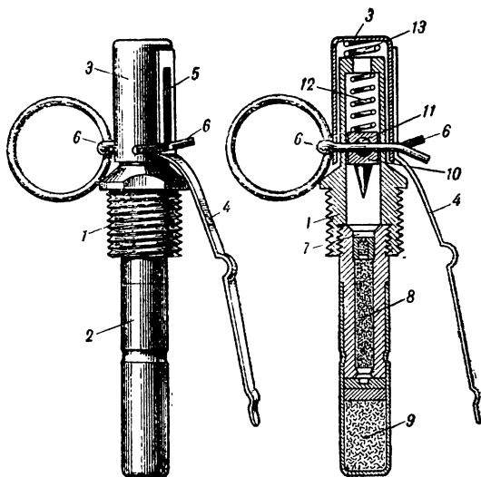
Рис. 28. Запал
