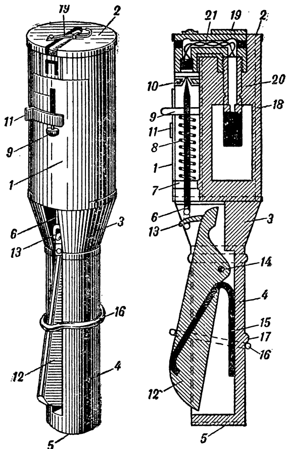
Рис. 20. Детали гранаты
