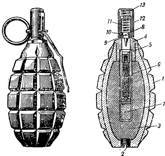
Рис. 26. Общий вид и части гранаты марки Ф-1
