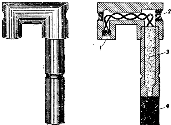
Рис. 22. Запал
