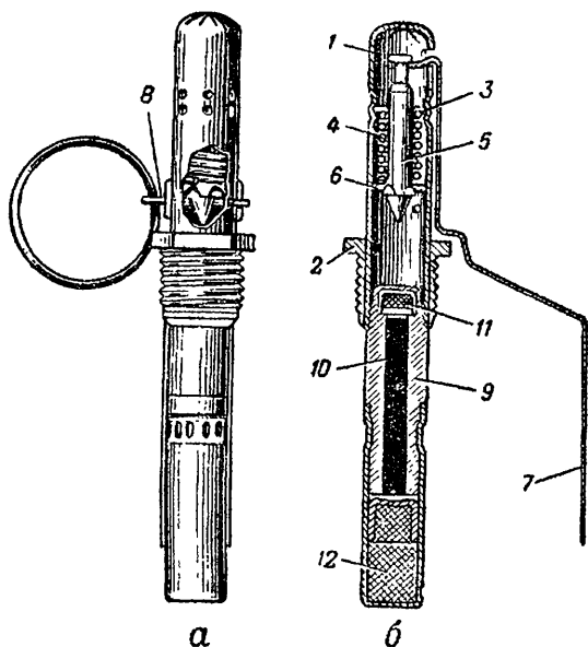
Рис. 4. Запал гранаты УЗРГМ:
