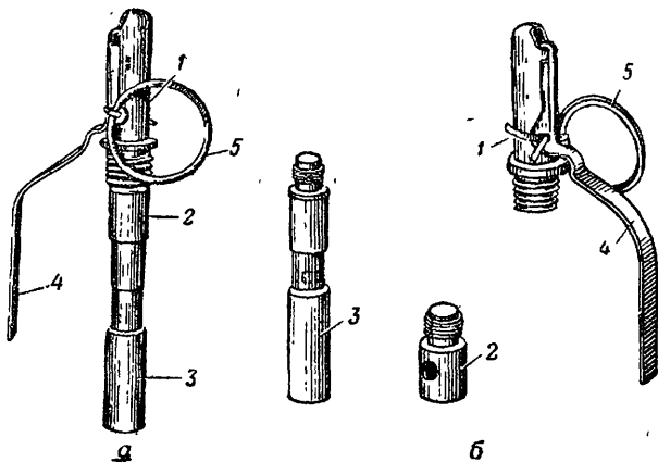
Рис. 2. Имитационный запал:
