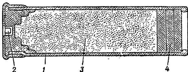
Рис. 7. Имитационный запал:
