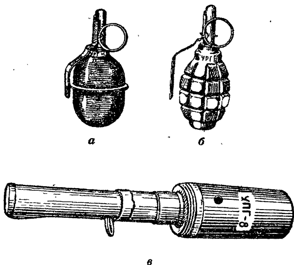
Рис. 1. Общий вид учебно-имитационных ручных гранат:
