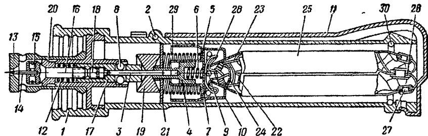
Рис. 6. Рукоятка (в разрезе):
