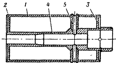
Рис. 5. Корпус гранаты (в разрезе): 1 — оболочка; 2 — дно; 3 — крышка; 4 — ствол; 5 — трубка и отверстие в ствол- лике
