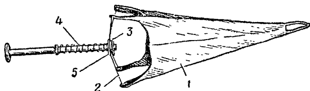
Рис. 14. Стабилизатор:
