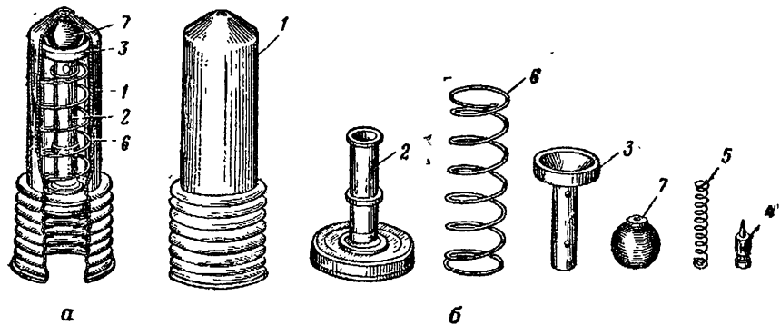
Рис. 13. Ударный механизм:
