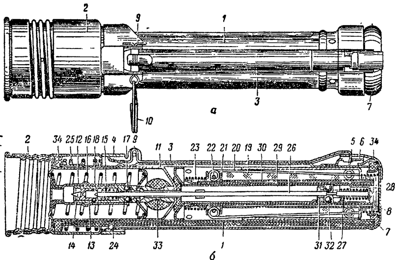
Рис. 12. Рукоятка:
