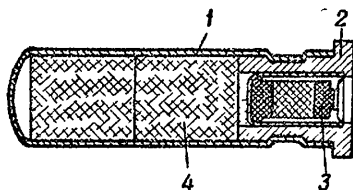
Рис. 15. Запал (в разрезе): 1 — гильза; 2 — втулка; 3 — капсюль-детонатор; 4 — дополнительный детонатор
