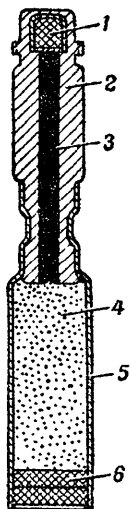
Рис. 3. Имитационная часть запала (в разрезе):
