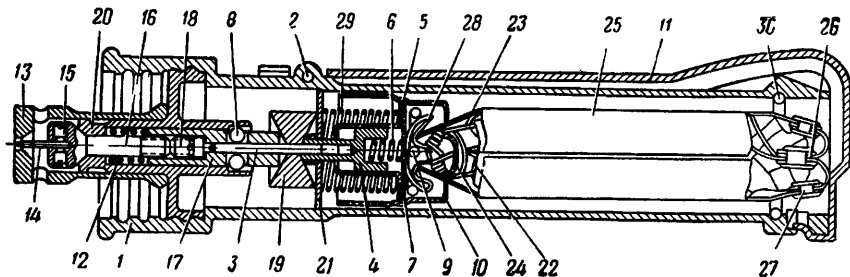
Рис. 6. Рукоятка (в разрезе):
