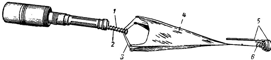
Рис. 17. Граната во время полета:
