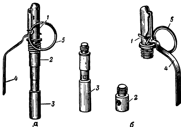
Рис. 2. Имитационный запал:
