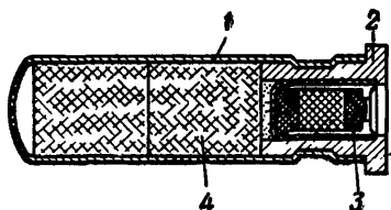
Рис. 15. Запал (в разрезе):
