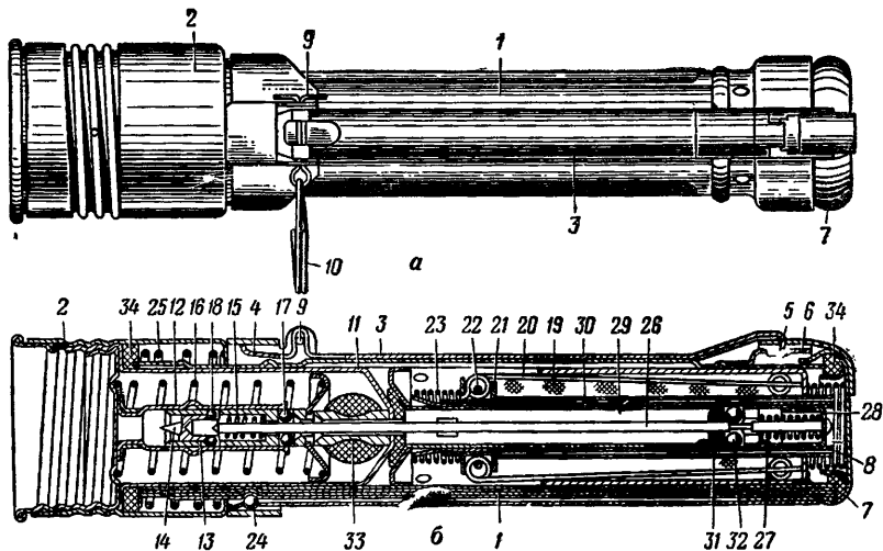
Рис. 12. Рукоятка:
