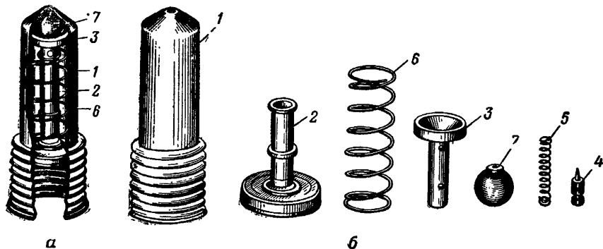
Рис. 13. Ударный механизм:
