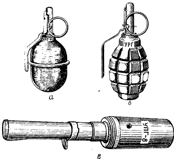
Рис. 31. Общий вид учебно-имитационных ручных гранат: а — УРГ-Н; б — УРГ; в — УПГ-8
