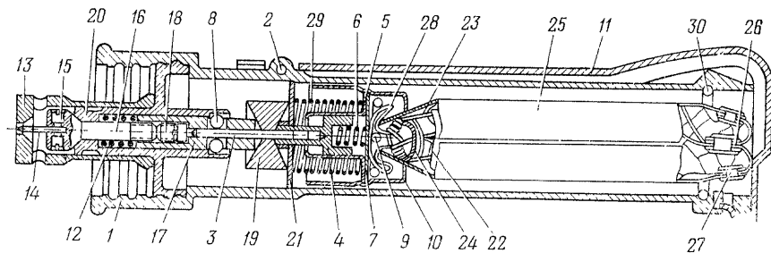
Рис. 36. Рукоятка (в разрезе):
