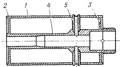
Рис. 35. Корпус гранаты (в разрезе): 1 — оболочка; 2 — дно; 3 — крышка; 4 — ствол; 5 — трубка и отверстие в стволике
