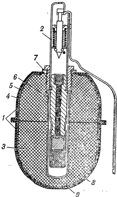
Рис. 3. Устройство ручной осколочной гранаты РГД-5:
