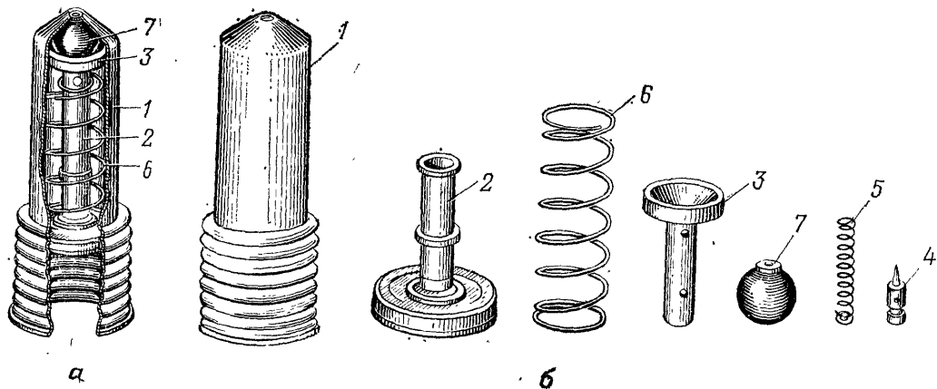
Рис. 13. Ударный механизм:
