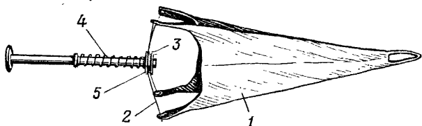
Рис. 14. Стабилизатор:
