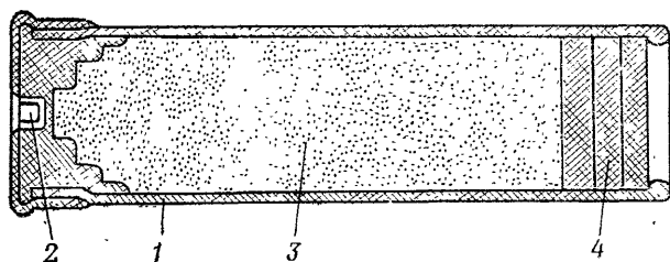
Рис. 37. Имитационный запал:
