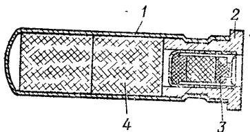
Рис. 15. Запал (в разрезе):
