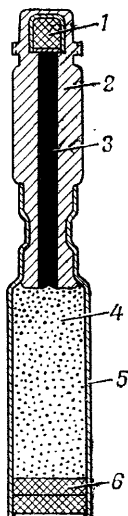
Рис. 33. Имитационная часть запала (в разрезе):
