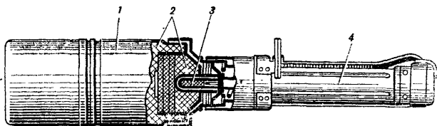
Рис. 10. Устройство ручной противотанковой кумулятивной гранаты РКГ-3:
