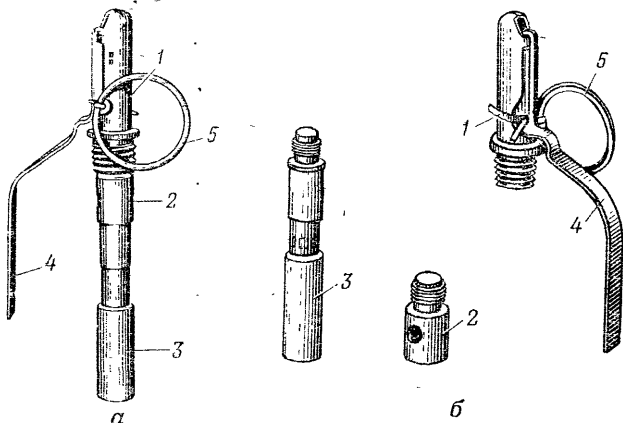
Рис. 32. Имитационный запал:
