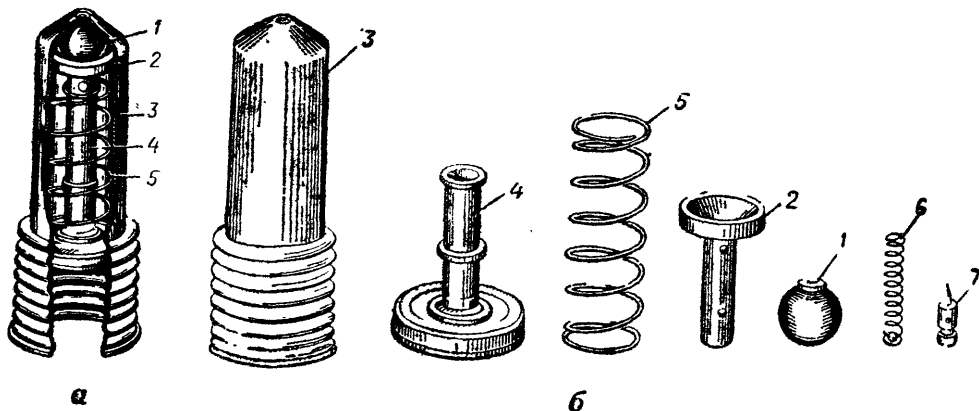
Рис. 17. Ударный механизм:
