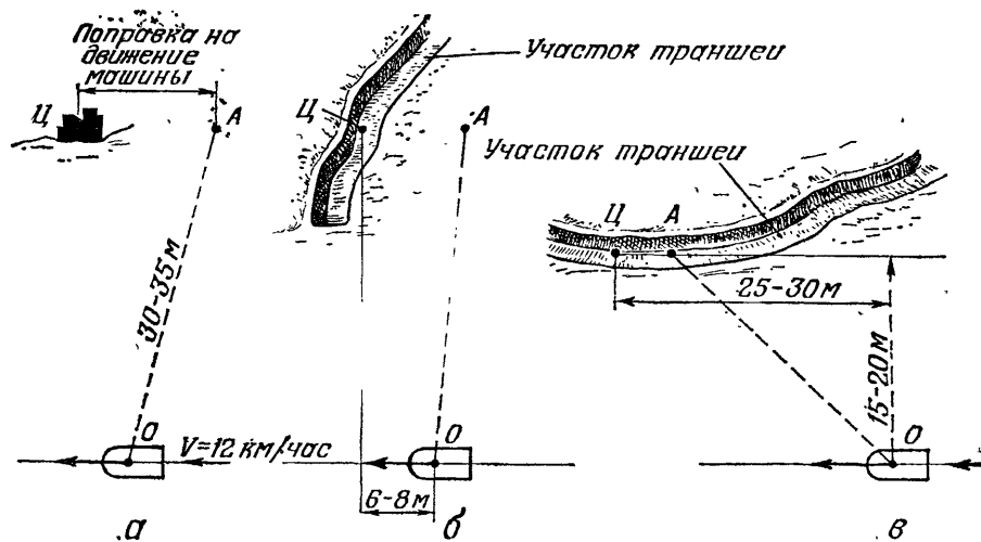
Рис. 30. Выбор направления и момента броска гранаты из движущегося бронетранспортера:
