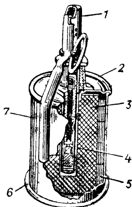
Рис. 8. Устройство ручной осколочной гранаты РГ-42:
