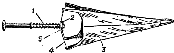
Рис. 18. Стабилизатор:
