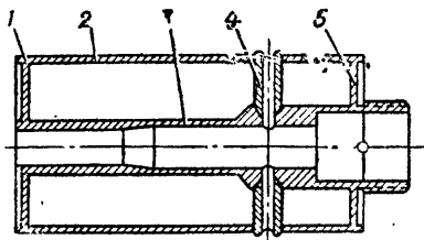
Рис. 39. Корпус гранаты (в разрезе): 1—дно; 2—оболочка; 3—ствол; 4—трубка и отверстие в стволке; 5 — крышка
