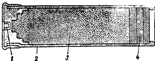
Рис. 41. Имитационный запал:
