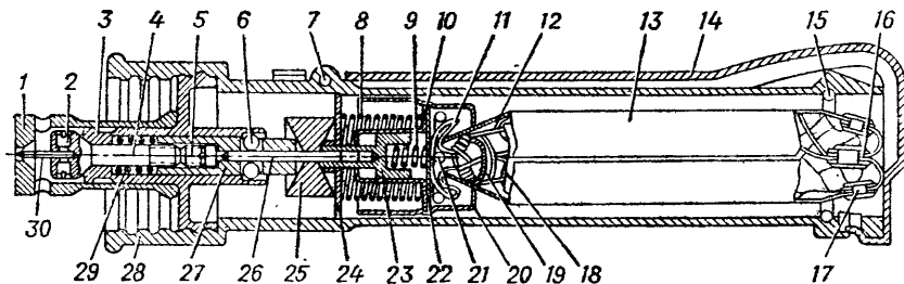
Рис. 40. Рукоятка (в разрезе):
