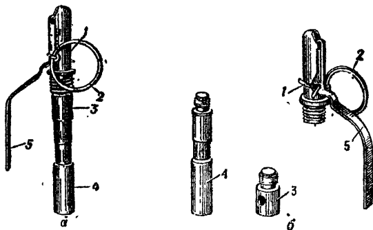
Рис. 36. Имитационный запал:
