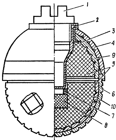
Рис. 12. Устройство ручной гранаты РГО без запала:
