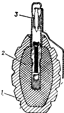
Рис. 13. Устройство ручной осколочной гранаты Ф-1.
