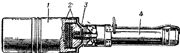
Рис. 14. Устройство ручной противотанковой кумулятивной гранаты РКГ-3:
