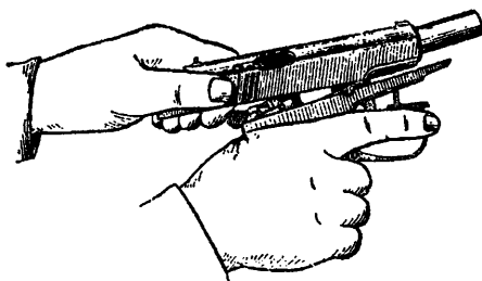
Рис. 6. Отделение затвора от рамки
