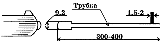
Рис. 79. Алюминиевая трубка с мушкой
