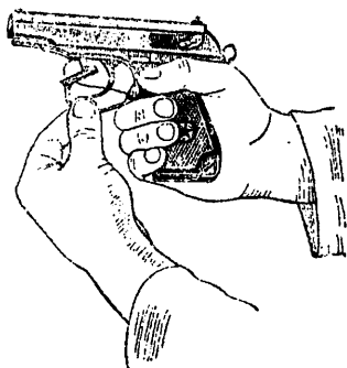
Рис. 5. Оттягивание спусковой скобы
