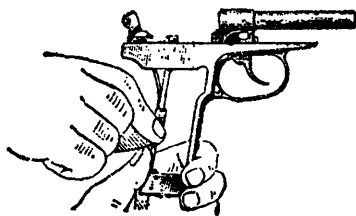
Рис. 26. Закрепление боевой пружины задвижкой
