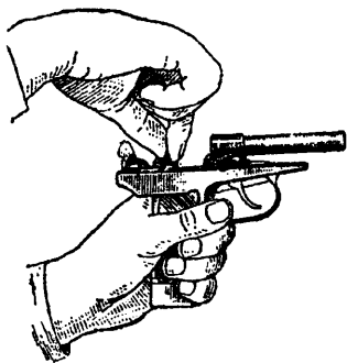
Рис. 27. Присоединение затворной задержки и шептала к рамке
