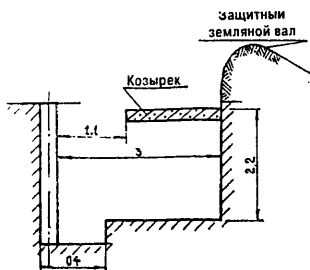
Рис. 112. Заглубленный блиндаж
