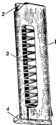
Рис. 42. Магазин:
