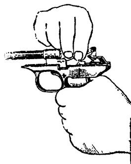
Рис. 17. Отделение спусковой тяги с рычагом взвода от рамки
