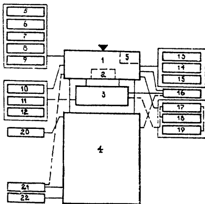
Рис. 107. Схема взаимосвязей вспомогательных помещений между собой и с основными помещениями и сооружениями отдельно стоящих закрытого и полукрытого тиров:
