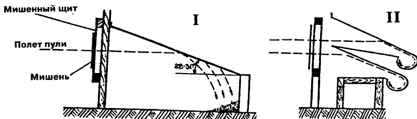
Рис. 111. Схемы устройства пулеулавливателей: I - в виде наклонной металлической плоскости; II - в форме улитки
