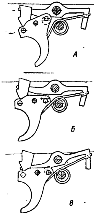
Рис. 24. Схема положения частей спускового механизма в различные периоды:
