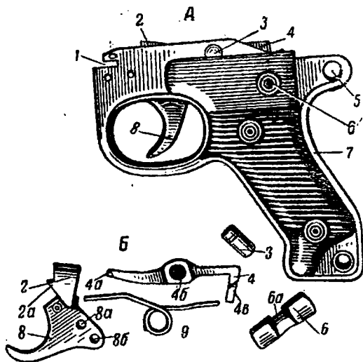
Рис. 8. Спусковой и предохранительный механизмы:
