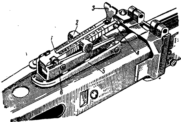
Рис. 10. Прицел:
