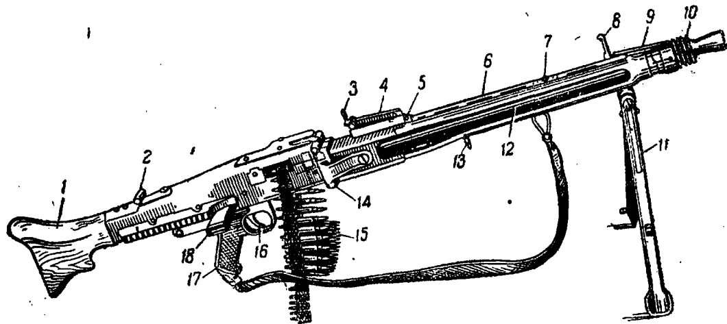
Рис. 1. Общий вид германского 7,92-мм пулемёта обр. 1942 г. MG-42:
