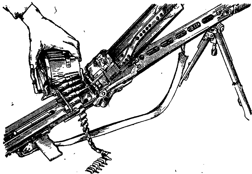
Рис. 18. Как примыкать барабан
