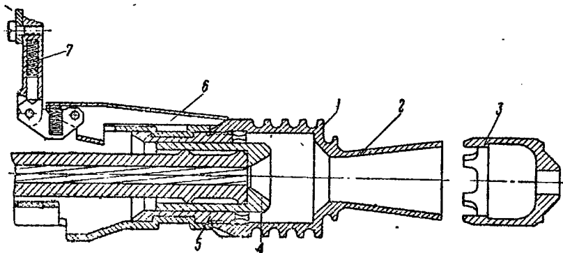
Рис. 3. Надульник:
