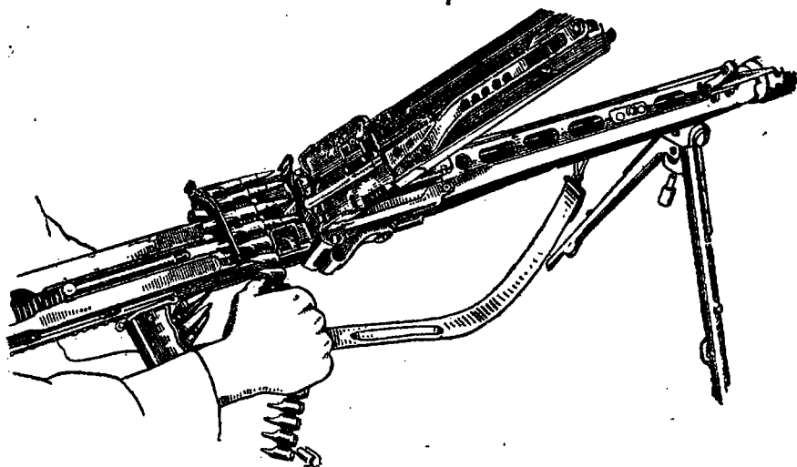
Рис. 17. Как зарядить пулемёт при питании из ленты
