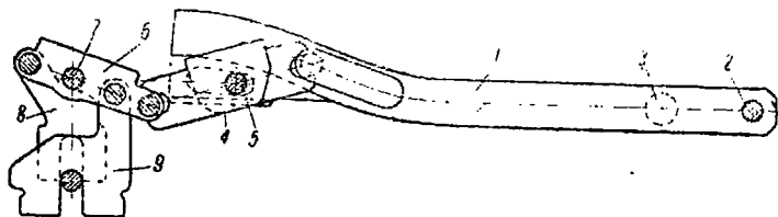
Рис. 22. Схема подающего механизма (вид сверху):
