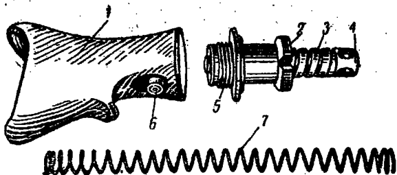
Рис. 9. Затыльник:
