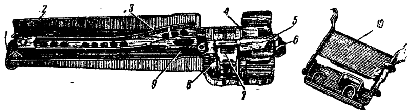
Рис. 7. Крышка короба с подающим механизмом:
