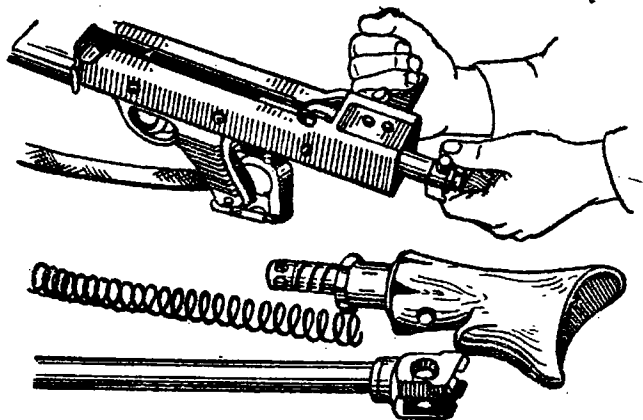
Рис. 13. Как отделить затвор
