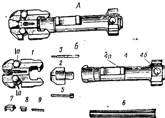
Рис. 6. Затвор (вид снизу):
