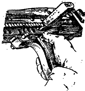
Рис. 16. Как поставить затвор на предохранитель
