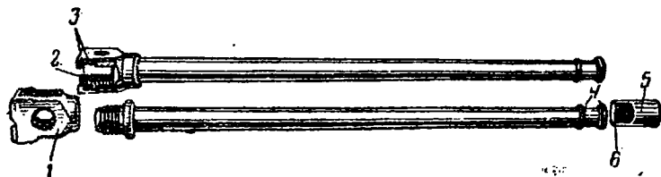
Рис. 2. Ствол:
