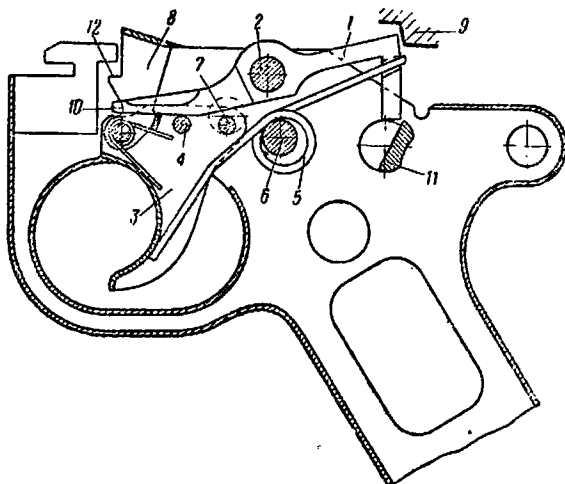
Рис. 23. Схема положения частей спускового механизма при затворе, находящемся на боевом взводе:
