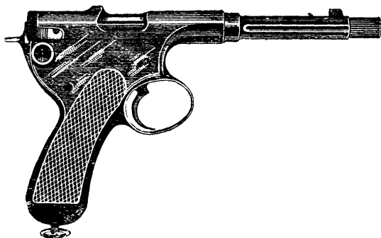
Р и с. 23. Пистолет военного образца сист. Глизенти 1909 г. (Италия), кал. 7,65 мм.
