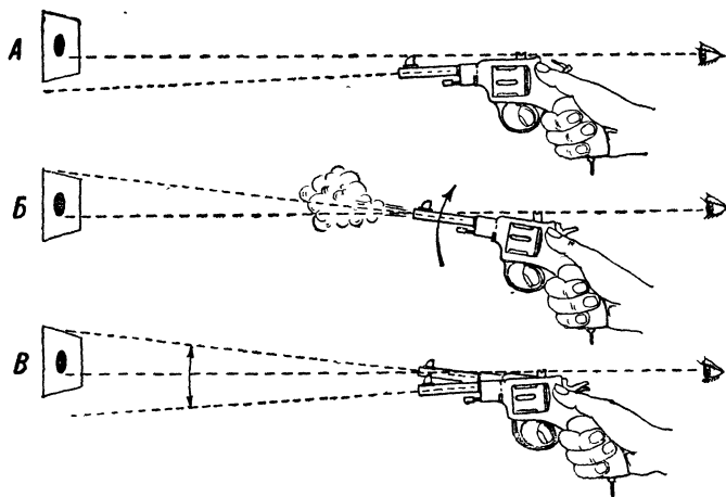
Р и с. 75. Схема образования углов прицеливания, бросания и вылета при стрельбе из личного портативного оружия:
