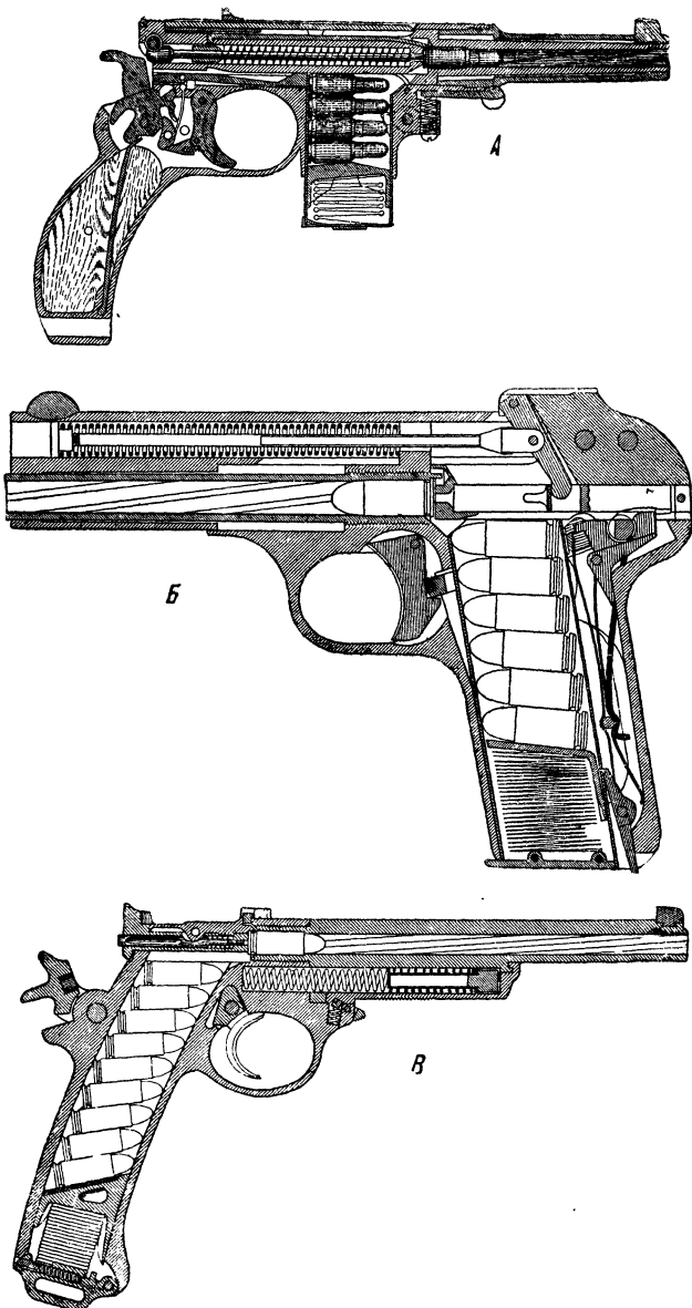
Рис. 16. Схематический разрез, самозарядных пистолетов разных систем:
