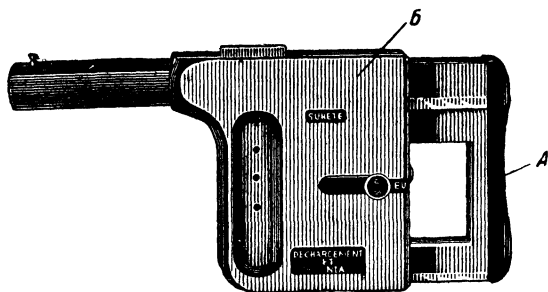
Рис. 41а. Оригинальный неавтоматический пятизарядный пистолет сист. Галюа. Галюа. Чтобы произвести из него выстрел, нужно, захватив пистолет кистью руки, вжимать подвижную раму (А) в корпус пистолета (В).
