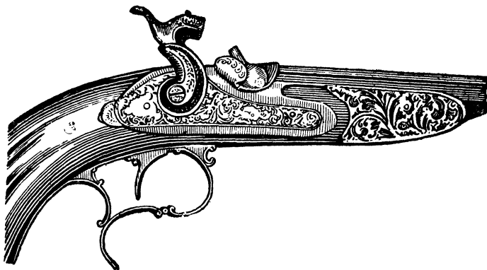
Р и с. 13. Ударно-капсюльный замок целевого пистолета XIX в.
