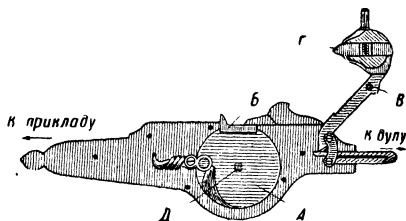
Рис. 7. Немецкий колесцовый замок первой половины XVI в.
