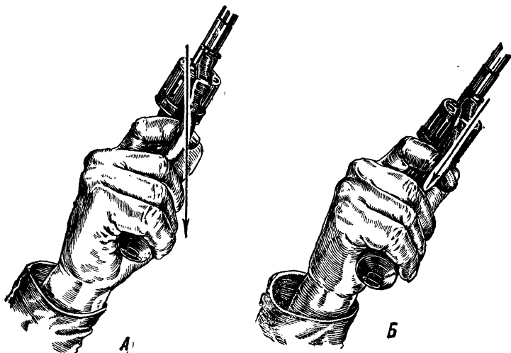
Р и с. 79. Направление силы при нажиме на спусковой крючок: А — неправильное направление (под углом к плоскости стрельбы); Б — правильное направление.
