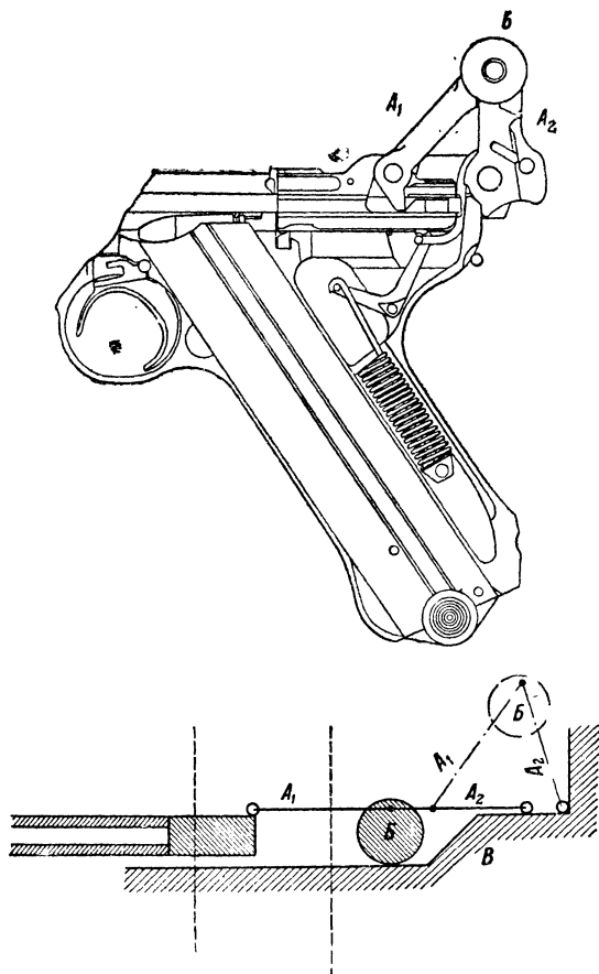
Рис. 20. Схема запирающего механизма пистолета „Парабеллум“.
