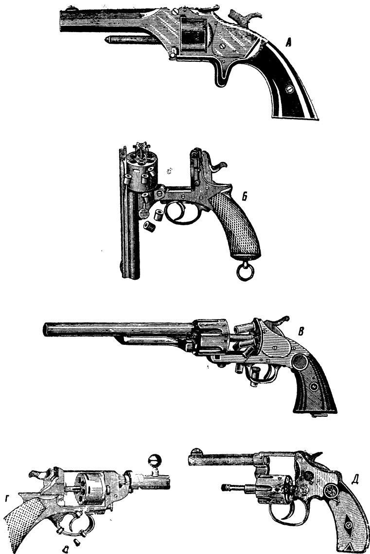
Р и с. 15а. Различные системы откидных стволов и барабанов револьверов:
