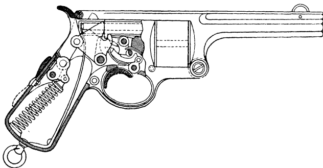
Р и с. 38. Автоматический револювер военного образца сист. Коломбо-Риччи (Италия) в разрезе.
