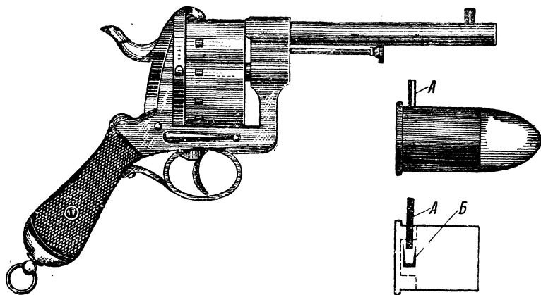
Рис. 15. Револьвер, патрон и гильза (в разрезе) сист. Лефаше обр. 1846 г.:
