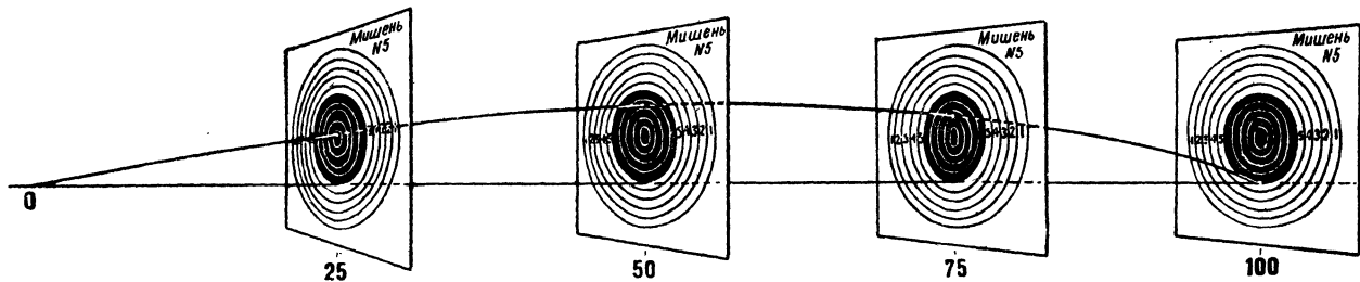
Р и с. 118. Траектория пули револьвера Наган обр. 1895 г., кал. 7,62 м.м., пристрелянного для 25 м по мишени № 5
