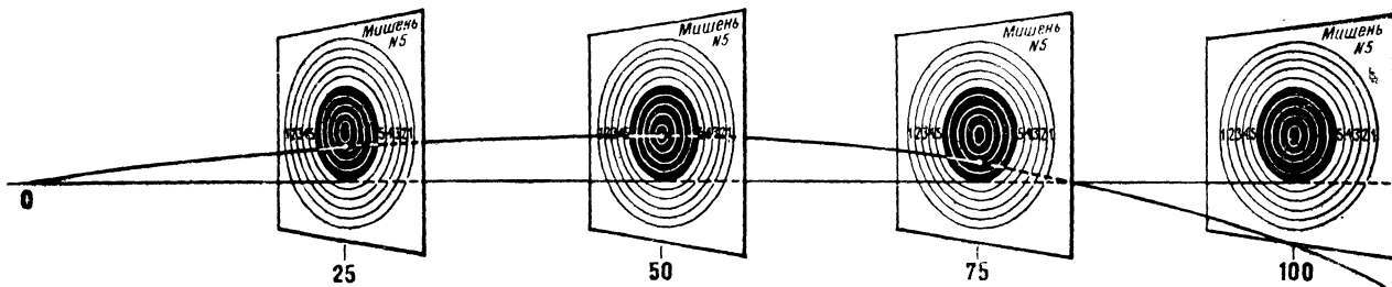
Р и с. 119. Траектория пули револьвера сист. Наган обр. 1895 г., кал. 7,62 м.м., пристрелянного для 50 м по мишени № 5,
