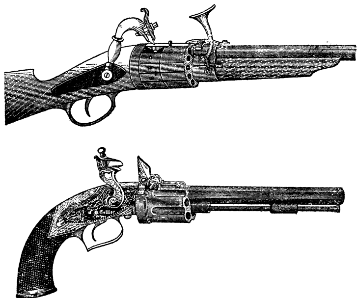
Рис. 11. Кремневые барабанные системы оружия: наверху — ружье первой половины XVII в.; внизу — револьвер мастера Коллиера в Англии (1810 г.).
