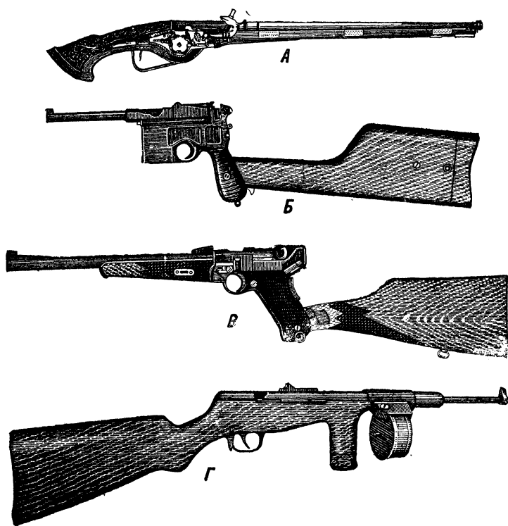
Р и с. 1. Разные пистолеты:
