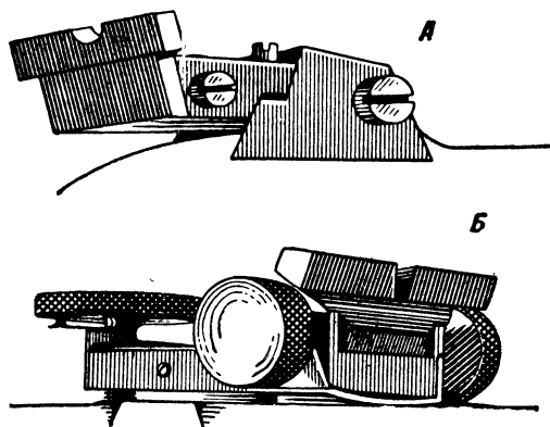
Р и с. 43. Прицельные приспособления (прицелы) целевых спортивных пистолетов:
