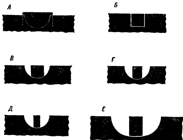
Р и с. 71. Соотношение поперечника мушки и ширины прорези:
