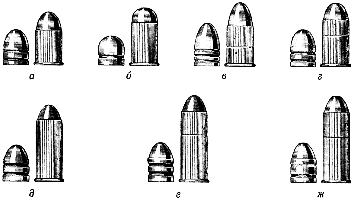
Р и с. 47е. Образцы патронов в натуральную величину. Патроны центрального огня для револьверов: а — различных английских (Булльдог, Скотт и др.), кал. 11,42 мм (450-го калибра); б — Веблей, кал. 11,43 мм (450-го калибра); в — Веблей, армейская модель (II образца), кал. 11,5 мм (450-го калибра); г — автоматических (45 230) английских, кал. 11,5 мм (455-го калибра); д — Смит-Вессона, кал. 11,43 мм (5-го калибра); е — Кольта, кал. 11,43 мм (45-го калибра); ж — казенного образца 1909 г. (США), кал. 11,43 мм (45-го калибра).
