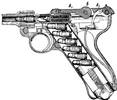
Р и с. 19. Продольный вертикальный разрез пистолета „Парабеллюм“ обр. 1900 г.
