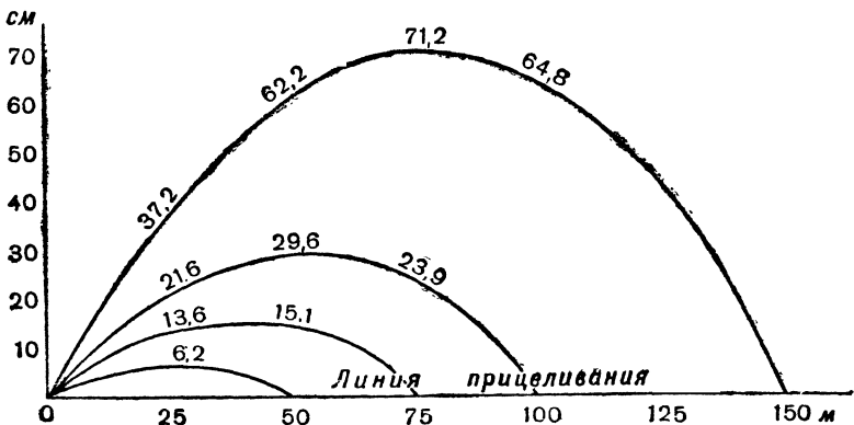
Р и с. 117. Траектория пули малокалиберного („Long Bifle 22“) пистолета.
