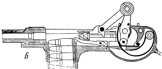
Р и с. 17. Пистолет сист. Борхардта:
