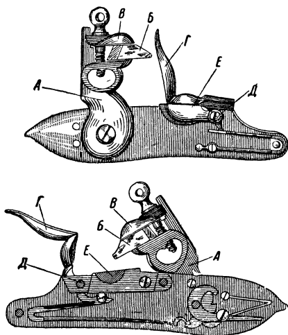
Рис. 9. Ударный кремневый замок позднейшего времени для военных ружей и пистолетов: наверху — наружный вид (курок взведен, полка накрыта крышкой-огнивом); внизу — вид с внутренней стороны (виден механизм; курок спущен, крышка-огниво откинута).
