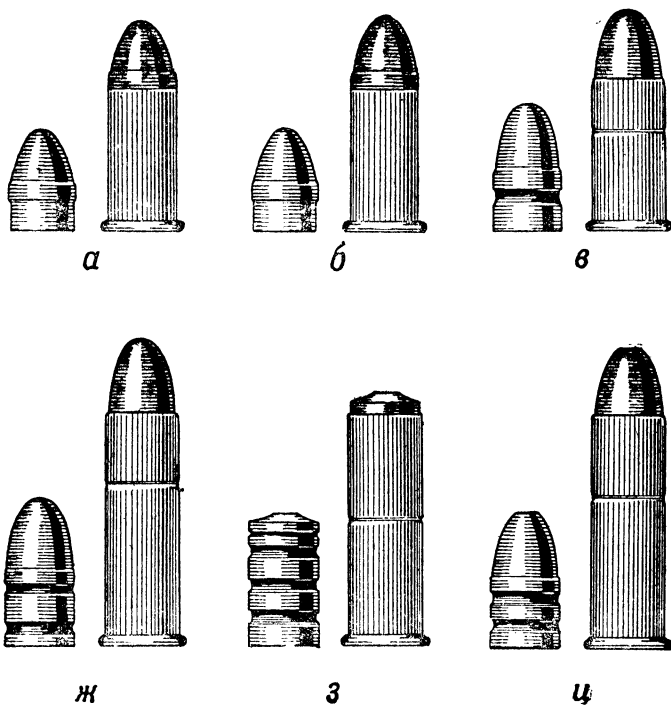
Рис. 47г. Образцы патронов в натуральную величину а — Кольта (короткий патрон), кал. 9 мм (38-го калибра); б — Кольта полицейского образца, кал. 9 мм (380-го калибра); в — Кольта полицейского образца, кал. 9 мм (38-го калибра); ж — Смит-Вессона „специальный“ (усиленный патрон), средних дистанций“, кал. 9 мм (38-го калибра); з — Кольта „спе- циальный полицейский“ (последний образец); и — Кольта „спе- циальный полицейский“ (последний образец); к — Кольта, так называемый „38-40“, кал. 9 мм (8-го калибра); л — Кольта (бойный патрон), кал.
