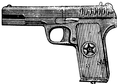
Р и с. 33. Пистолет военного образца сист. Токарева („ТТ“) 1933 г. (СССР), кал. 7,62 мм.
