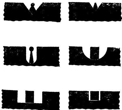
Р и с. 70. Прицельные приспособления револьверов и пистолетов (основные типы).
