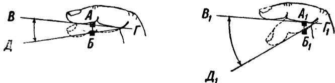
Рис. 78. Преимущество спуска курка первой фалангой: движение пальца получается меньше.
