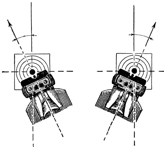
Р и с. 76. Сваливание оружия.
