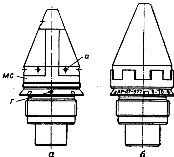
Рис. 3. Внешний вид радиовзрывателя AP-27: а — без герметизирующего колпака; б — с герметизирующим колпаком; МС — металлизированный слой; Г — гнезда под ключ; а — отверстия для выхода воздуха
