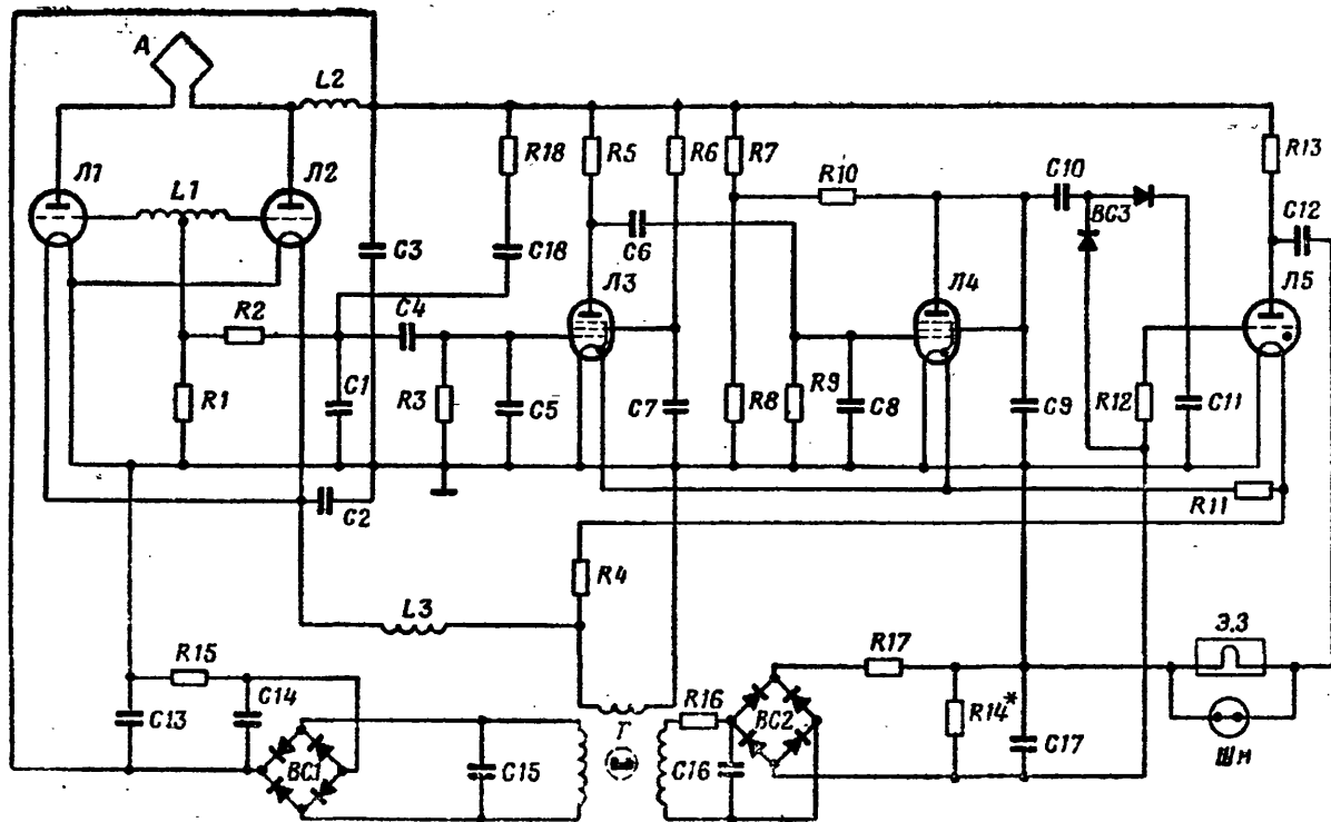
Рис. 4. Принциальная электрическая схема радновзрывателя AP-27
