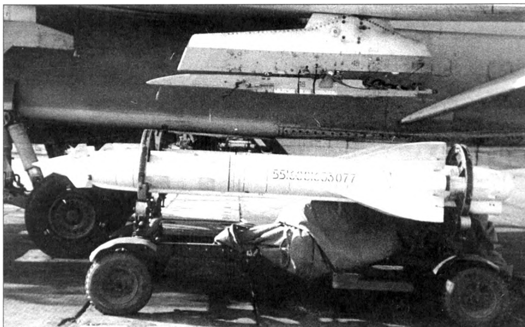
В качестве носителя Су-24 мог нести до четырех ракет X-23М
