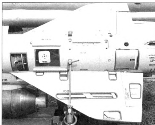
«Препарированная» ракета Х-59МЭ
