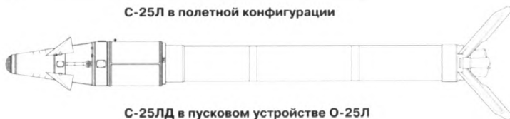
С-25ЛД в пусковом устройстве О-25Л
