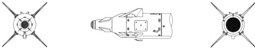
Х-29Л на авиационном катапультном устройстве АКУ-58-1
