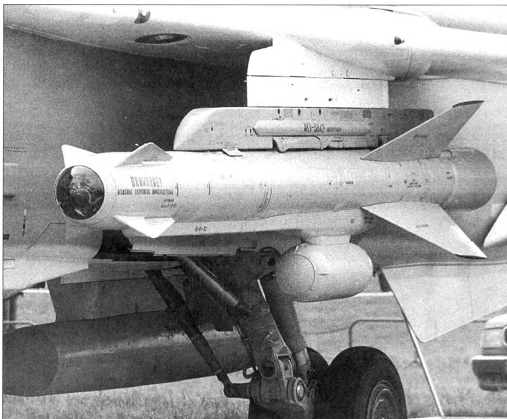
Х-59М на катапультном устройстве АКУ-58АЭ бомбардировщика Су-24М2
