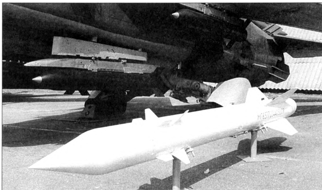
Масштабный макет X-27PC
