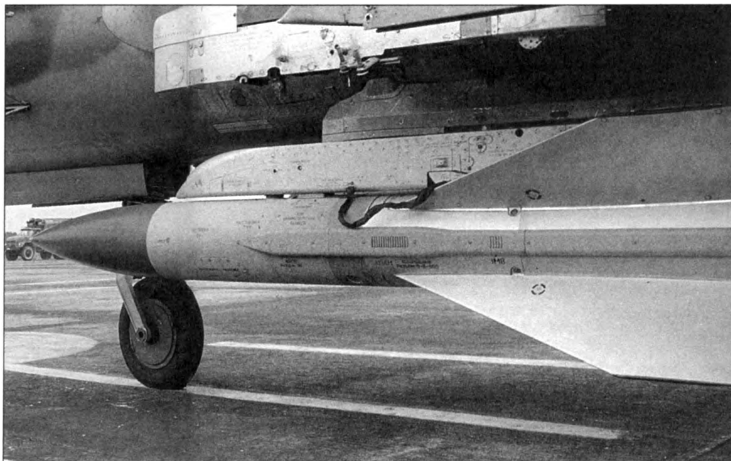
Х-58У на АКУ-58-1 под фюзеляжем Су-17М4
